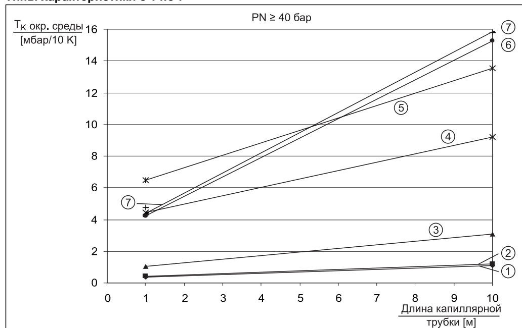
График зависимости T_{\text{к окр. среды}} от длины капиллярной трубки для PMP55, PN ≥ 40 бар
