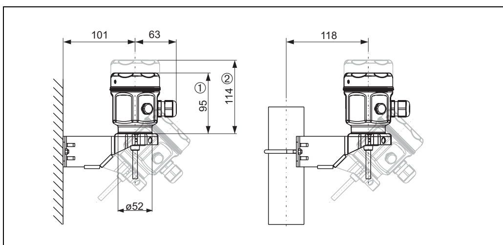
Размеры корпуса F15 Вес корпуса → стр. 55. 1) Крышка без смотрового стекла. 2) Крышка со смотровым стеклом.
