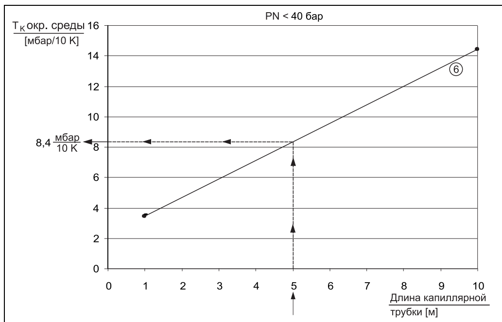
График зависимости коэффициента T_K окр. среды от длины капиллярной трубки для PMP55, PN < 40 бар
