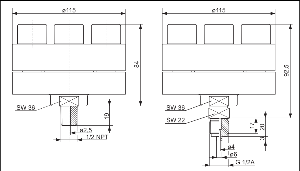
Присоединение к процессу PMP55, резьбовое исполнение UBJ" и UCJ, с встроенной уплотняющей кромкой, материал AISI 316L
