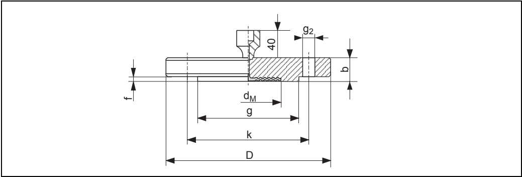
Присоединение к процессу PMP55, фланец JIS с выступом, материал AISI 316L
