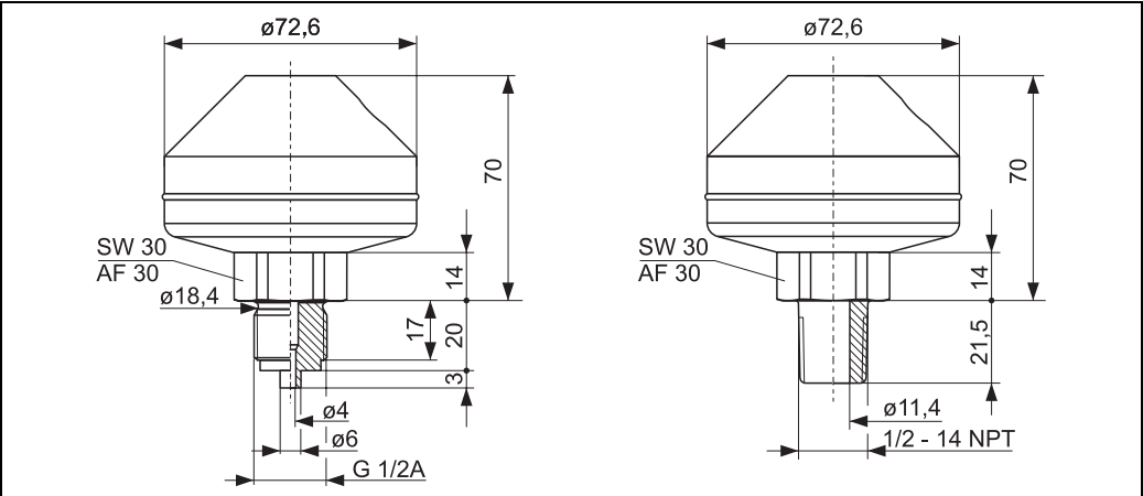
Присоединение к процессу PMP55, сварное исполнение UBJ и UCJ, материал AISI 316L
