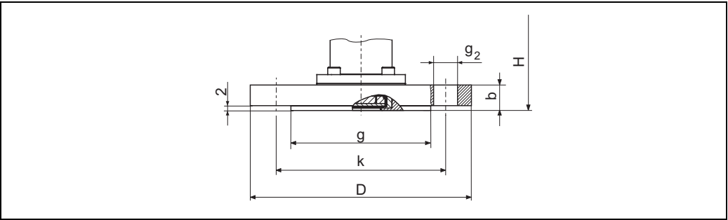
Присоединение к процессу PMC51, фланец JIS с выступом (мембрана «заподлицо»), материал AISI 316L. Для получения информации о высоте H см. таблицу ниже.
