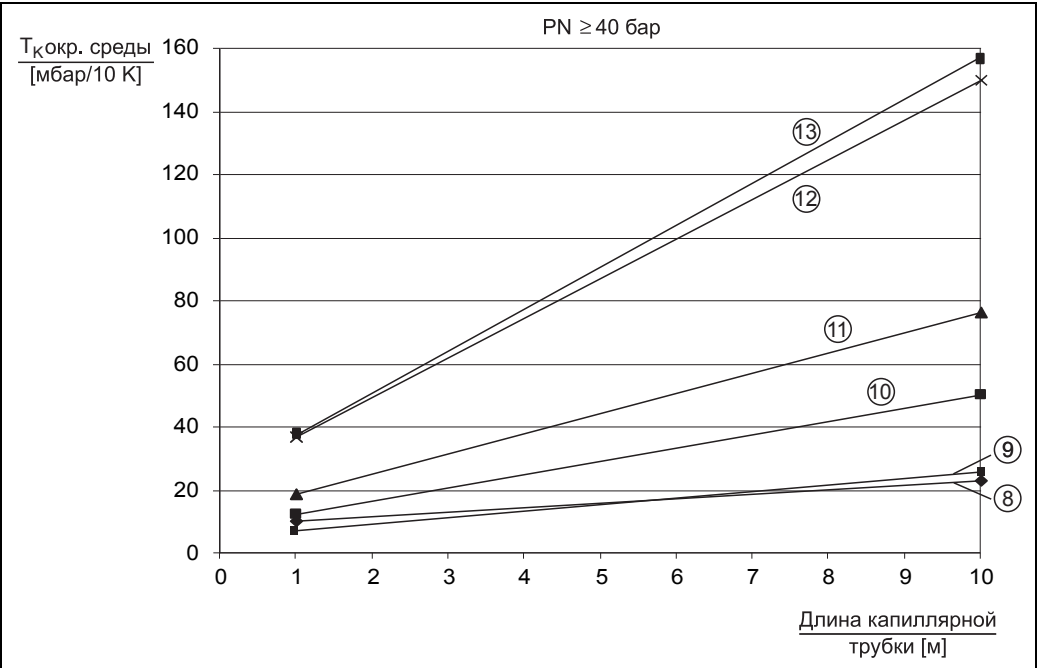
График зависимости T_K окр. среды от длины капиллярной трубки для PMP55, PN \geq 40 бар
