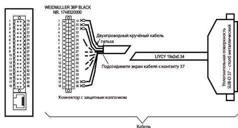
Схема кабельных соединений
