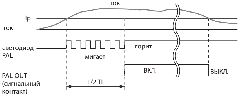
Диаграмма предварительной сигнализации
