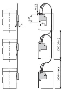
Вертикальный монтаж
