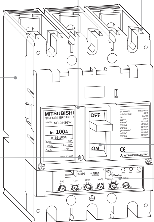
Конструкция выключателя типа NF125-SGW
