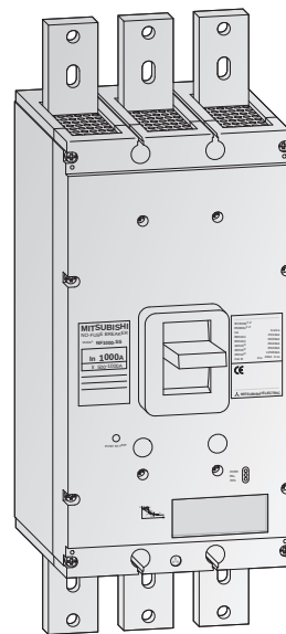
NF1000-SEW, 3-полюсный
