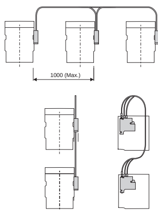
Горизонтальный монтаж
