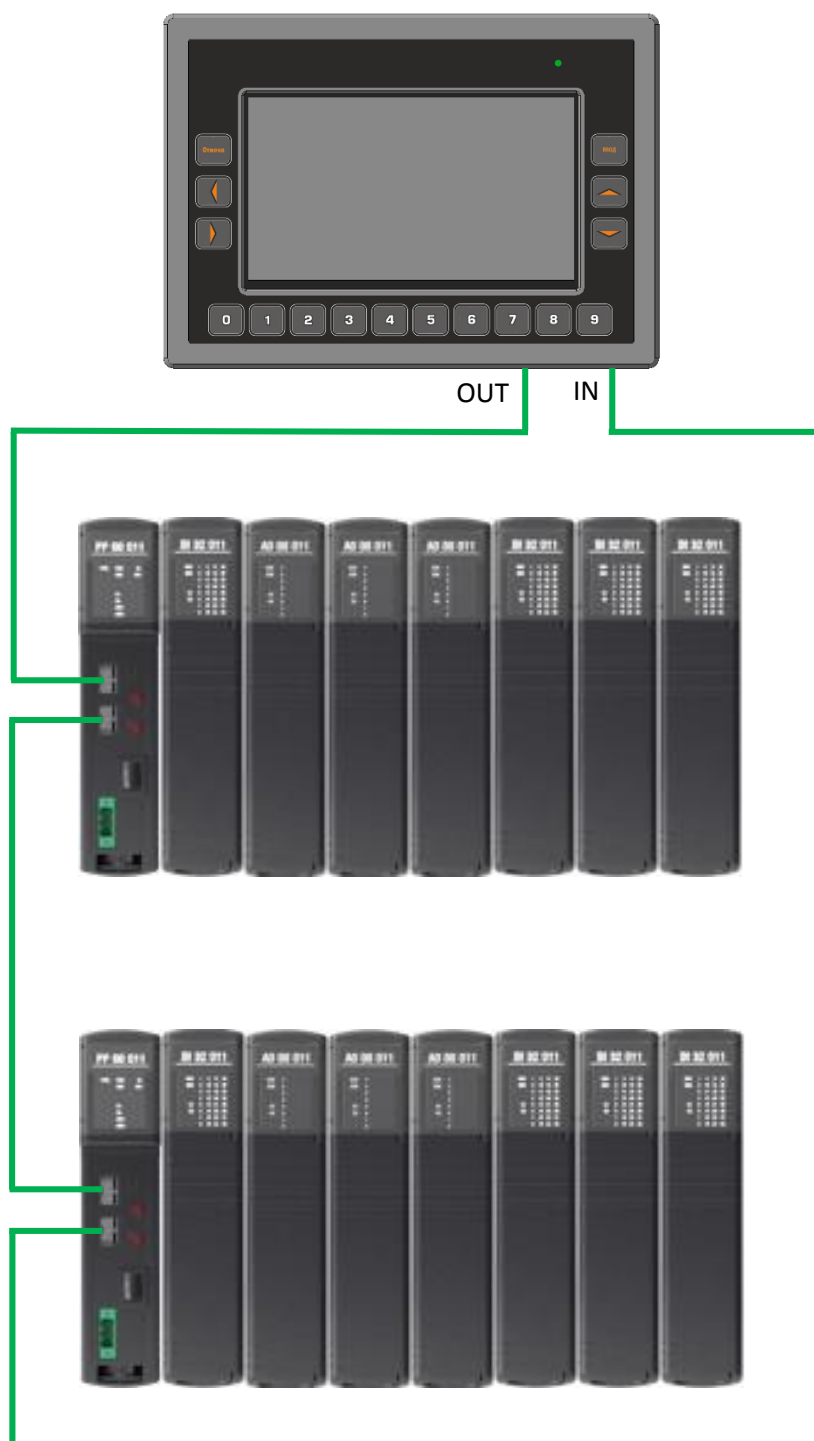
Рисунок 8 - Схема соединения крейтов «кольцо»
