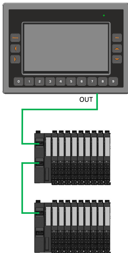
Рисунок 7 - Схема соединения крейтов «звезда»
