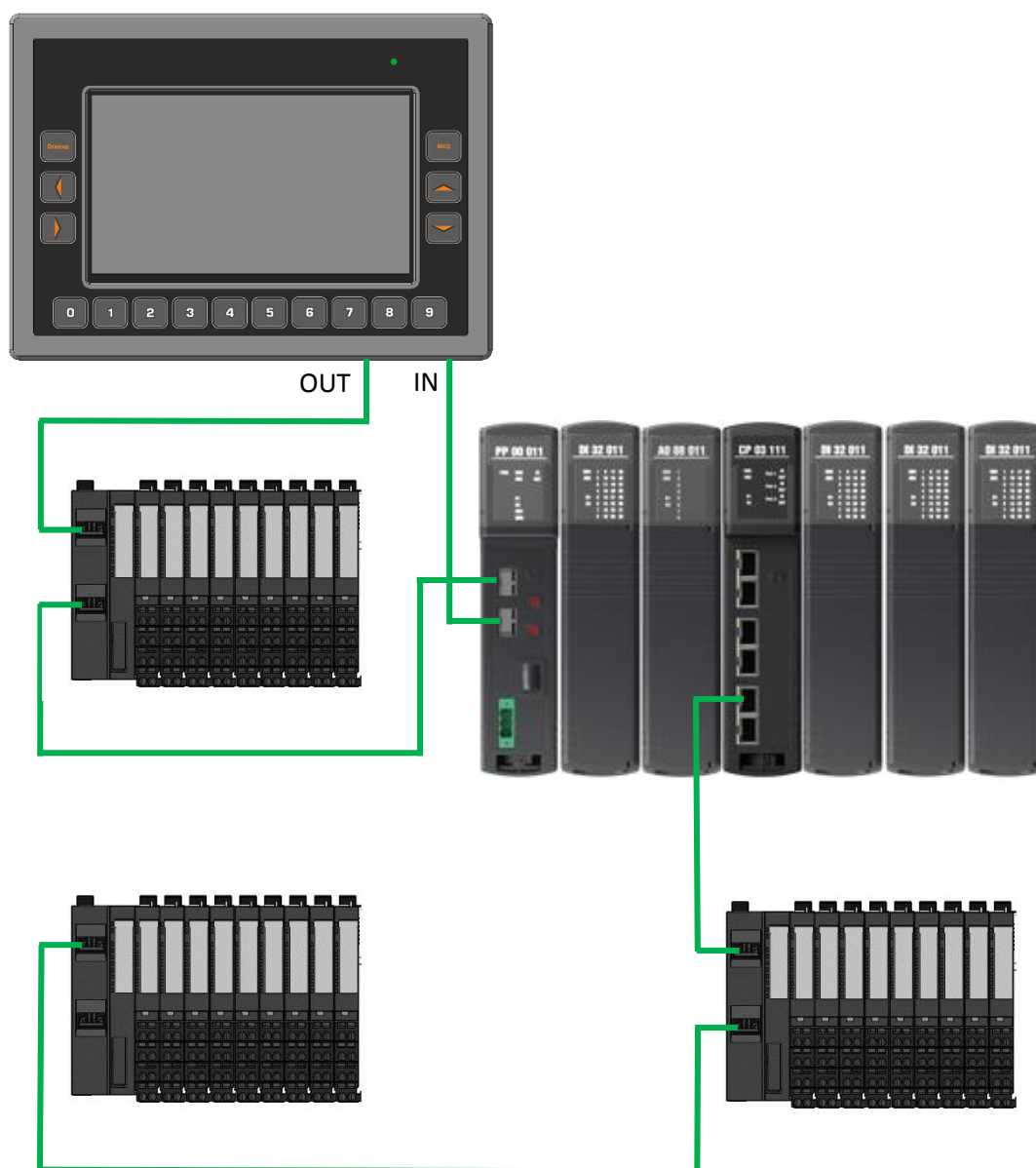
Рисунок 9 - Смешанная схема соединения крейтов
