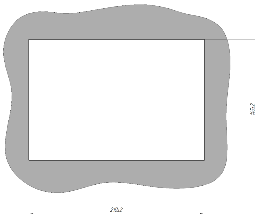
Рисунок 1 – Вырез в панели для установки контроллера
