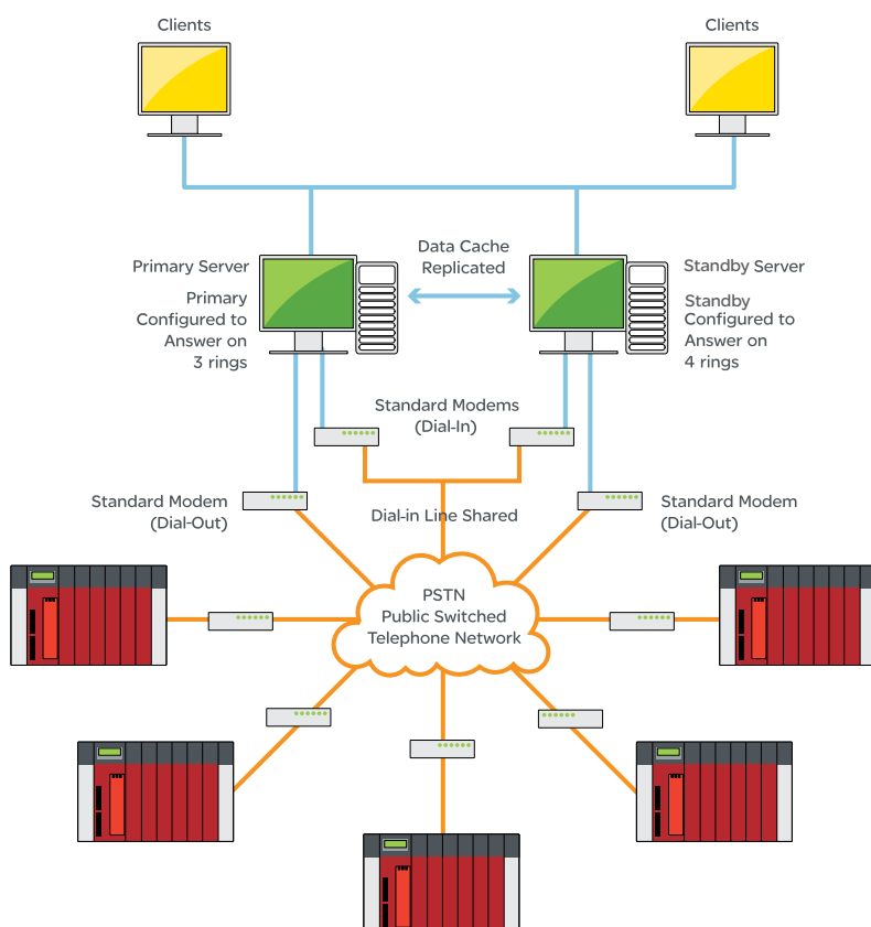
Пример архитектуры мониторинга удаленных устройств ввода-вывода с поддержкой резервирования входящих и исходящих вызовов на установление соединения
