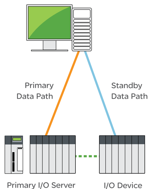
Резервирование устройств ввода-вывода
