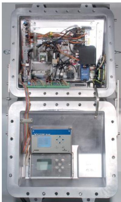
Вид изнутри: один модуль NDIR, один модуль NDUV, одна парамагнитная ячейка O 2 , термореле (без крышки), аналоговые выходы и выходы реле, цифровые входы и последовательный интерфейс.
