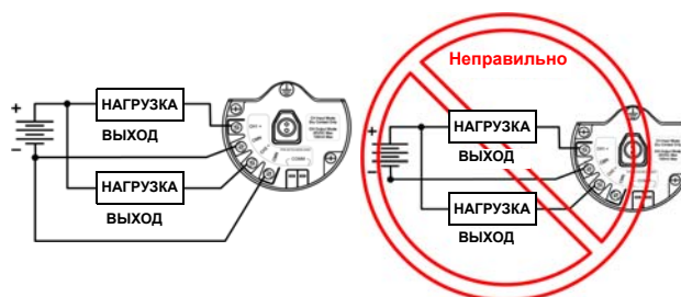
Рисунок 10. Двойные цепи выхода с одним источником питания
