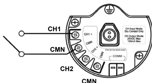
Рисунок 2. Одиночный, двойной вход
