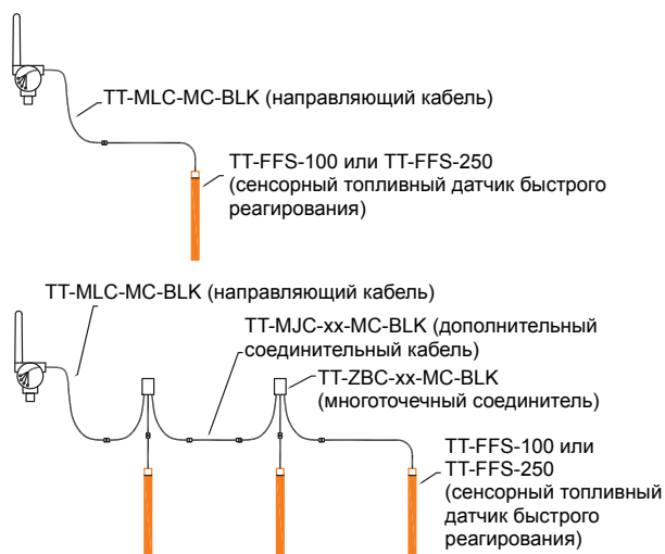
Рисунок 14. Схема подключения топливного датчика
