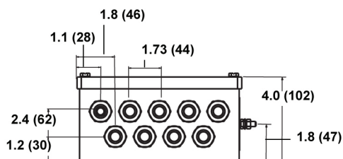
Вид спереди
