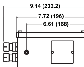
Вид сбоку
