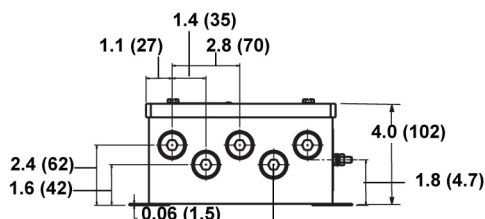
Вид спереди
