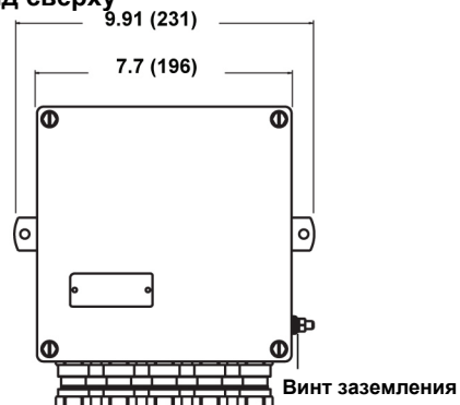
Вид сверху
