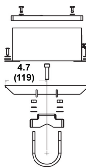
Вид спереди
