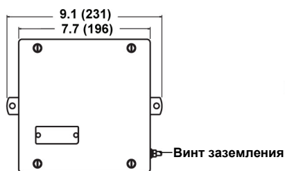
Вид спереди
