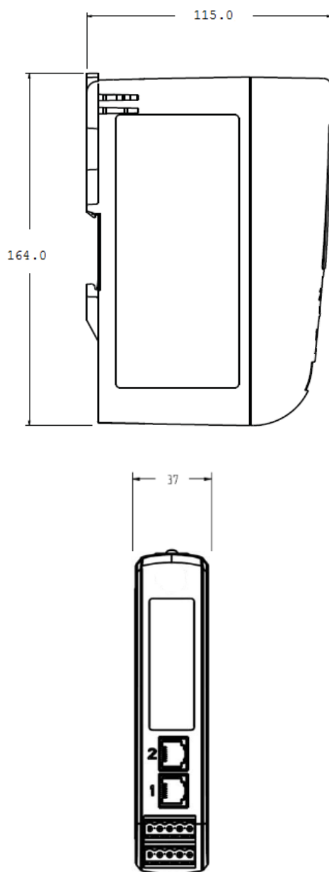
Рисунок 4. Интеллектуальный беспроводной шлюз
