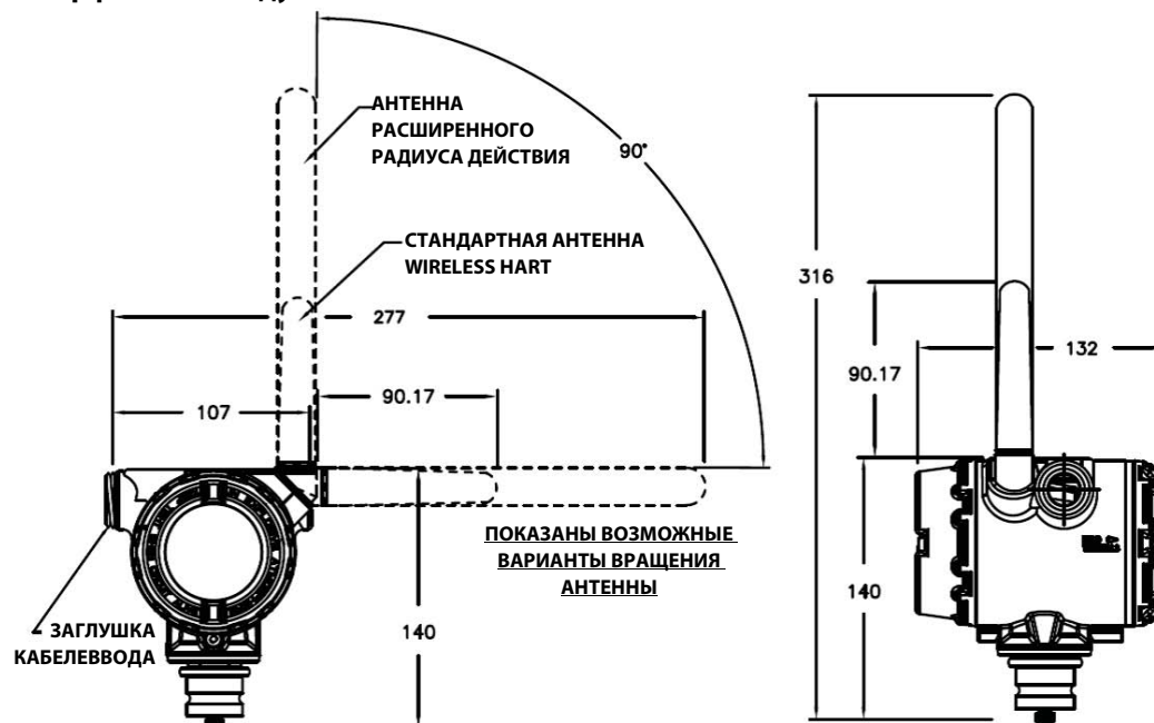
Рисунок 5. Интерфейсный модуль Smart Wireless Field Link
