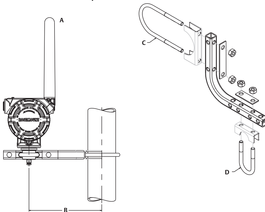
Рисунок 6. Конфигурация монтажа измерительного преобразователя Rosemount модели 781 с опциональным монтажным кронштейном
