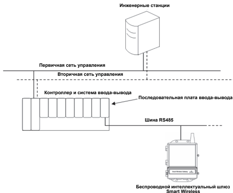
Рис.5-3. Архитектура ЛВС RS485
