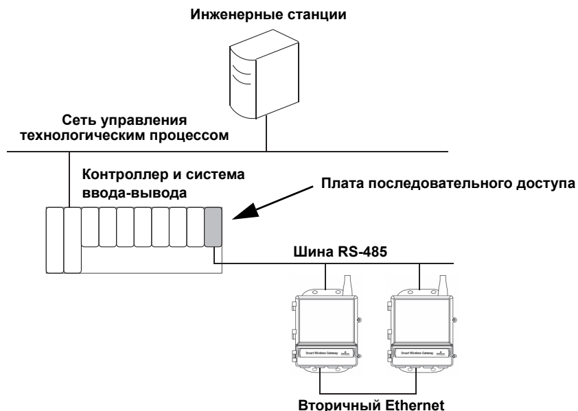
Рис.D-4. Архитектура одинарного порта RS-485
