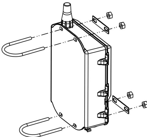
Рис.3-2. Трубный монтаж
