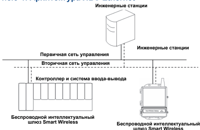
Рис.5-1. Архитектура ЛВС Ethernet
