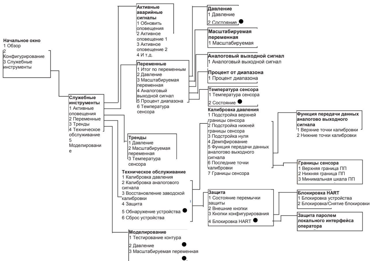
Рис. С-5. Древо меню полевого коммуникатора преобразователя 2051 - Служебные инструменты
