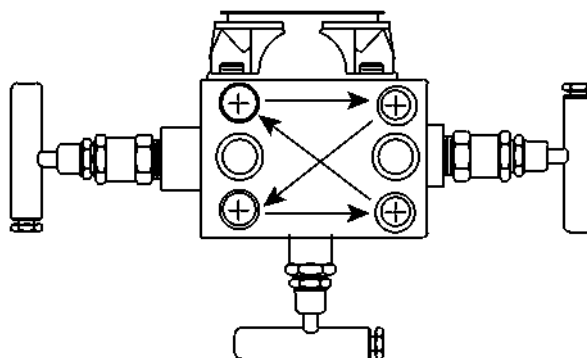
Рис. 3-13. Последовательность затяжки болтов
