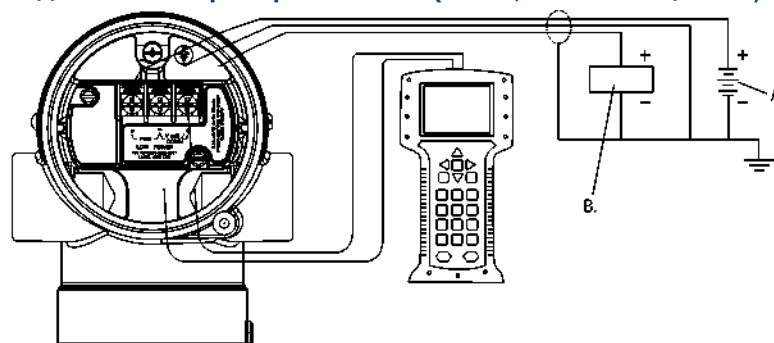
Рис. 2-2. Подключение преобразователя (1 - 5 В, малая мощность)
