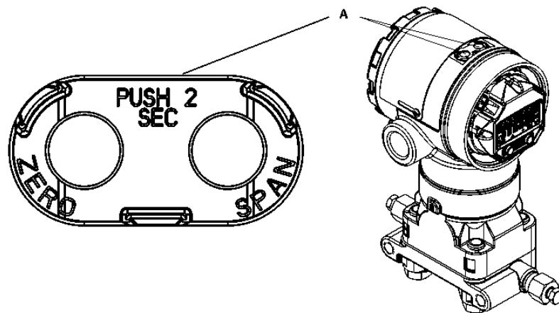
Рис. 2-10. Кнопки настройки аналогового нуля и шкалы
