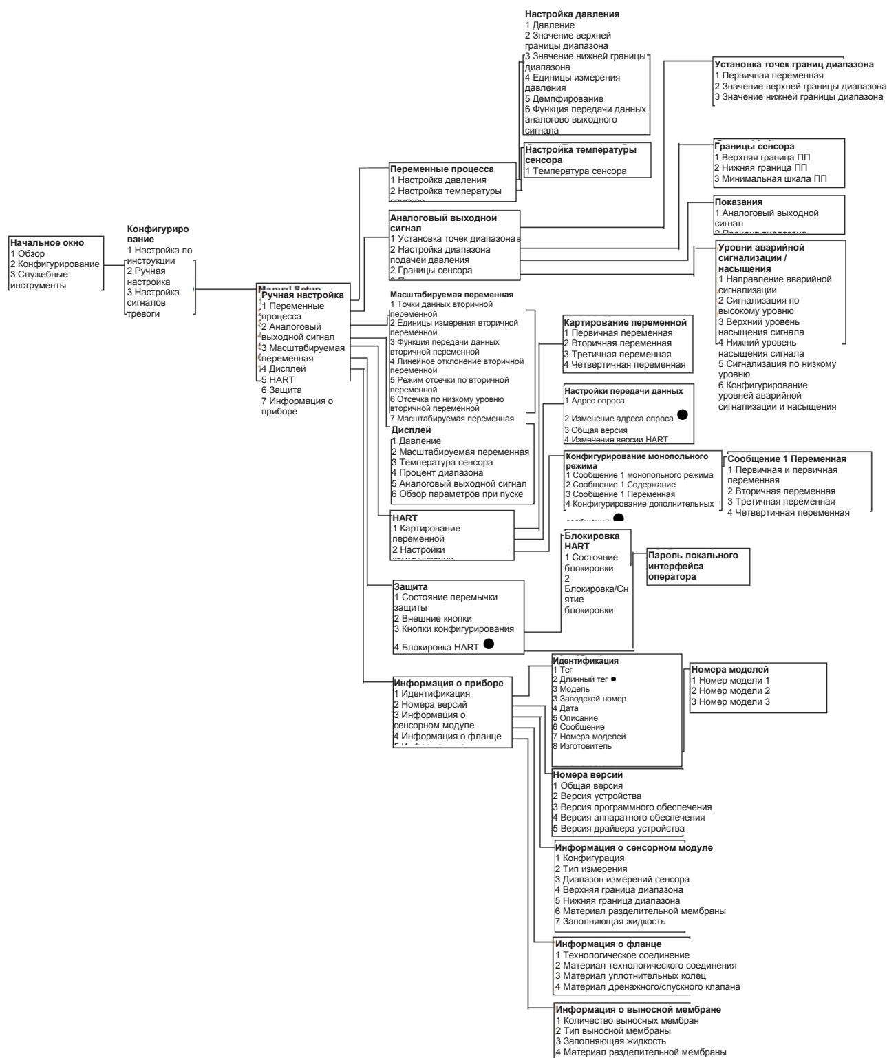
Рис. С-3. Древо меню полевого коммуникатора преобразователя 2051 Конфигурирование - ручная настройка
