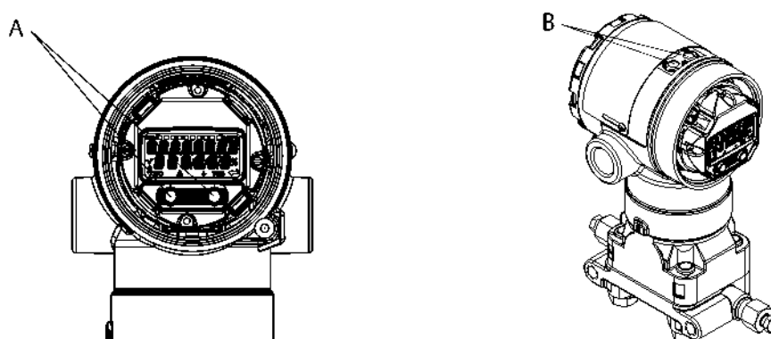
А. Внутренние кнопки конфигурирования В. Внешние кнопки конфигурирования
