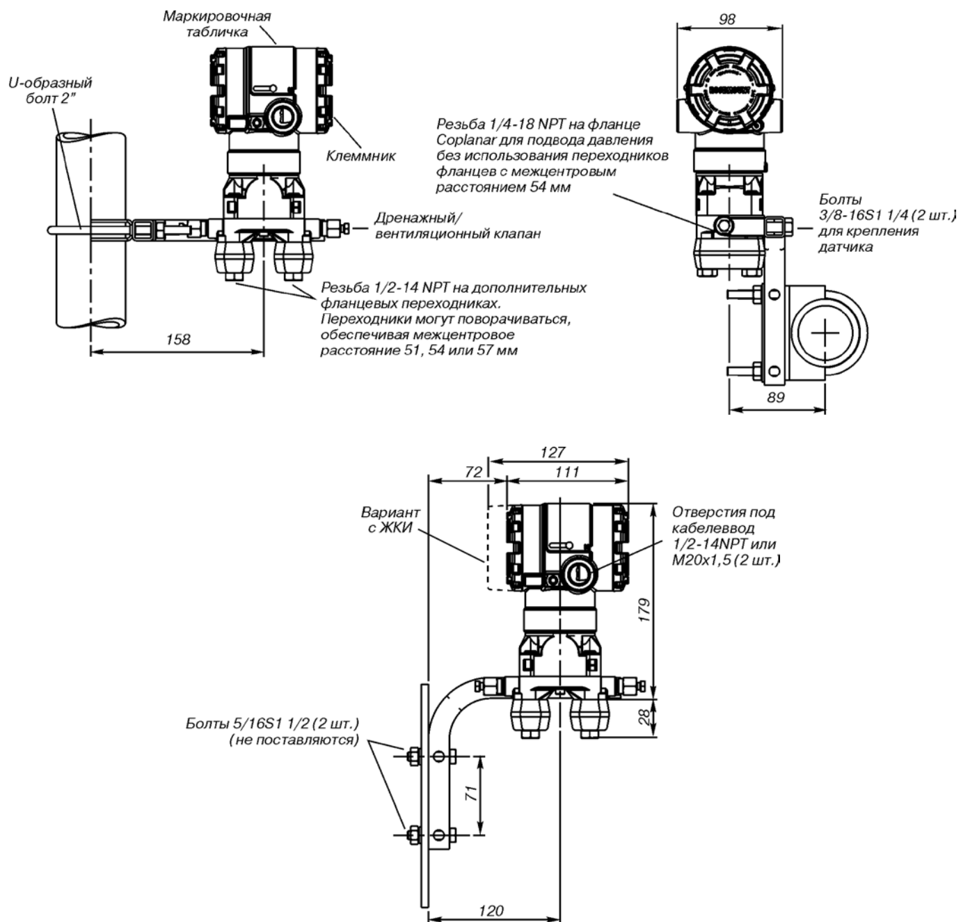
Рис.4. Преобразователь давления модели 2051C с фланцем Corplanar с дополнительным кронштейном (B4) для монтажа на 2-дюймовой трубе или панели.
