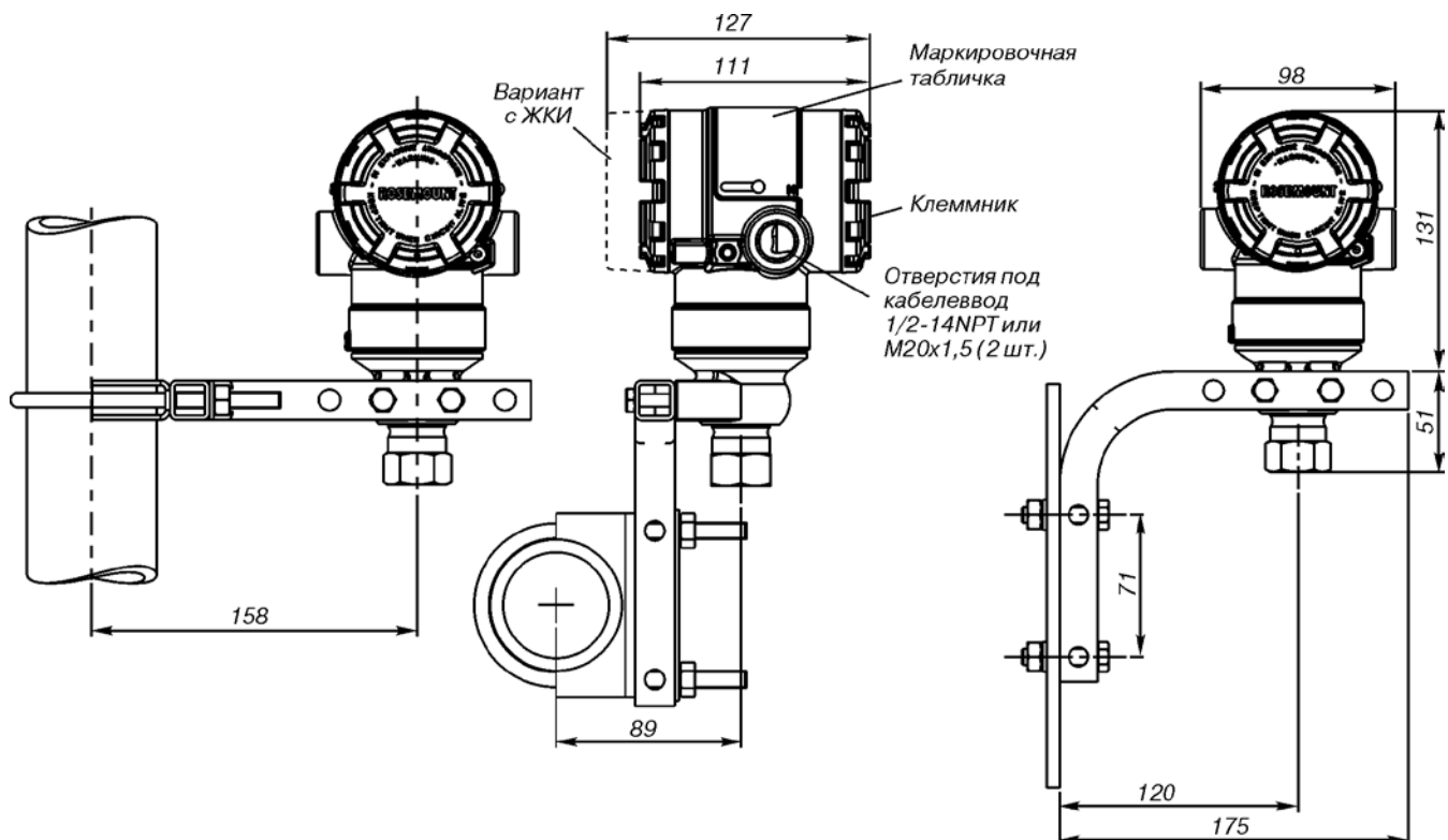
Рис.3. Преобразователь давления модели 2051T с дополнительным кронштейном (B4) для монтажа на 2-дюймовой трубе или панели.
