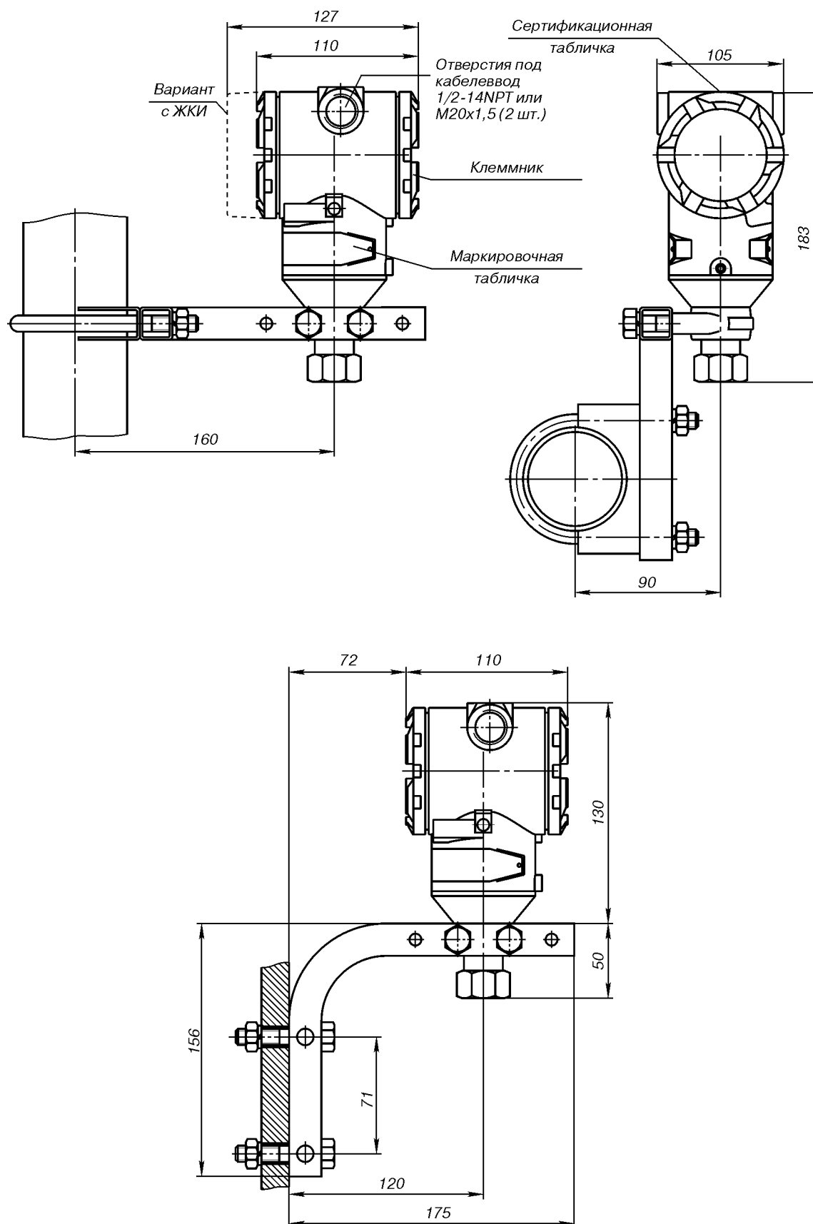
Рис.8. Преобразователь давления модели 3051T с кронштейном (B4) для монтажа на 2-дюймовой трубе или панели.
