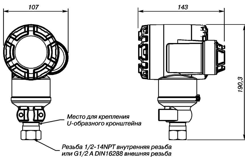
Рис. 11. Беспроводной измерительный преобразователь давления 3051Т.
