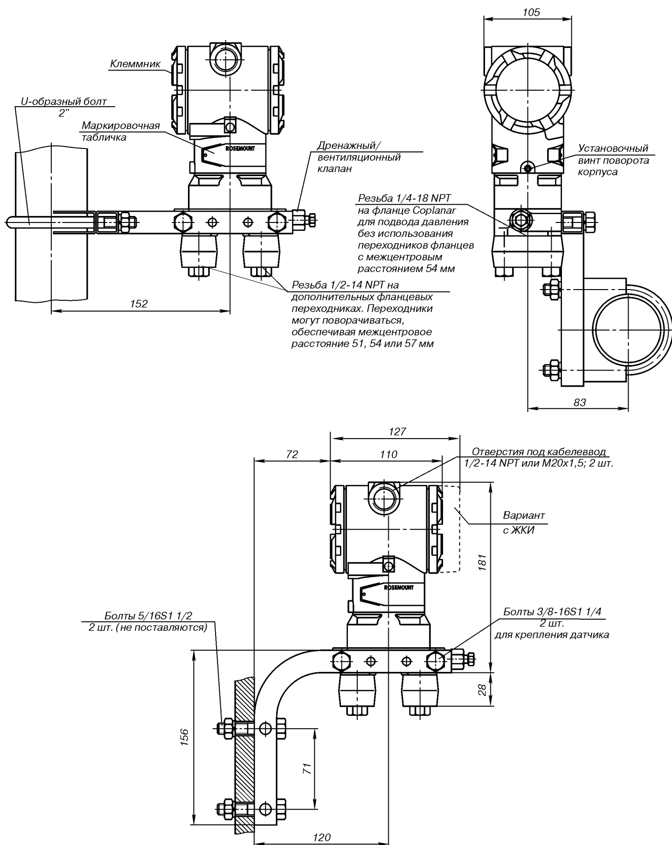
Рис. 7. Преобразователь давления модели 3051C с фланцем Coplanar с дополнительным кронштейном (B4) для монтажа на 2-дюймовой трубе или панели.
