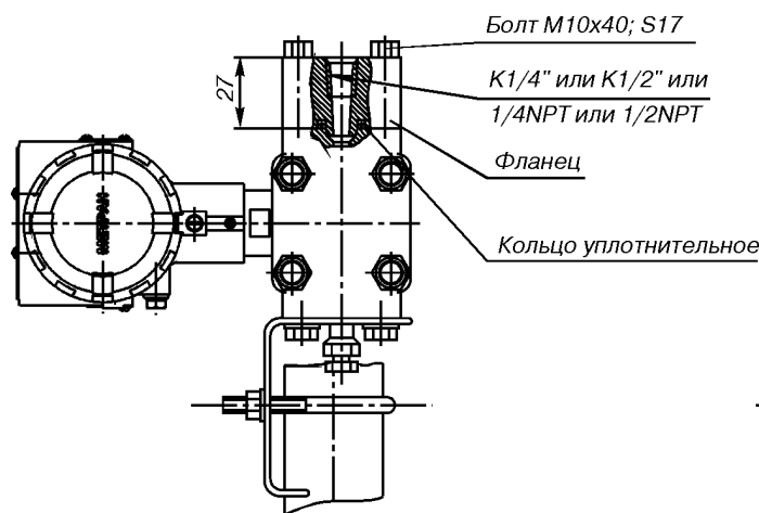
Рис.30. Датчики мод. 150CD с установленными монтажными фланцами с резьбовым отверстием K1/4" (код D1), или K1/2" (код D2), или 1/4NPT (код D3), или 1/2NPT (код D4) и монтажным кронштейном для установки на трубе ф50 мм (код В1). Остальное см.рис.27.
