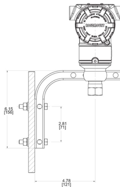
Монтаж на панели
