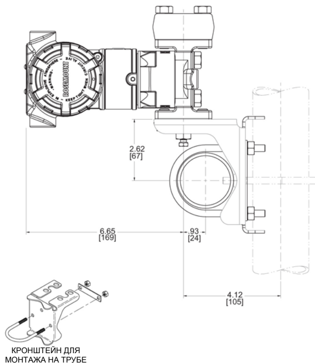
Кронштейн для монтажа на 2-дюймовой трубе (код опции В1/В7/В8)
