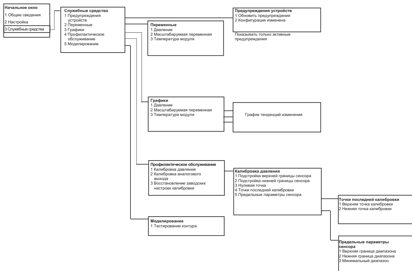
Рис. 3-7. Device Dashboard 3051S – Служебные средства
