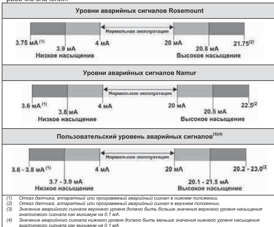
Рис. 6-1. Уровни аварийных сигналов
