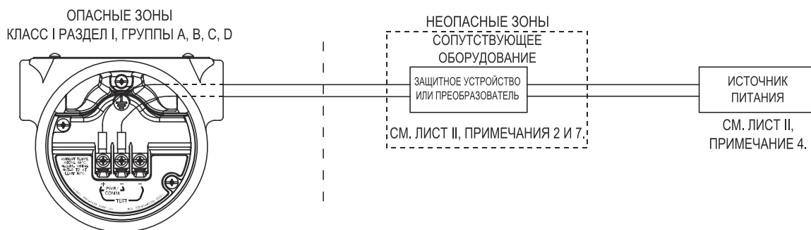
ПРИНЦИПИАЛЬНАЯ ЭЛЕКТРИЧЕСКАЯ СХЕМА 1 ОДНО ЗАЩИТНОЕ УСТРОЙСТВО ИЛИ ПРЕОБРАЗОВАТЕЛЬ ОДИН ИЛИ ДВА КАНАЛА
