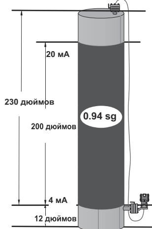
Рис. 3-9. Пример резервуара
