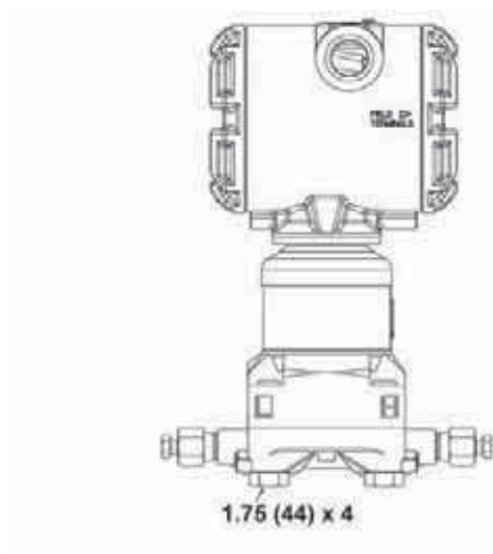
Датчик с болтами фланца
