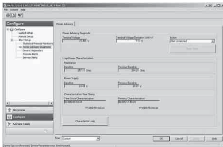
Рис. 7-18. Ручная настройка основного окна функции Power Advisory
