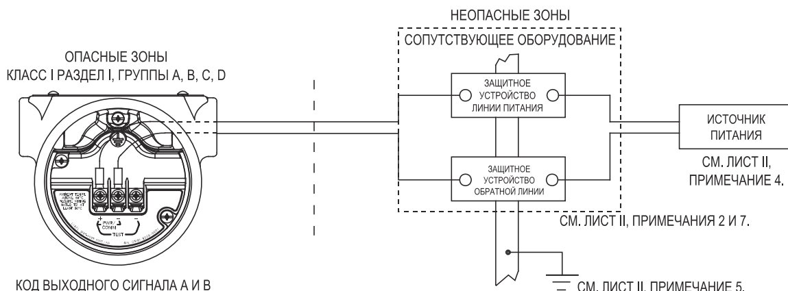
ПРИНЦИПИАЛЬНАЯ ЭЛЕКТРИЧЕСКАЯ СХЕМА 2 ЗАЩИТНЫЕ УСТРОЙСТВА НА ЛИНИИ ПИТАНИЯ И ВОЗВРАТА (ТОЛЬКО ДЛЯ ИСПОЛЬЗОВАНИЯ С ЗАЩИТНЫМИ УСТРОЙСТВАМИ, УТВЕРЖДЕННЫМИ В ДАННОЙ КОМПОНОВКЕ)
