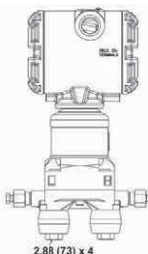
Датчик с фланцевыми переходниками и болтами фланца/переходника
