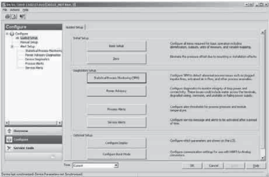
Рис. 7-7. Меню пошаговой настройки
