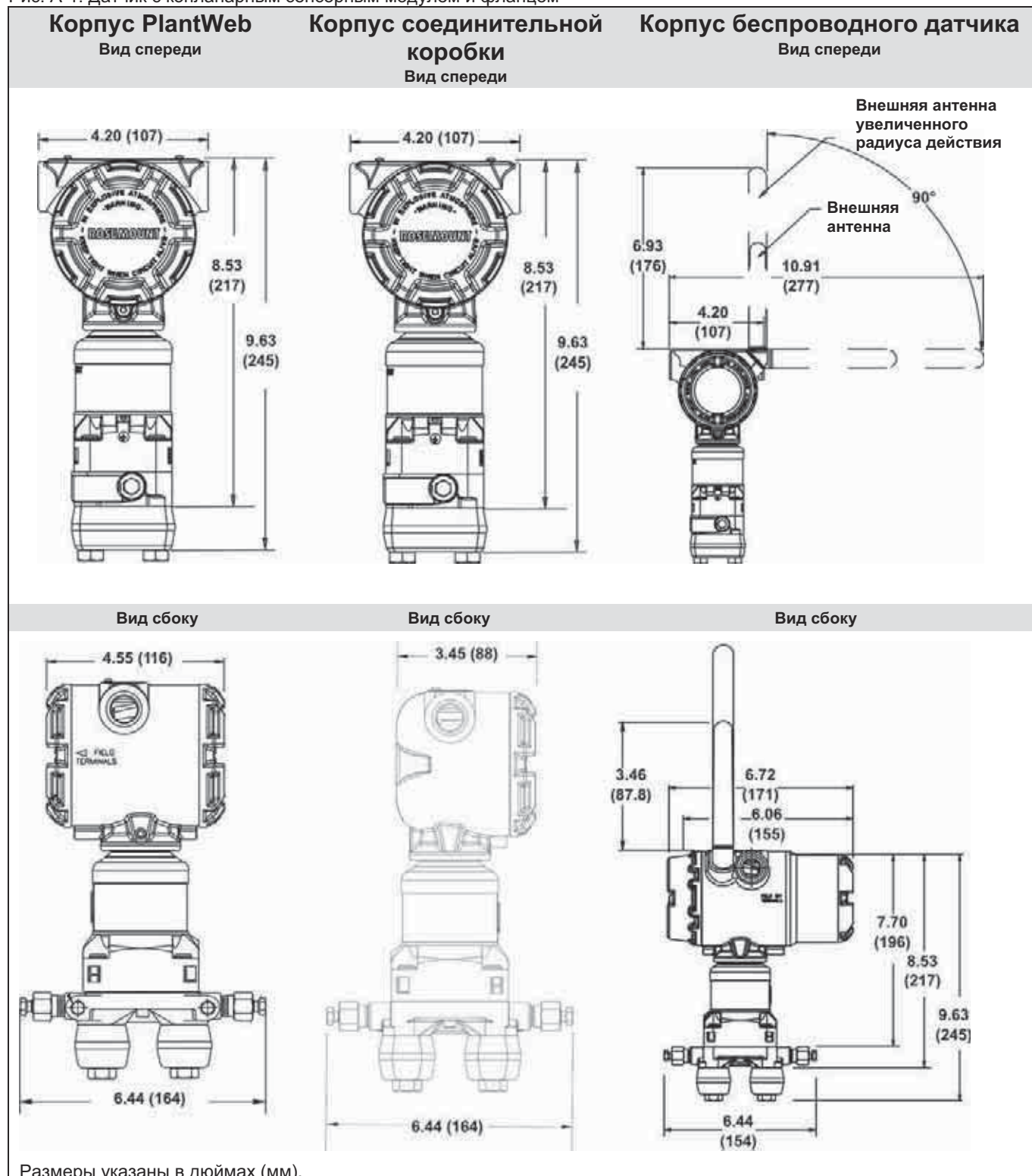
Рис. А-1. Датчик с копланарным сенсорным модулем и фланцем
