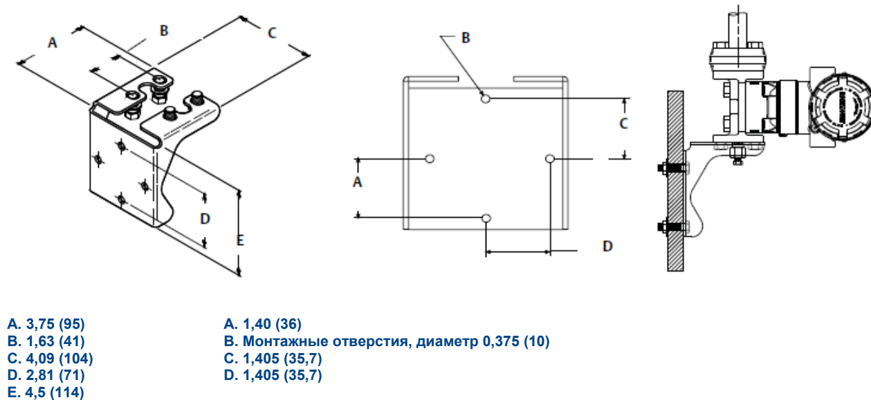
Рис. 3-5. Коды опции монтируемого на панели кронштейна В2 и В8
