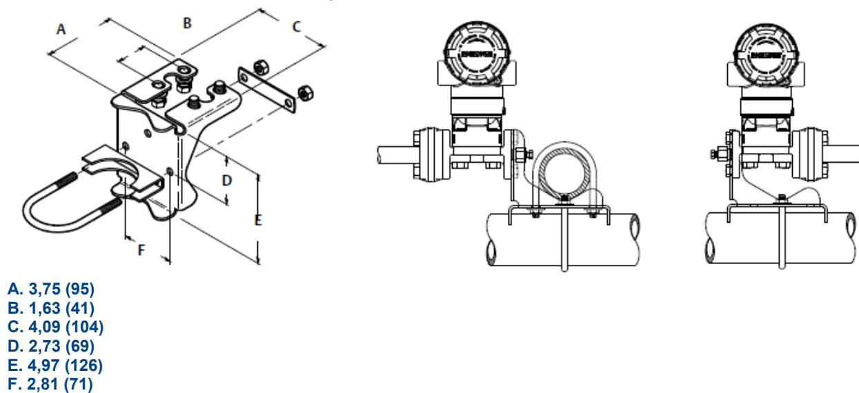
Рис. 3-4. Коды опции монтажного кронштейна В1, В7 и ВА
