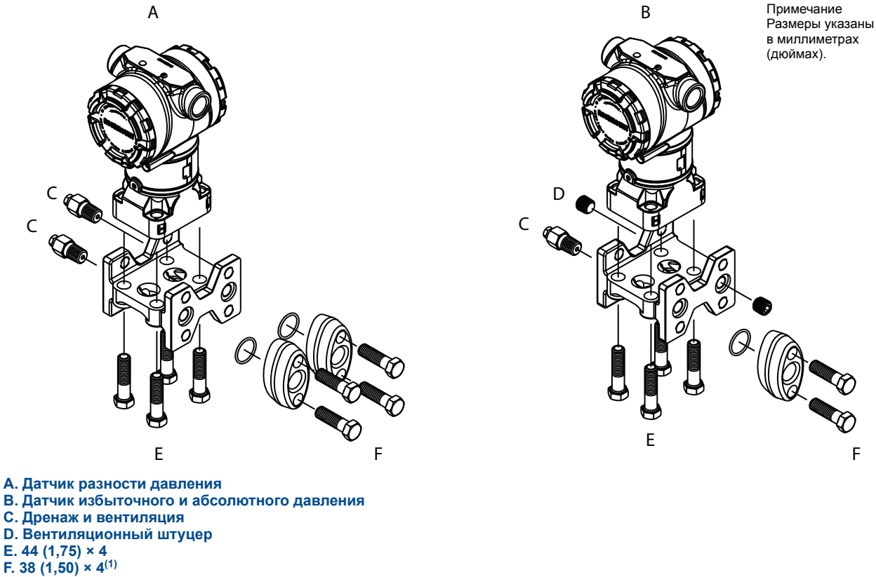
Рис.3-3. Варианты болтового крепления преобразователя с традиционным фланцем
