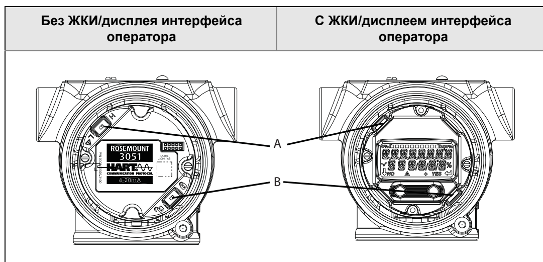
Рис.4-2. Плата электроники
