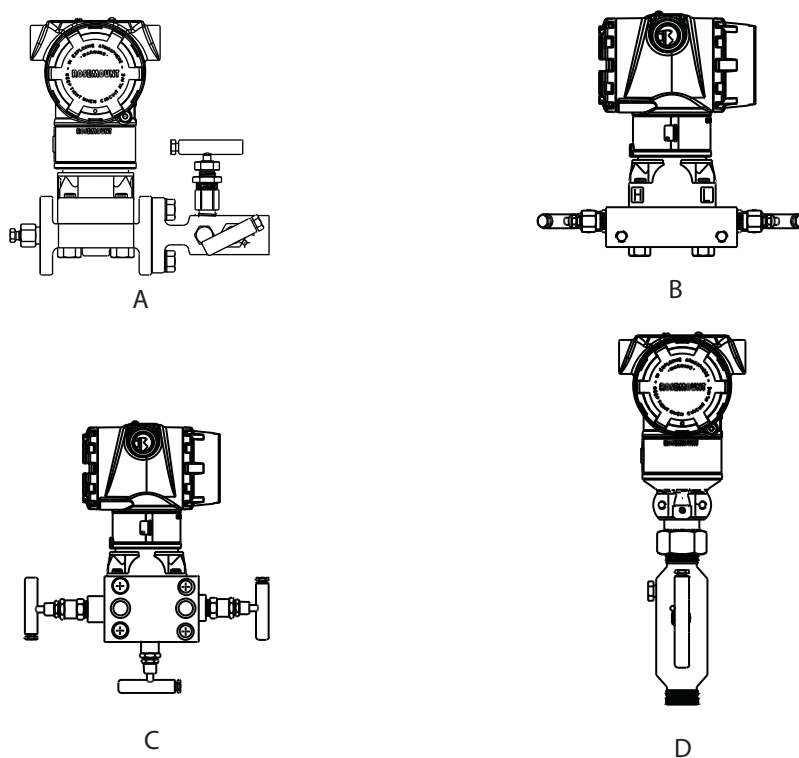
Рис.3-11. Клапанные блоки
