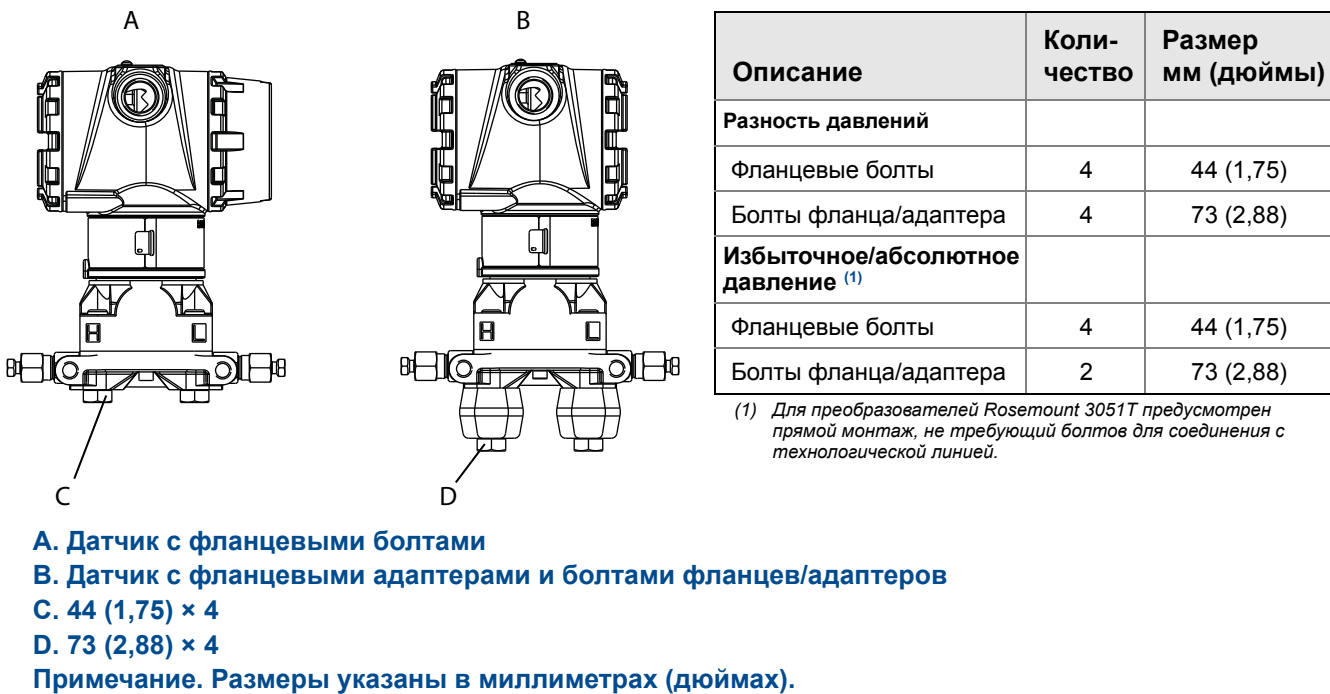
Рис.3-4. Болты и болтовое крепление преобразователей с фланцем Corplanar
