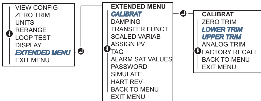
Рис.5-3. Подстройка первичного преобразователя с локальным интерфейсом пользователя
