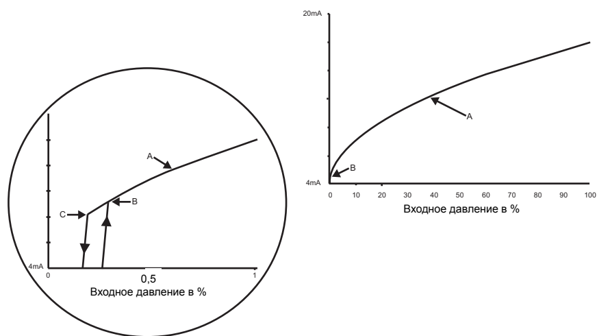
Рис.2-6. Точка перехода среднеквадратичного выходного сигнала HART 4–20 мА
