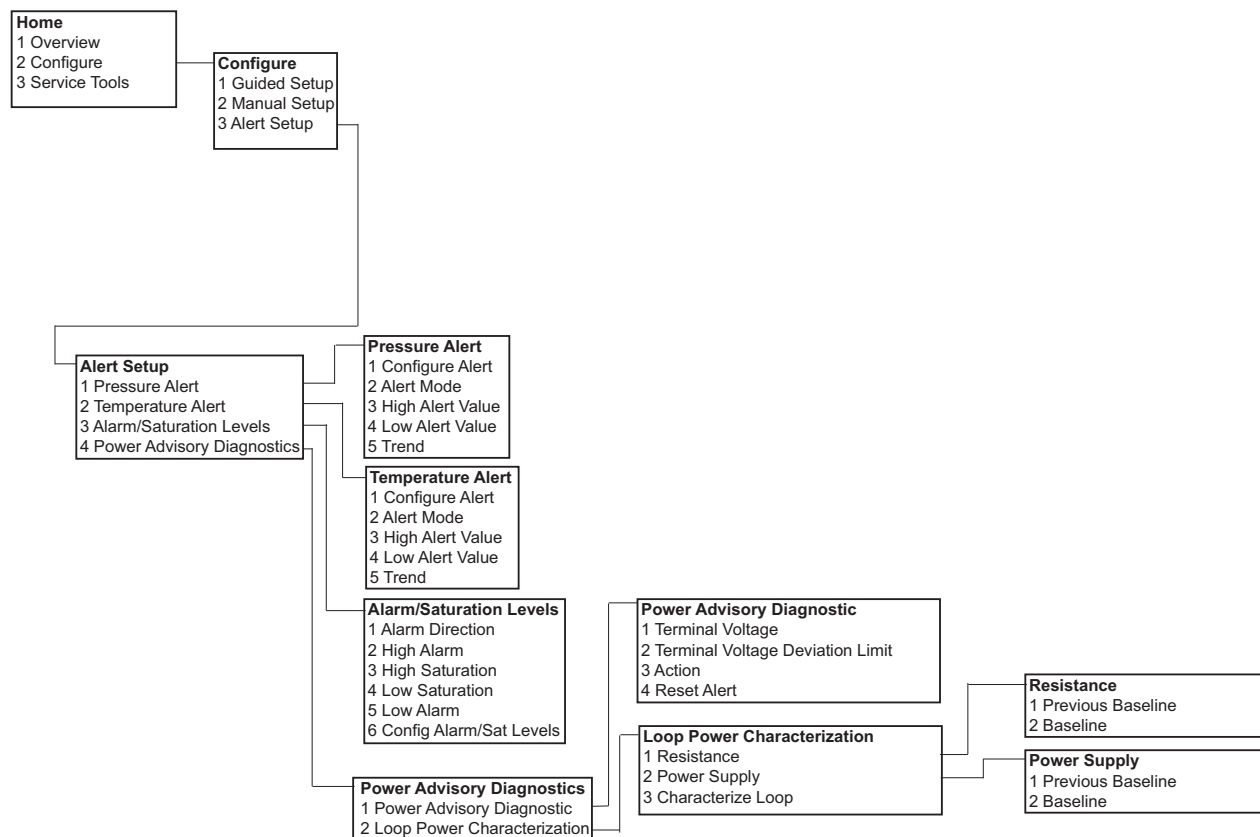
Рис.С-4. Система меню полевого коммутатора Rosemount 3051: Конфигурация – настройка сигнала тревоги
