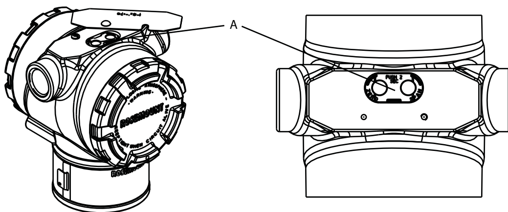
Рис.2-9. Кнопки регулировки нуля аналогового выхода и диапазона шкалы
