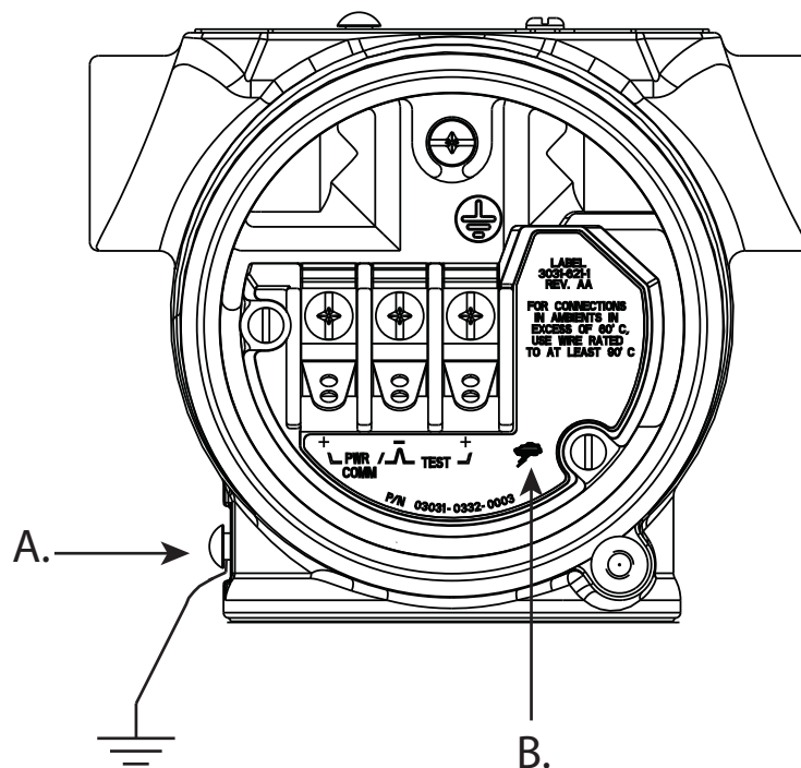
Рис.4-10. Клеммный блок с защитой от переходных процессов
