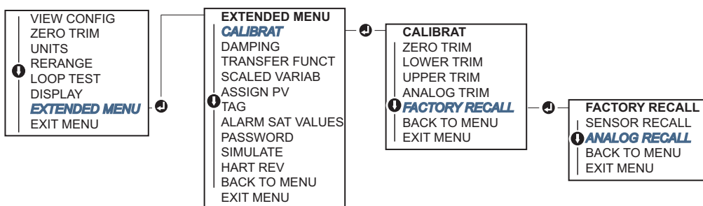
Рис.5-7. Восстановление заводской настройки – аналогового выхода с помощью локального интерфейса оператора
