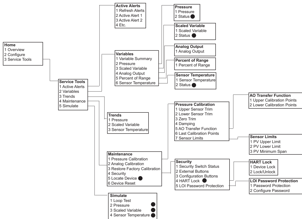
Рис.С-5. Дерево меню полевого коммуникатора Rosemount 3051 – служебные инструменты
