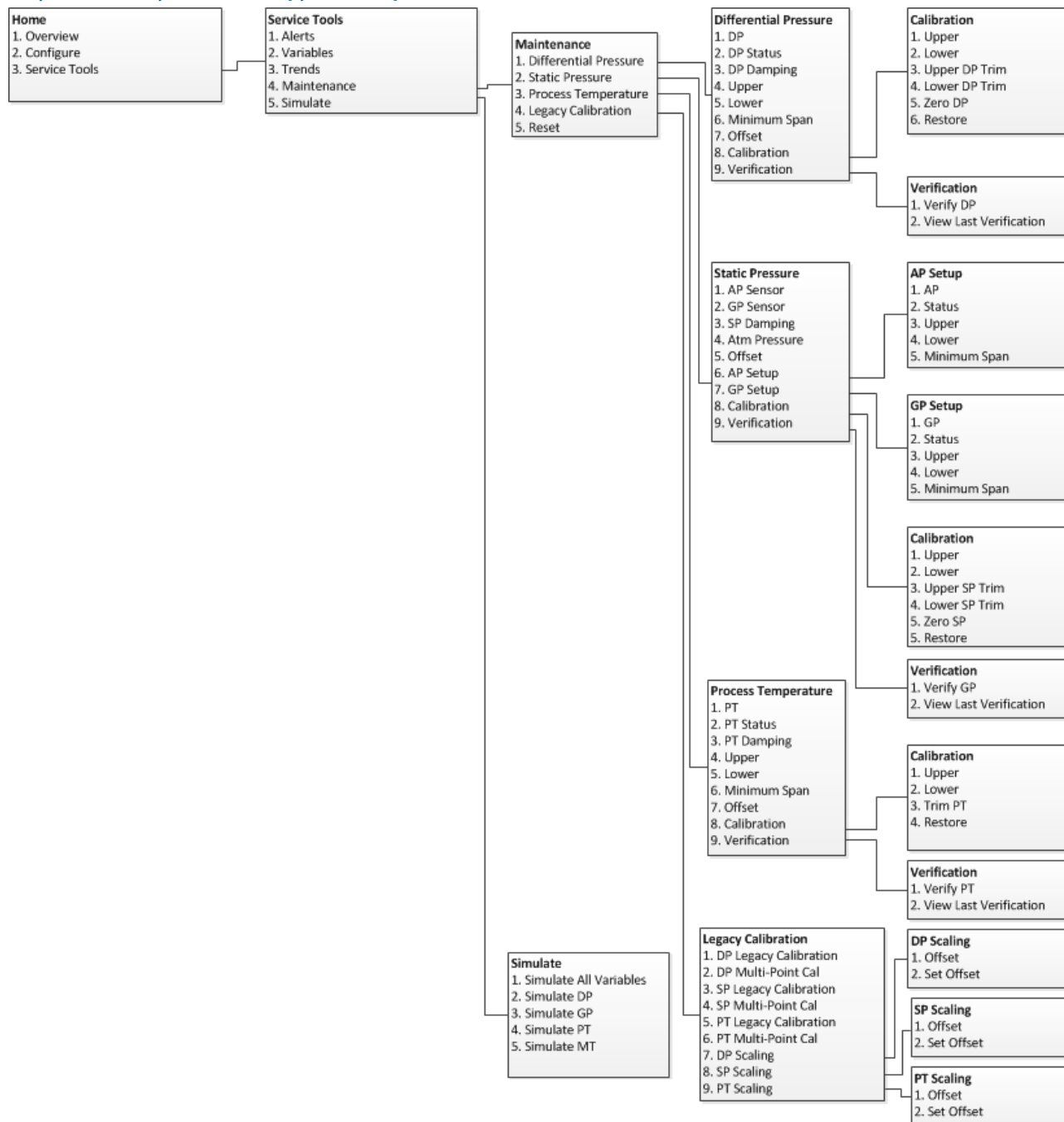
Рисунок 4-17. Служебные инструменты (продолжение)
