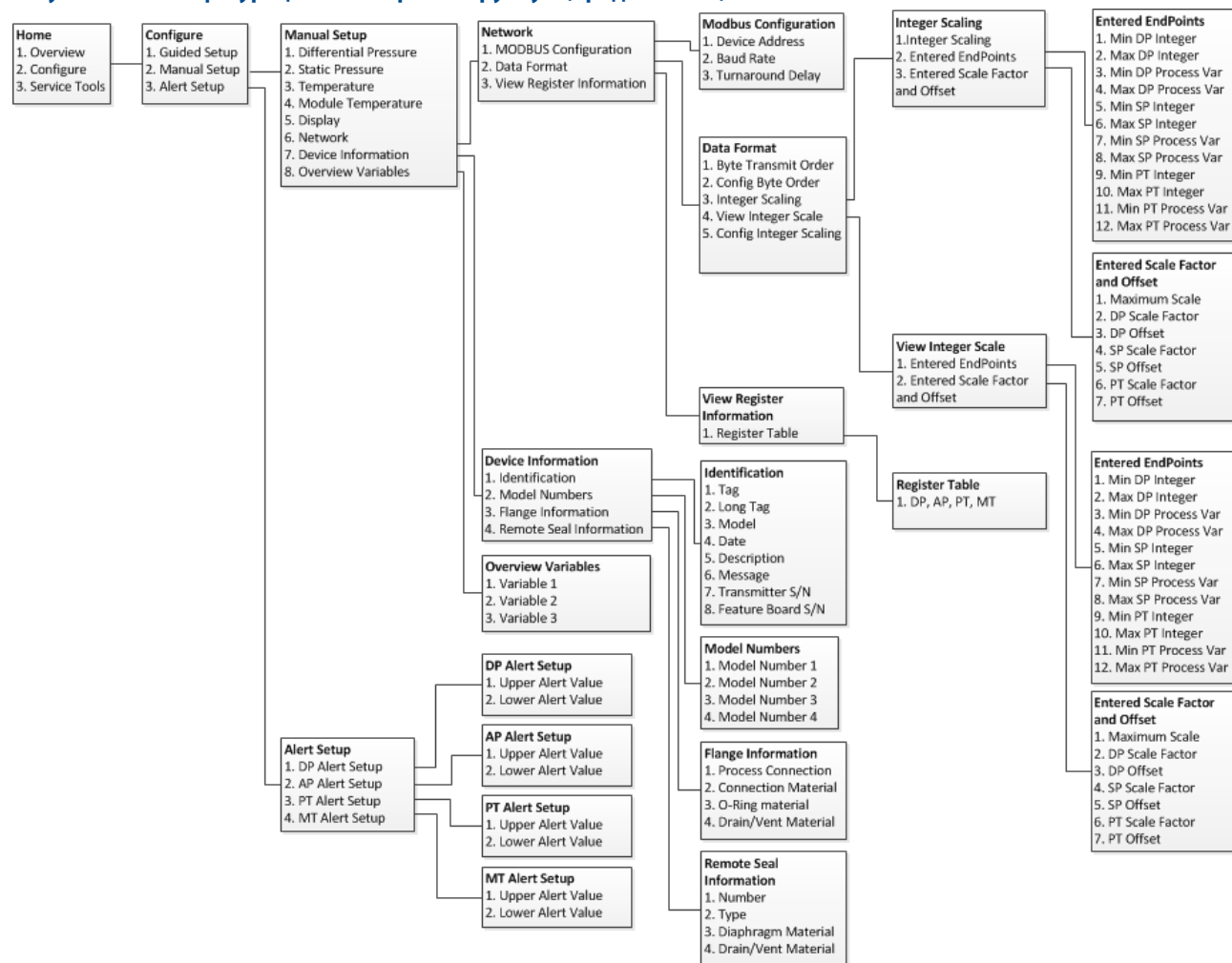
Рисунок 4-15. Конфигурация — Настройка вручную (продолжение)
