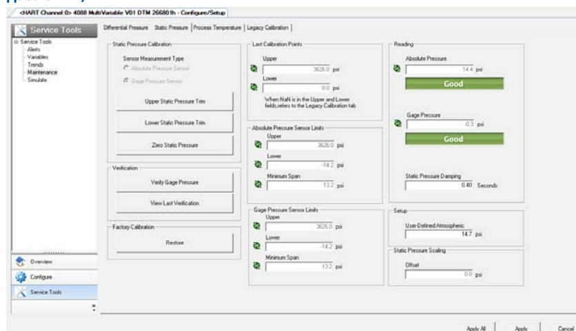
Рисунок 5-2. Калибровка — вкладка Static Pressure Calibration (Калибровка статического давления)
