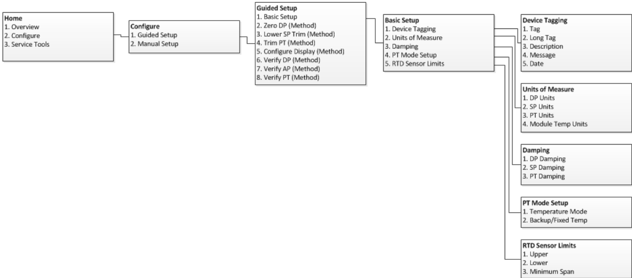
Рисунок 4-13. Конфигурация — Пошаговая настройка
