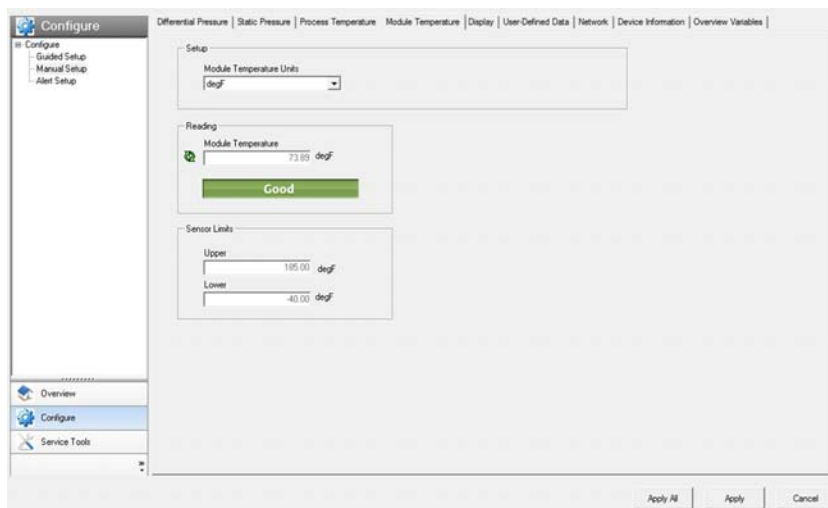
Рисунок 4-11. Вкладка Module Temperature (Температура модуля)
