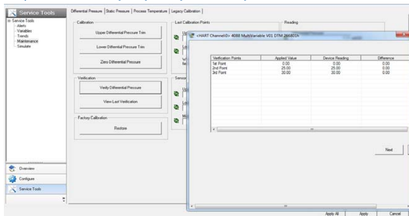
Рисунок 5-4. Метод проверки переменной процесса
