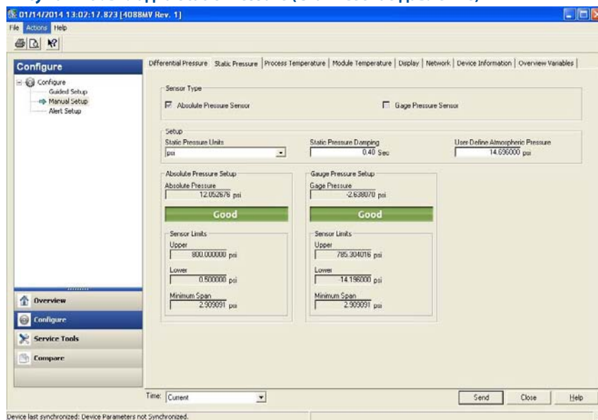
Рисунок 4-9. Вкладка Static Pressure (Статическое давление)
