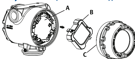
Рисунок 6-5. Опциональный ЖК-дисплей
