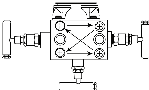
Рисунок 2-12. Схема затяжки болтов
