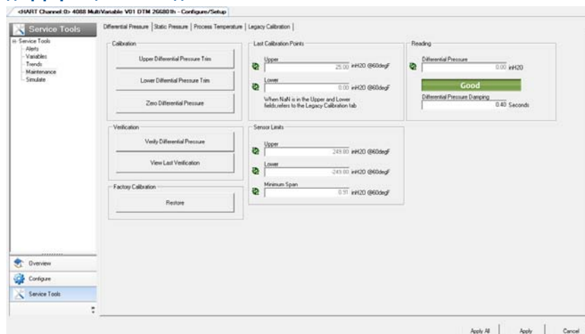
Рисунок 5-1. Калибровка — вкладка Differential Pressure Calibration (Калибровка дифференциального давления)
