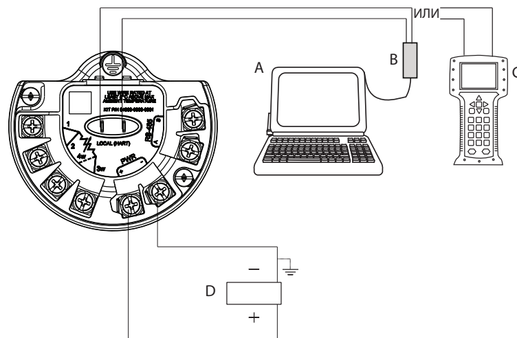
Рисунок 4-1. Подключение персонального компьютера к измерительному преобразователю
