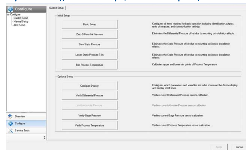
Рисунок 4-2. Вкладка «Guided Setup» (Пошаговая настройка)
