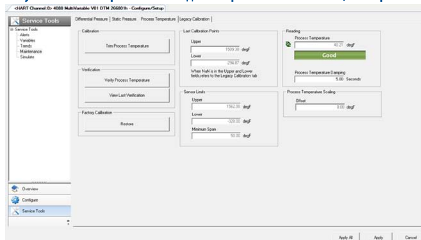
Рисунок 5-3. Калибровка — вкладка Temperature Calibration (Калибровка температуры)
