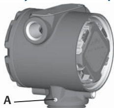
Рисунок 6-2. Стопорный винт
