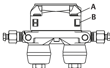
Рисунок 2-3. Правильная установка болтов
