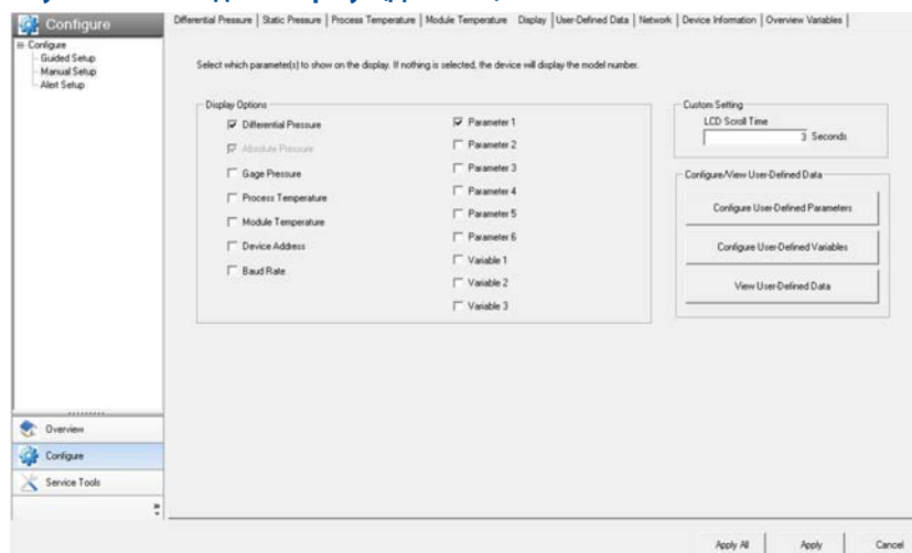
Рисунок 4-4. Вкладка «Display» (Дисплей)
