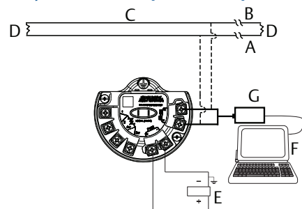
Рисунок 4-18. Настройка измерительного преобразователя через сетевой порт RS-485
