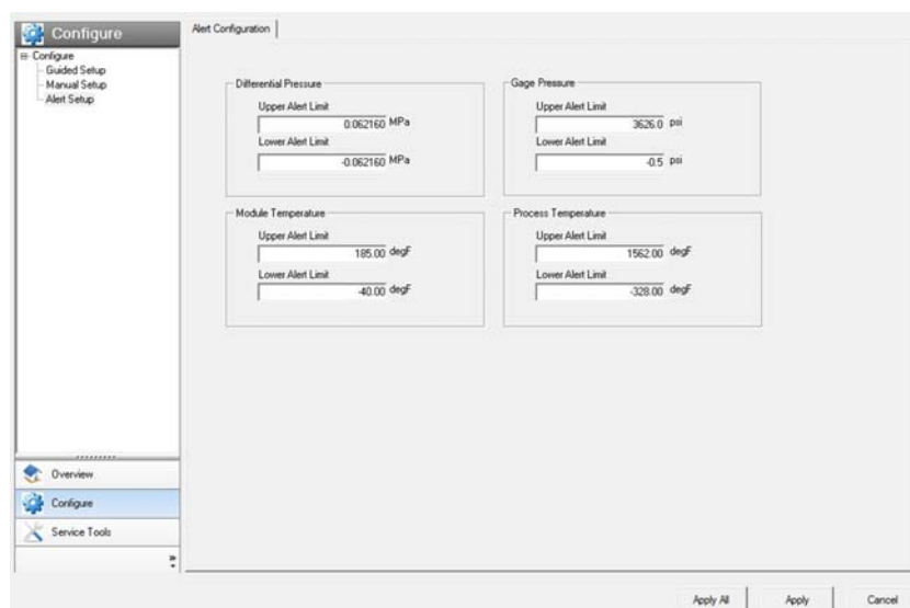
Рисунок 4-7. Вкладка «Alert Configuration» (Конфигурация сигналов тревоги)
