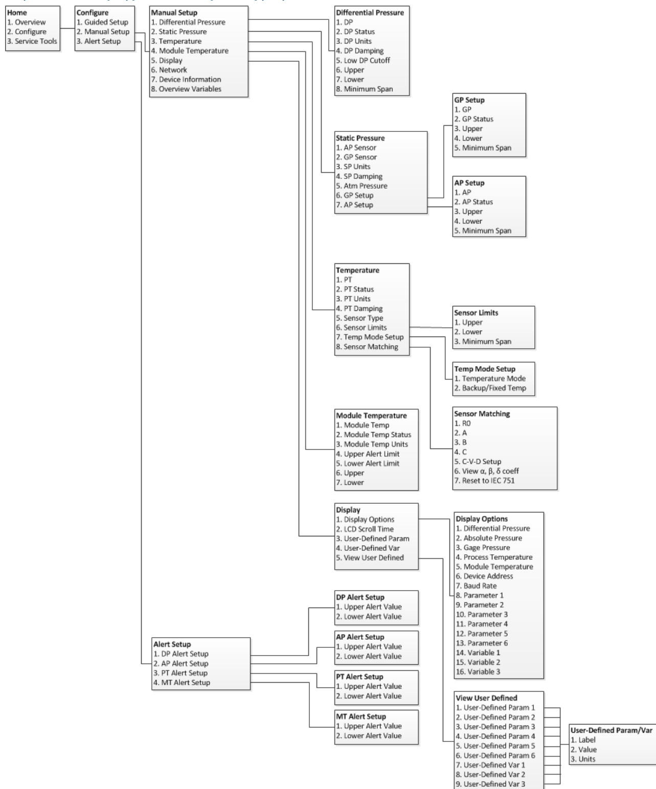
Рисунок 4-14. Конфигурация — Настройка вручную
