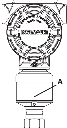
Рисунок 2-4. Штуцерный измерительный преобразователь
