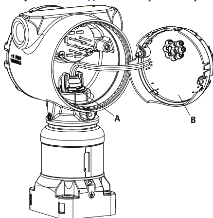
Рисунок 6-1. Вид коннектора сенсорного модуля
