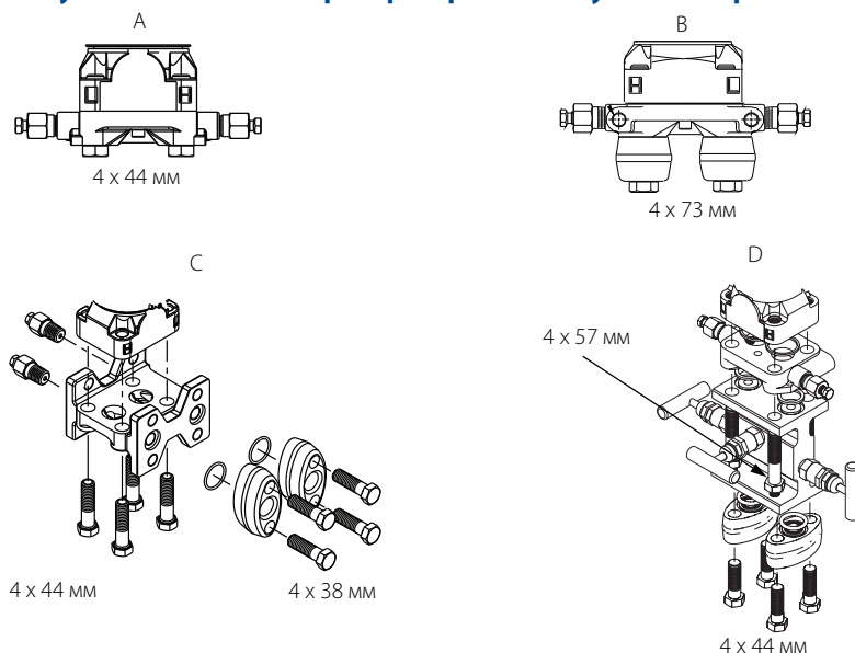
Рисунок 2-1. Наиболее распространенные узлы измерительного преобразователя
