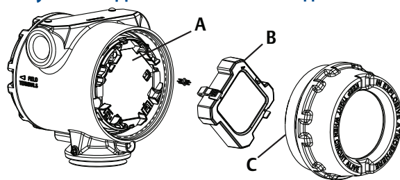
Рисунок 2-6. Дополнительный ЖК-дисплей
