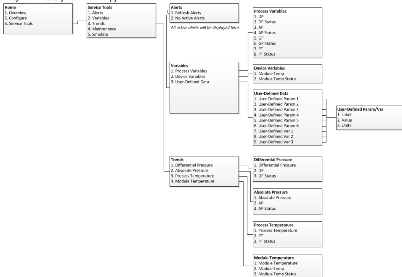
Рисунок 4-16. Службные инструменты
