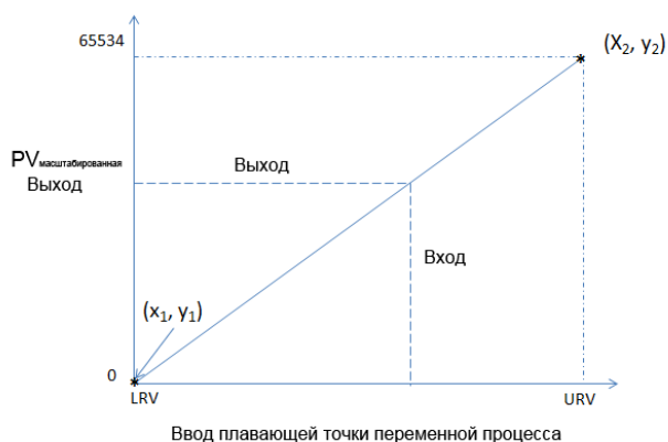
Рисунок 3-1. Целочисленное масштабирование
