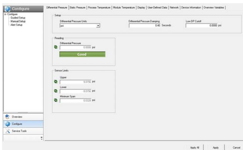
Рисунок 4-8. Вкладка «Differential Pressure» (Дифференциальное давление)
