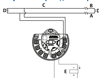
Рисунок 2-8. Проводка измерительного преобразователя для шины RS-485
