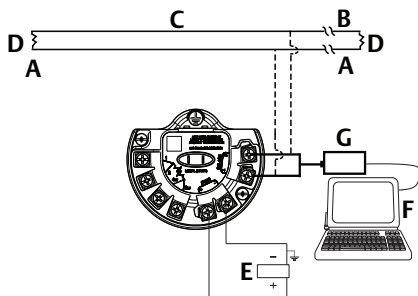
Рисунок 9. Настройка Rosemount 4088 MultiVariable через сетевой порт RS-485
