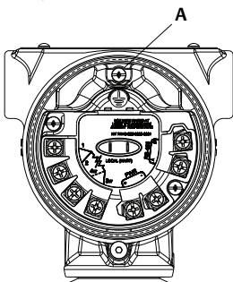
Рисунок 11. Подсоединение к внутреннему выводу заземления
