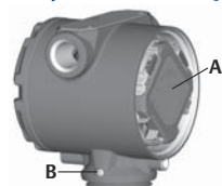
Рисунок 5. Стопорный винт корпуса измерительного преобразователя
