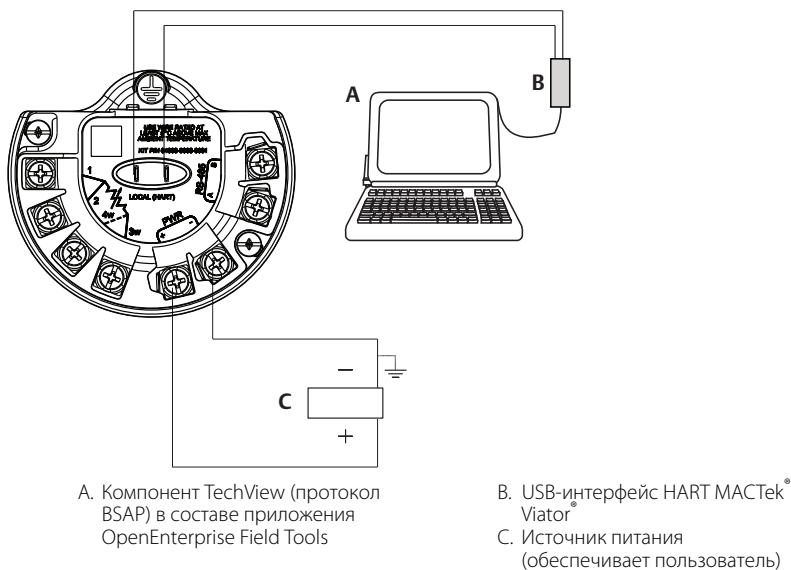
Рисунок 8. Настройка Rosemount 4088 MultiVariable через порт HART® или BSAP (локальный)
