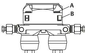
Рисунок 3. Правильная установка болтов
