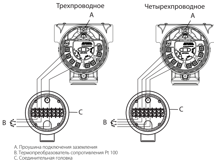
Рисунок 13. Подключение кабеля ТПС многопараметрического преобразователя Rosemount 4088 MultiVariable
