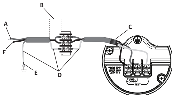
Рисунок 10. Проводка заземления сигнального кабеля
