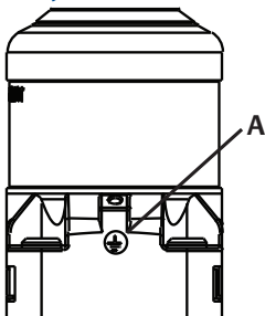
Рисунок 12. Внешнее подсоединение заземления
