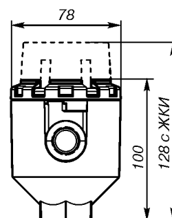
Рис. 9. Соединительная головка исполнения DIN (код исполнения R1, R2, R3 или R4).
