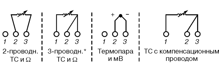
Рис. 10. Схема подключения ПП к преобразователю Rosemount 848T.
