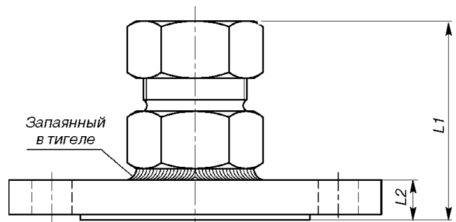
Рис.6. Регулируемые фланцы.
