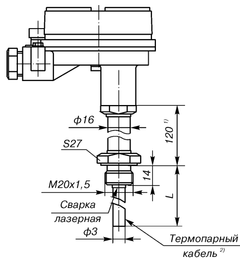
Рис.19 (ост.см.рис.1) (штуцер неподвижный) Метран-281-19, Метран-281-19-Exia
