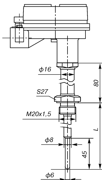
Рис.6 2) (ост.см.рис.4) (штуцер неподвижный) Метран-286-06-Exd
