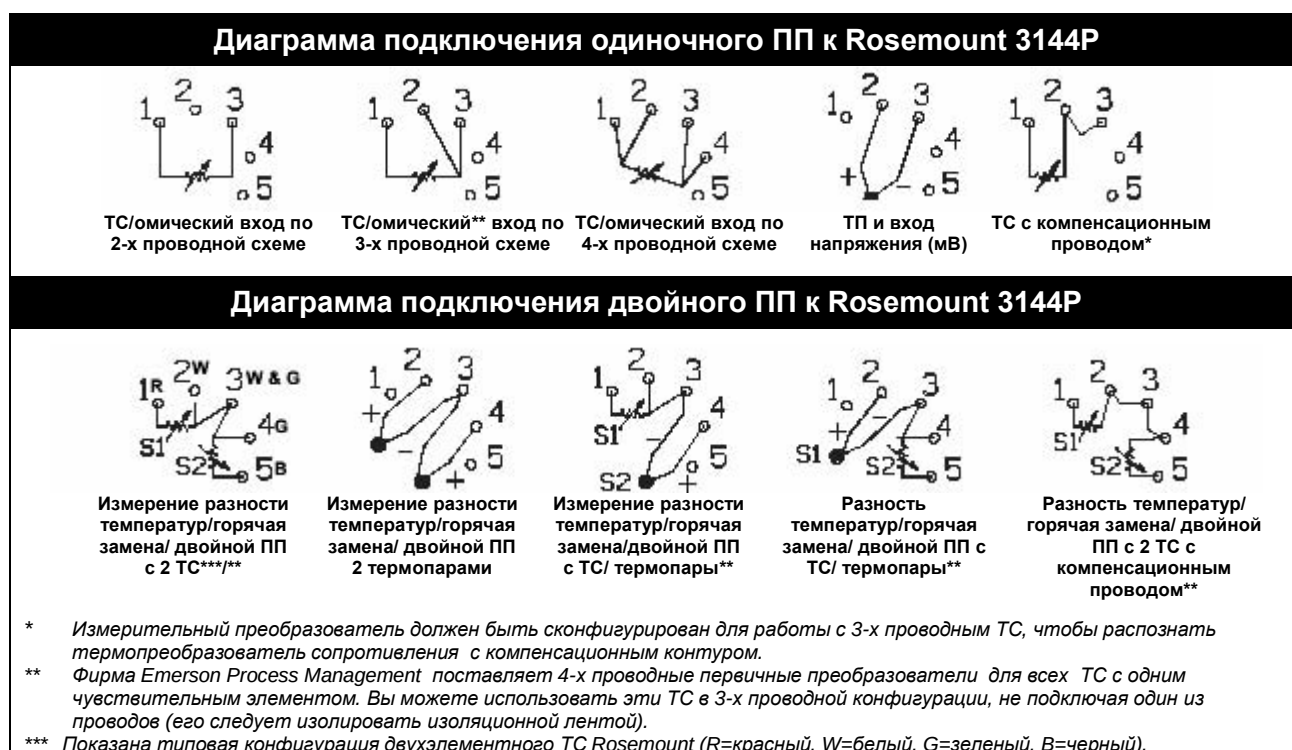
Рисунок 2-9. Схема подключения первичных преобразователей HART / 4-20 мА
