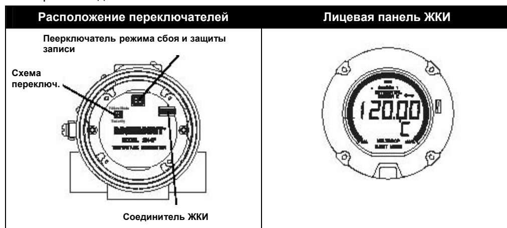
Рисунок 7-1. Расположение перемычек датчика
