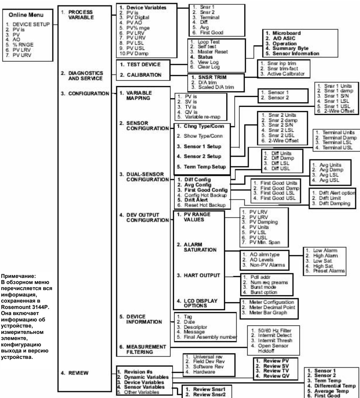
Рисунок 3-1. Дерево меню Коммуникатора HART 375
