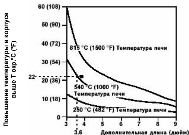
Рисунок 1-1. Корпус измерительного преобразователя Rosemount 3144P. Зависимость повышения температуры от дополнительной длины. Контрольная установка.
