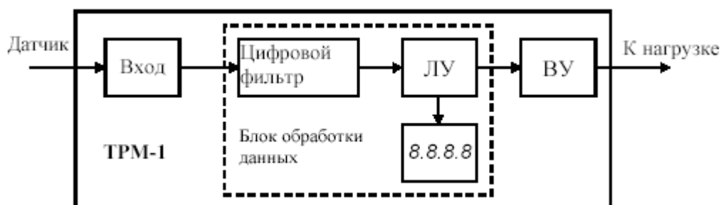
Рис. 6.2. Функциональная схема прибора ТРМ-1
