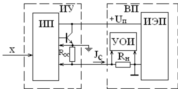
Рис. 2.39. до 20 мА. Схема измерения выходного тока измерительного преобразователя снимает сигнал с R_{OC} вычисляет рассогласование и
