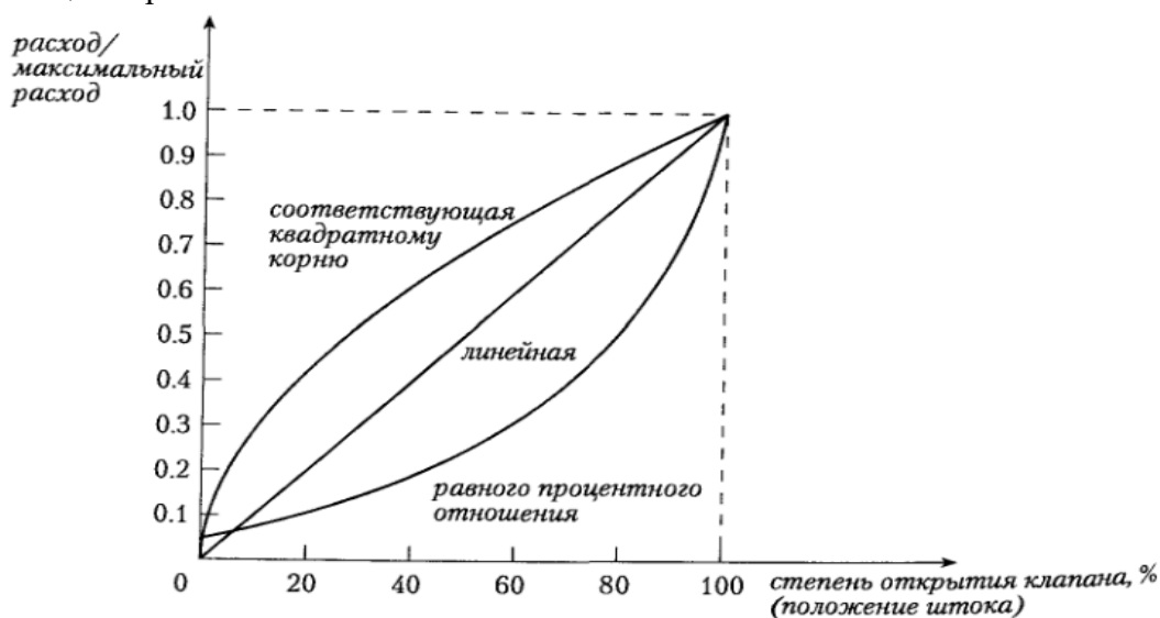
Рис. 9.2. Характеристики клапанов
