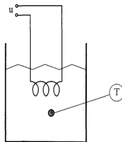
Рис. 1.4 Простая система регулирования температуры
