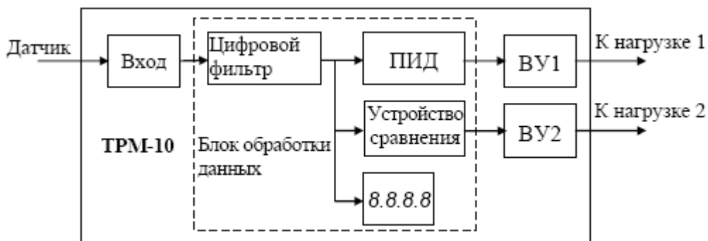
Рис. 6.4. Функциональная схема прибора ТРМ-10
