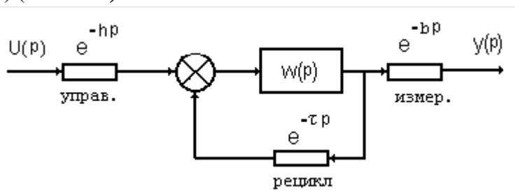
Рис. 10.2. Объект управления с запаздыванием.
