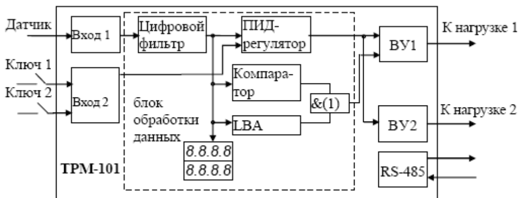
Рис. 6.5. Функциональная структура TPM-101
