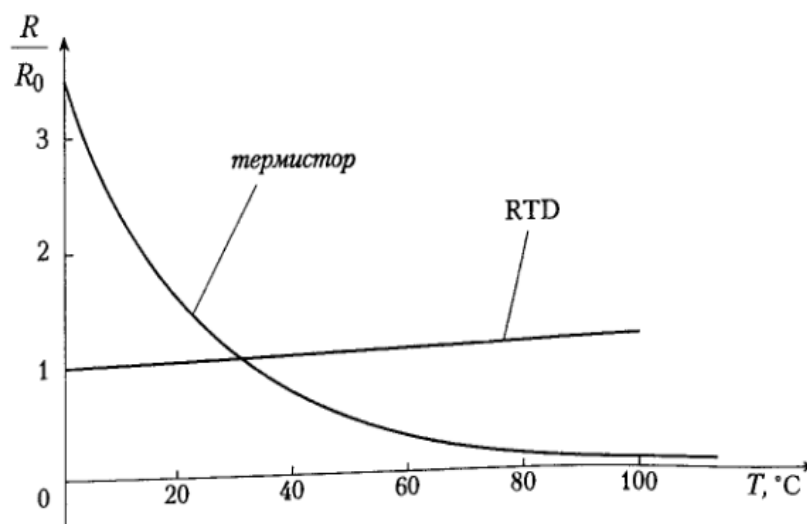
Рис. 2.15. Температурная характеристика сопротивления резистивного детектора температуры и термистора
