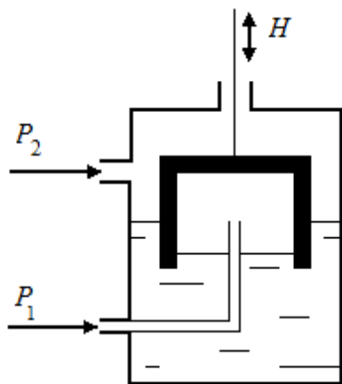
Рис. 4.2. Колокольный дифманометр
