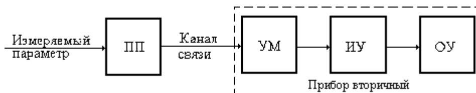
Рис. 1.1. Структурная схема измерительного прибора
