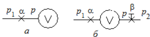
Рис. 9.2. Условное изображение глухой и проточной камер
