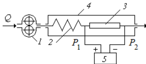
Рис. 7.25. Схема капиллярного вискозиметра
