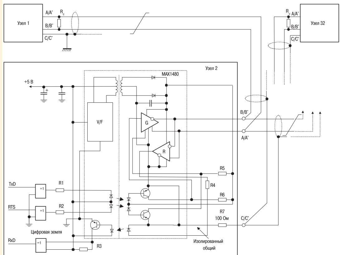
Рис. 13. Способ объединения приемопередатчиков EIA RS-485 с гальванической изоляцией
