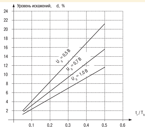
Рис. 15. График зависимости уровня искажений сигнала на входе приемника от минимального напряжения сигнала на его входе и от отношения длительности переднего фронта к длительности информационного бита
