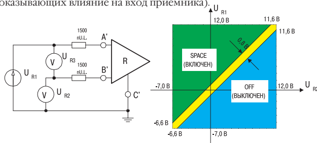
Рис. 8. Схема проверки степени симметрии входа приемника
