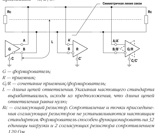
Рис. 1. Многоточечная система связи
