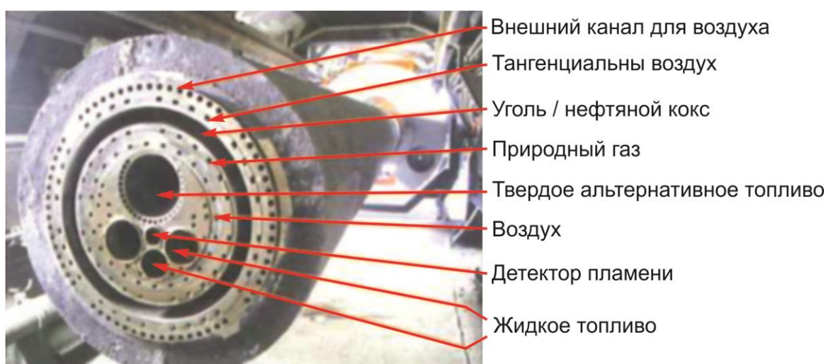
Рисунок 2.33 — Многоканальная горелка Flexiflame компании GRECO
