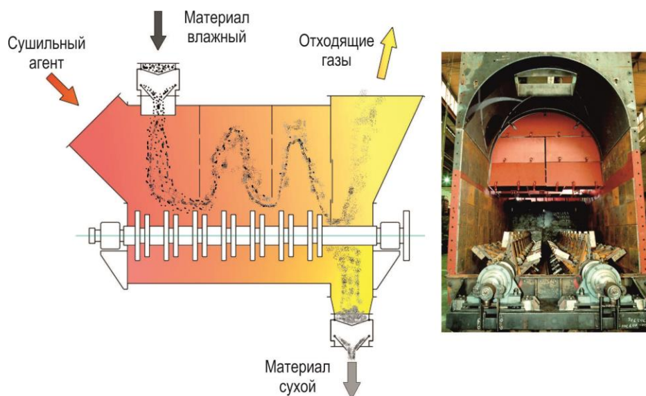
Рисунок 2.68 — Высокоскоростная сушилка фирмы HAZEMAG
