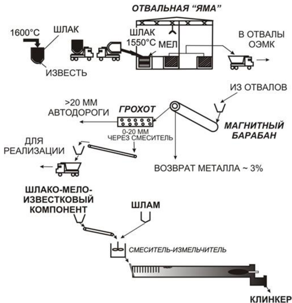
Рисунок 7.6 — Предлагаемая технологическая схема применения шлака
