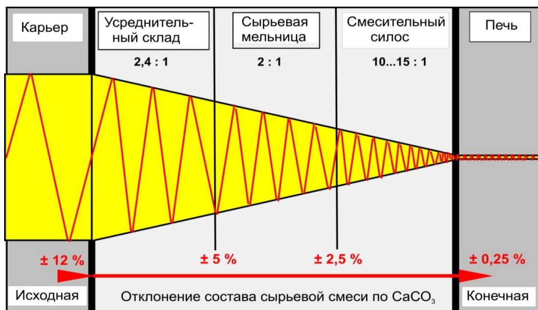
Рисунок 2.19 — Степень усреднения сырья на различных технологических переделах
