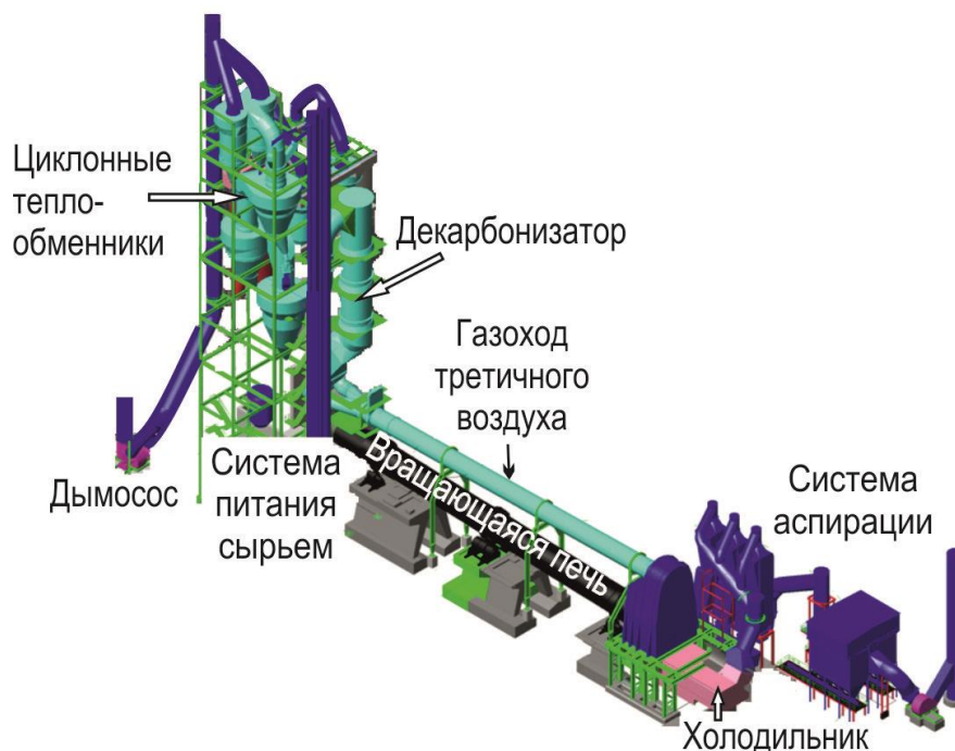
Рисунок 2.50 — Современная печная система с декарбонизатором
