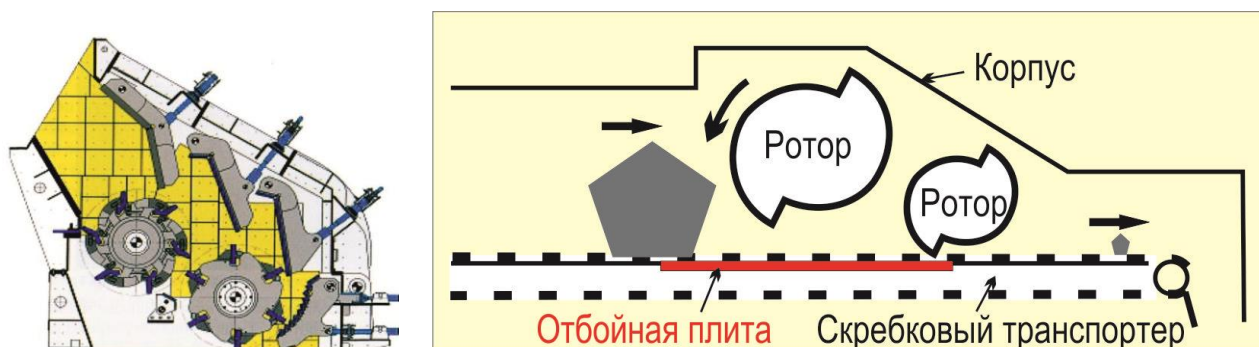
Рисунок 2.10 — Комбинированные двухроторные ударно- и валково-отражательные дробилки
