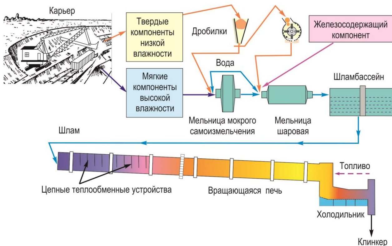
Рисунок 2.2 — Технологическая схема мокрого способа производства
