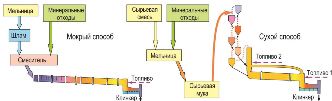
Рисунок 2.35 — Рациональные схемы применения минеральных отходов при различных способах производства клинкера
