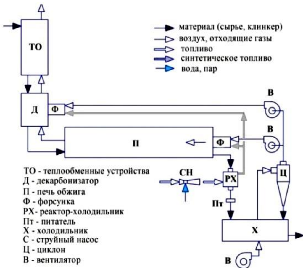
Рисунок 7.3 — Схема реализации метода химической регенерации теплоты клинкера
