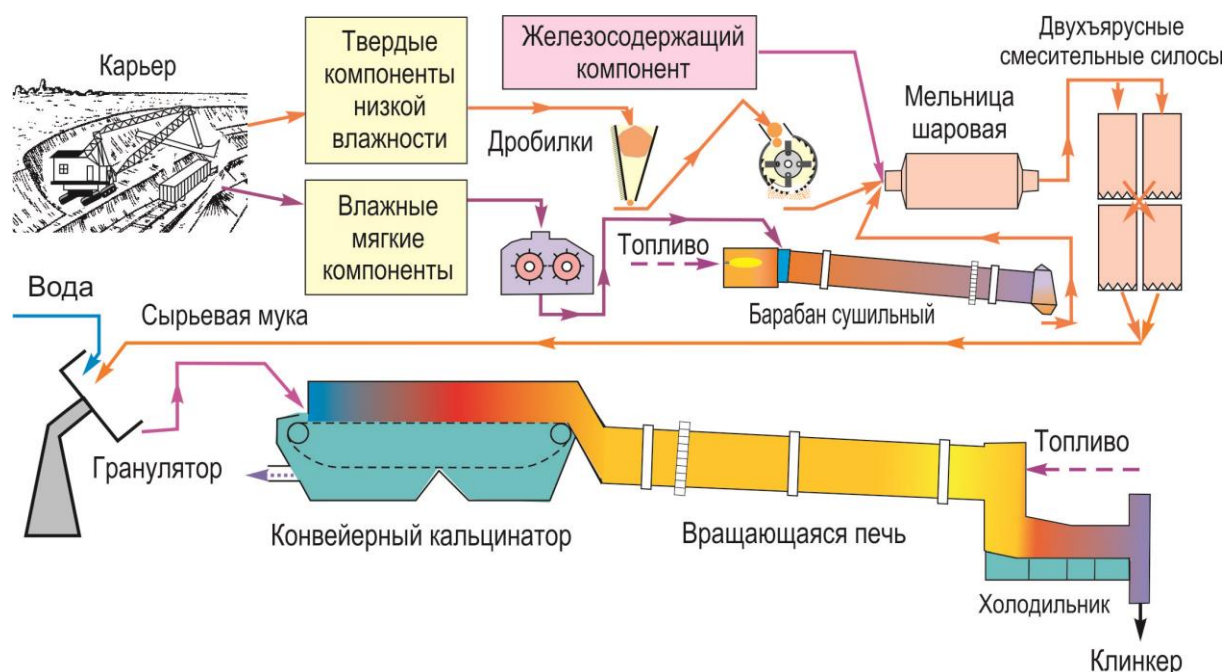
Рисунок 2.3 — Технологическая схема полусухого способа производства
