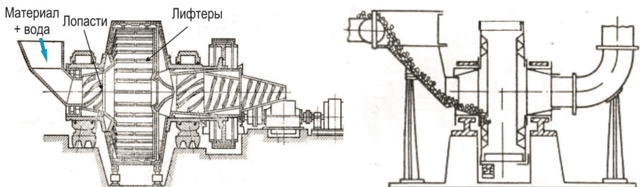
Рисунок 2.9 — Мельницы самоизмельчения мокрого и сухого способов производства
