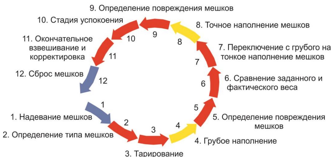
Рисунок 2.74 — Последовательность операций тарирования цемента упаковочной машиной
