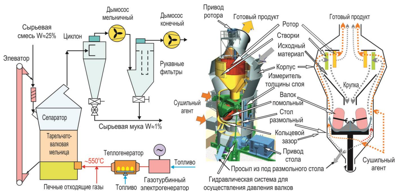
Рисунок 2.14 — Схема помола сырья с вертикальной тарельчато-валковой мельницей
