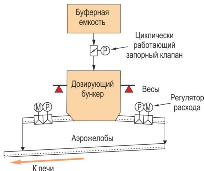
Рисунок 2.48 — Система питания печной системы материалом с дозирующим бункером
