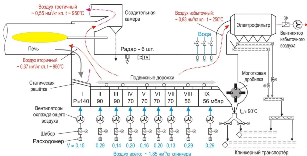
Рисунок 2.57 — Принципиальная схема клинкерного холодильника PYROFLOOR
