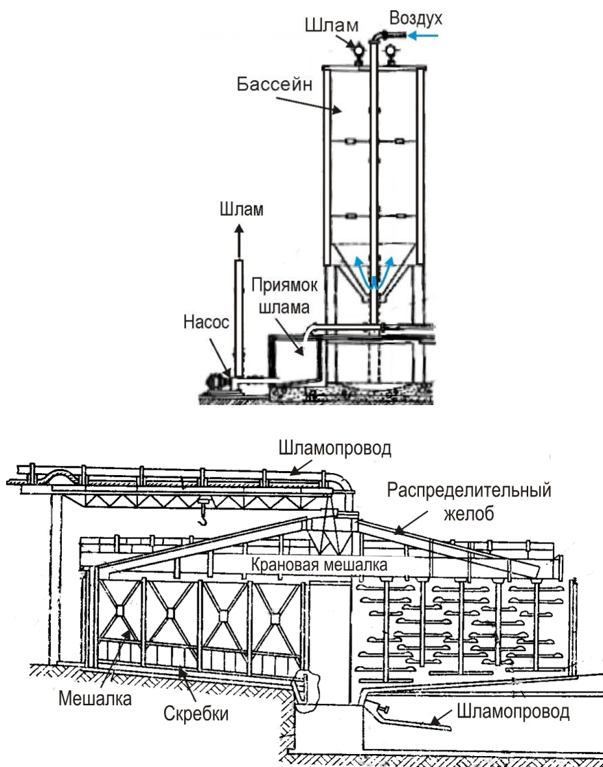
Рисунок 2.17 — Вертикальный и горизонтальный шламбассейны
