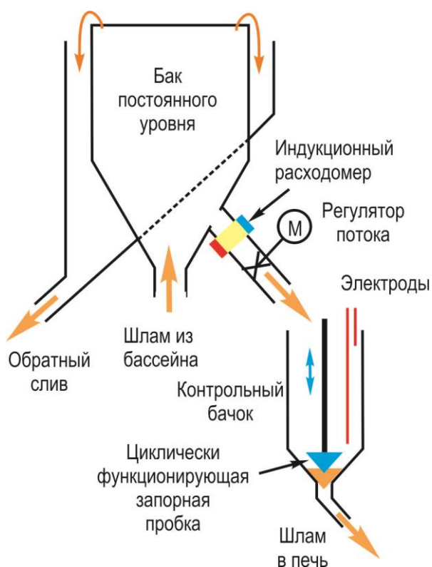
Рисунок 2.46 — Самоочищающийся питатель шлама
