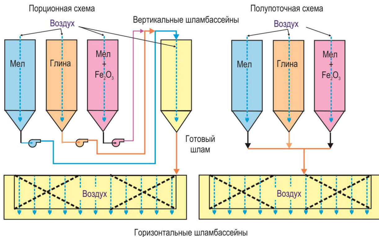
Рисунок 2.16 — Порционный и полупоточный способы корректирования шлама
