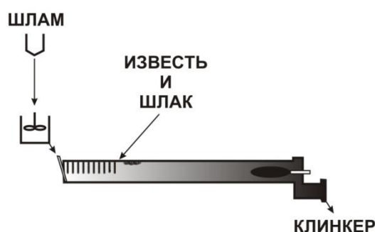
Рисунок 7.9 — Подача извести и шлака за цепную завесу
