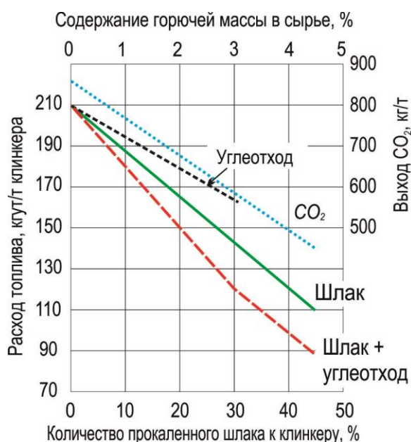
Рисунок 2.39 — Эффективность применения минеральных и горючих техногенных материалов
