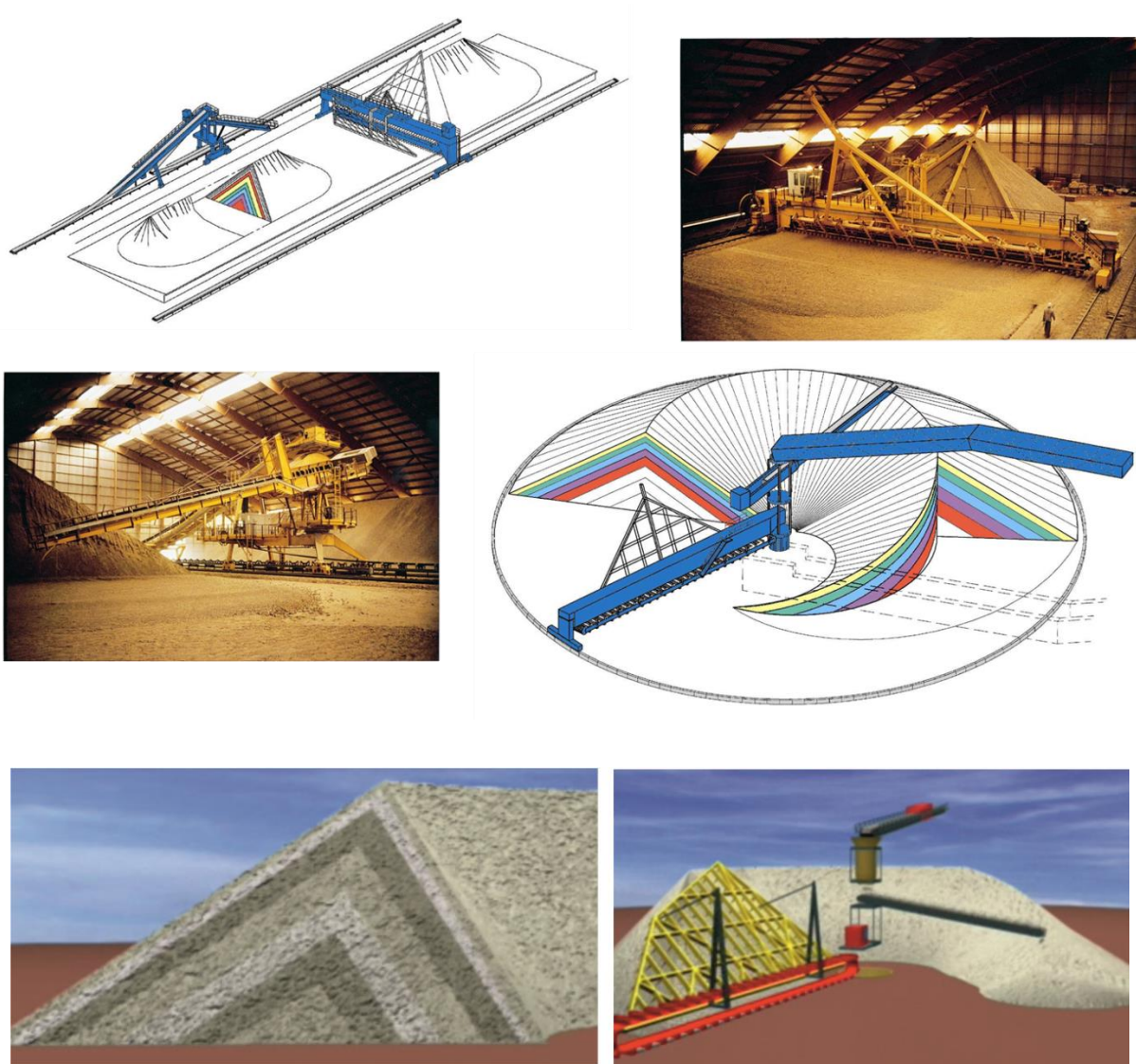
Рисунок 2.11— Усреднительный склад сырьевых компонентов фирмы Claudius Peters
