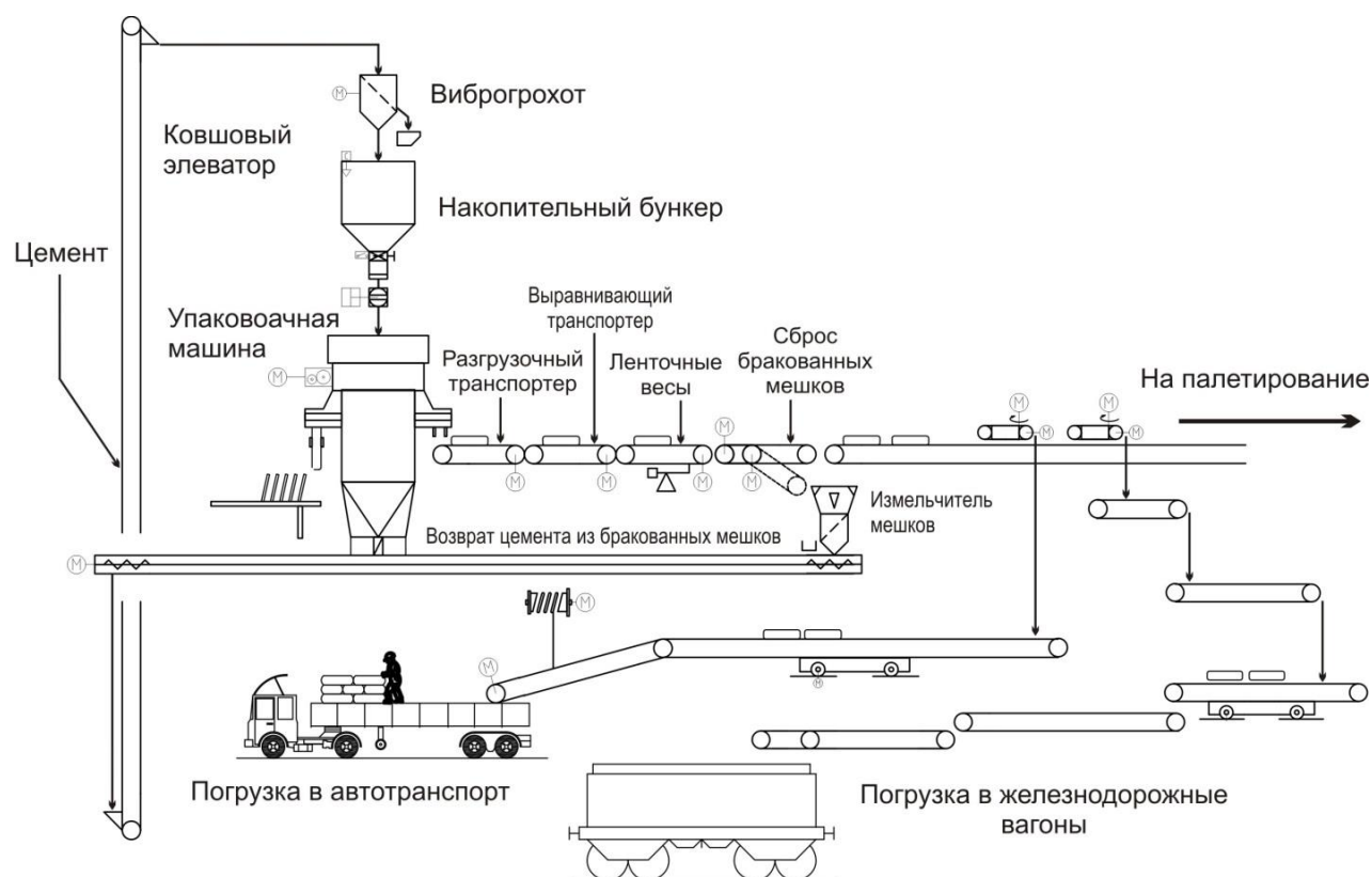
Рисунок 2.71 — Схема хранения и отгрузки цемента
