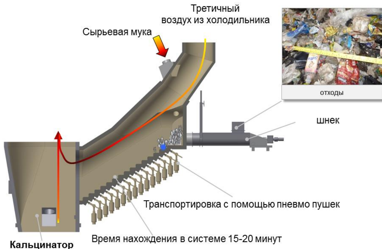
Рисунок 2.43 — Ступенчатая камера сгорания PREPOL
