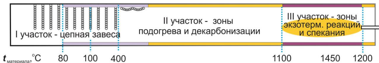
Рисунок 2.52 — Футеровка вращающейся печи мокрого способа производства
