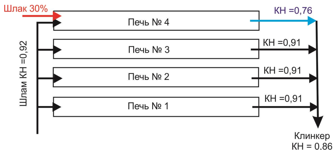
Рисунок 7.2 — Схема получения СДКЦ на одном составе шлама
