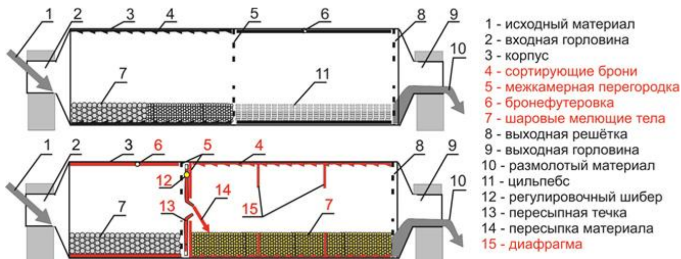
Рисунок 2.62 — Модернизация шаровой мельницы
