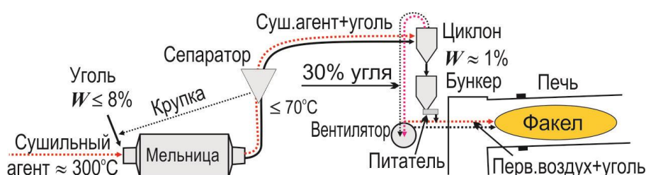
Рисунок 2.24 — Объединенная с печью система подготовки угля
