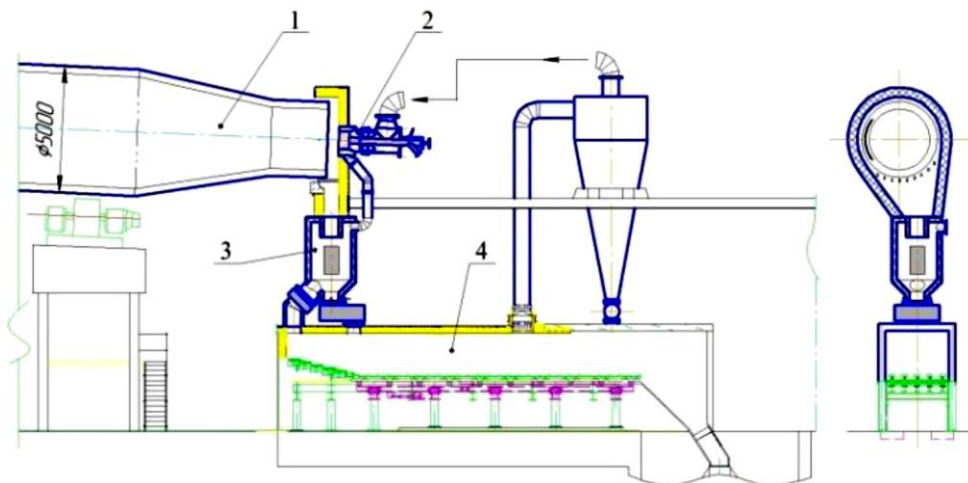
Рисунок 7.4 — Схема технической реализации метода ХРТ
