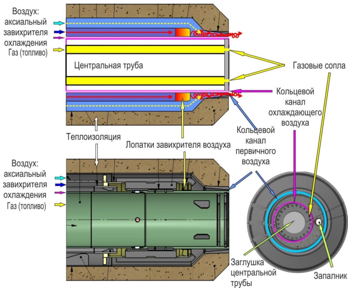
Рисунок 2.30 — Устройство и принцип работы горелки Duoflex фирмы FLSmith
