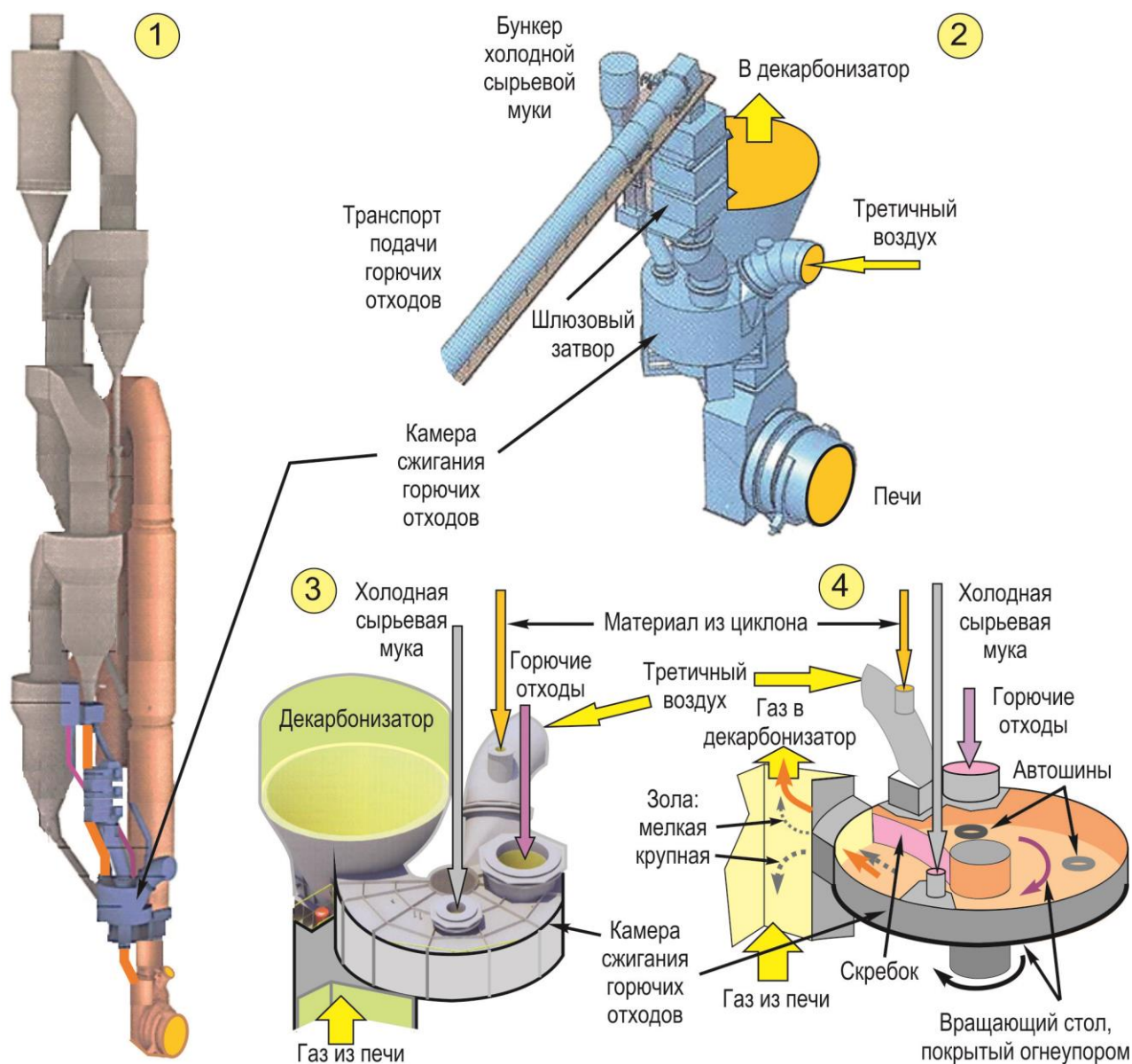
Рисунок 2.42 — Камера сгорания HOTDISC фирмы FLSmidth
