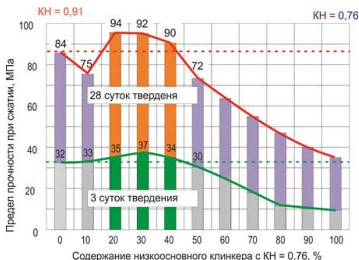
Рисунок 7.1 — Прочность при сжатии смешанного двухклинкерного цемента СДКЦ можно получить:
