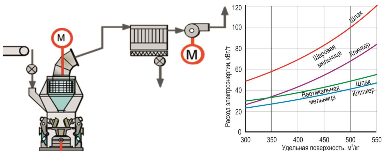
Рисунок 2.64 — Эффективность вертикальной валковой мельницы в сравнение с шаровой по данным фирмы Loesche
