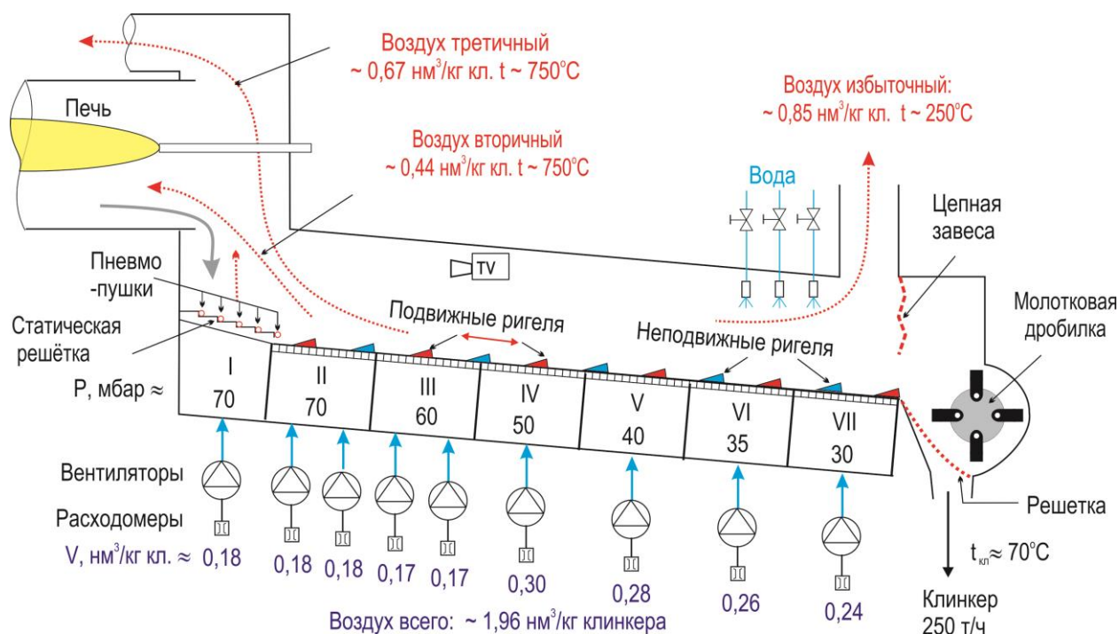
Рисунок 2.54 — Клинкерный ригельный холодильник фирмы FLSmidth
