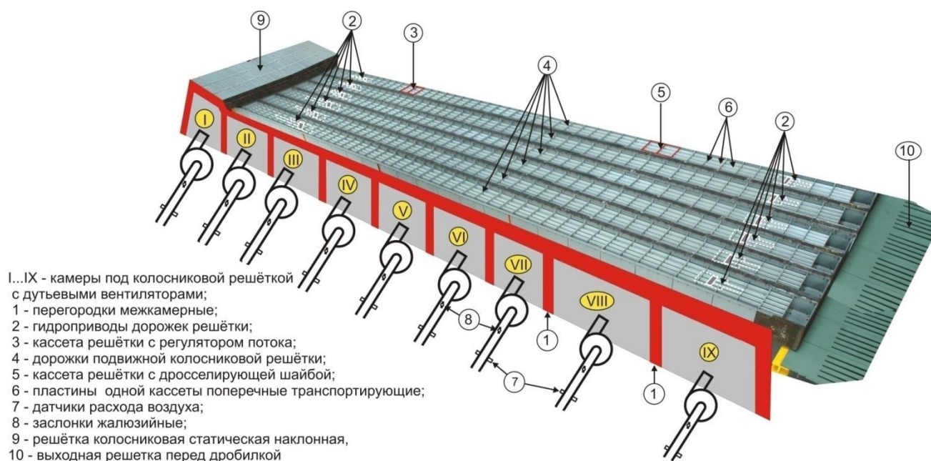
Рисунок 2.58 — Схема колосниковой решетки холодильника PYROFLOOR
