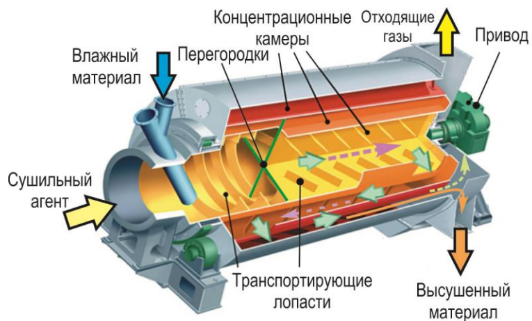
Рисунок 2.69 — Трехходовая барабанная сушилка фирмы GEBR. PFEIFFER
