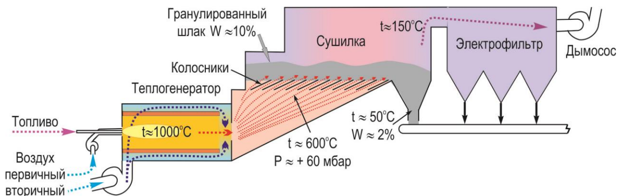
Рисунок 2.67 — Сушилка взвешенного слоя
