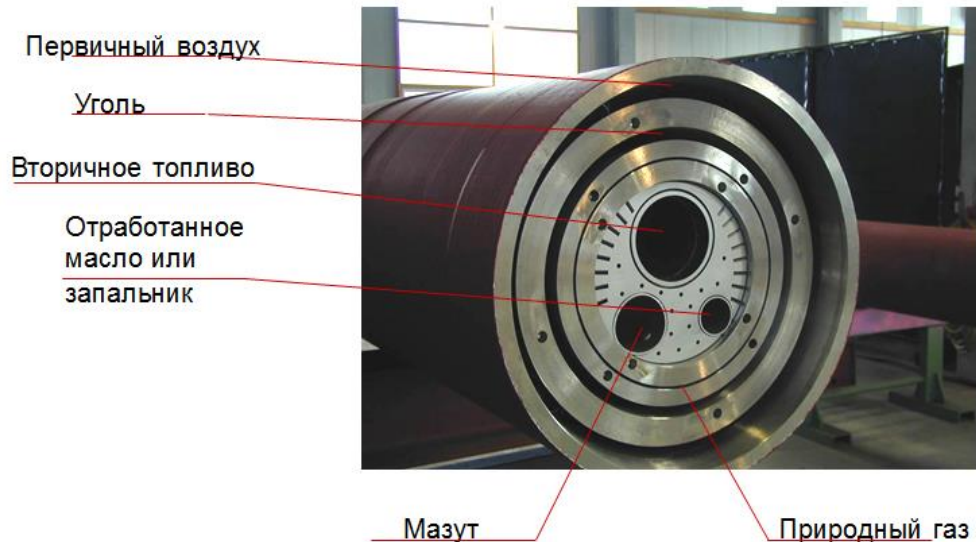
Рисунок 2.31 — Многоканальная горелка Unitherm компании Cemcon
