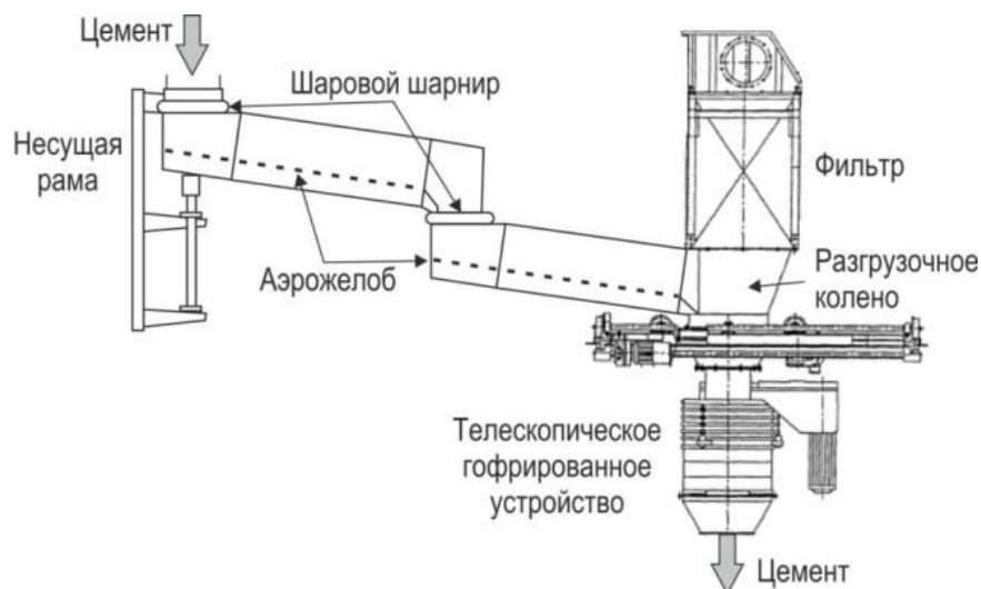
Рисунок 2.73 — Устройство для погрузки цемента навалом (FLSmidt)
