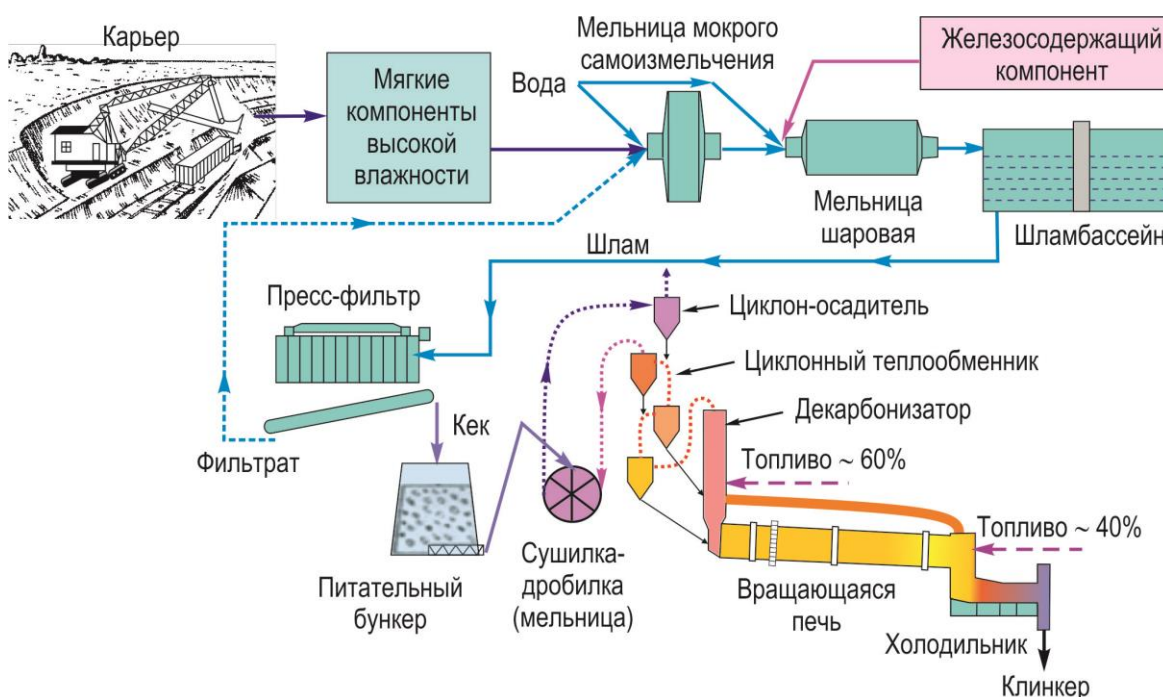
Рисунок 2.4 — Технологическая схема комбинированного способа производства
