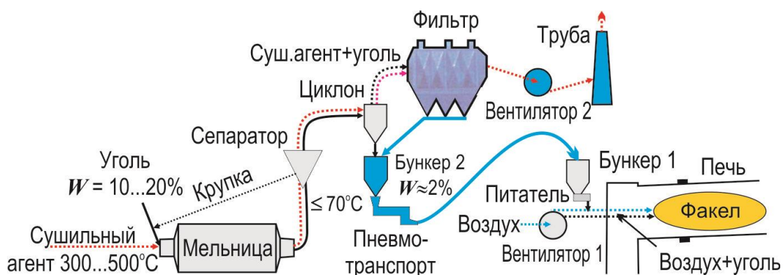
Рисунок 2.25 — Разъединенная с печью система подготовки угля
