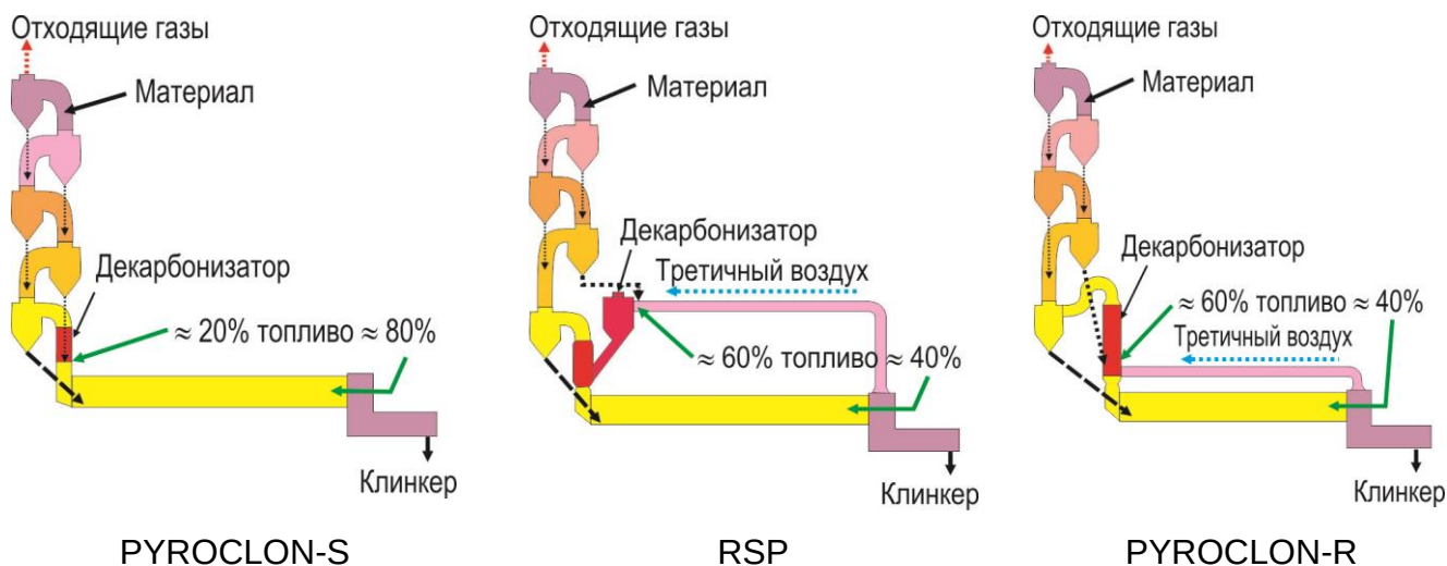
Рисунок 2.51 — Применяемые в России системы печей с декарбонизаторами
