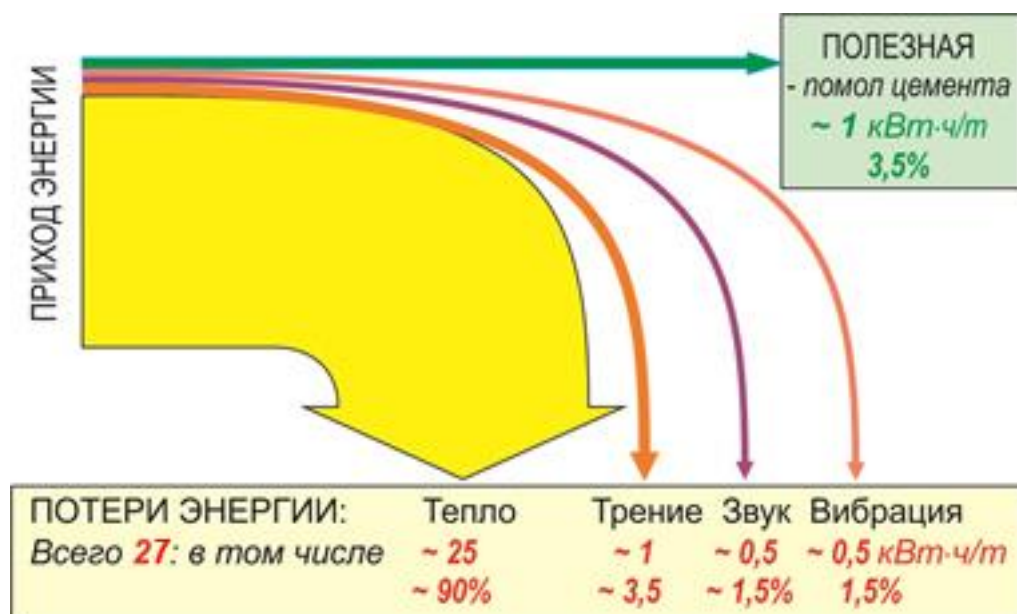
Рисунок 2.61 — Затраты энергии на отдельные процессы при помол цемента в шаровой мельнице по данным фирмы Christian Pfeiffer
