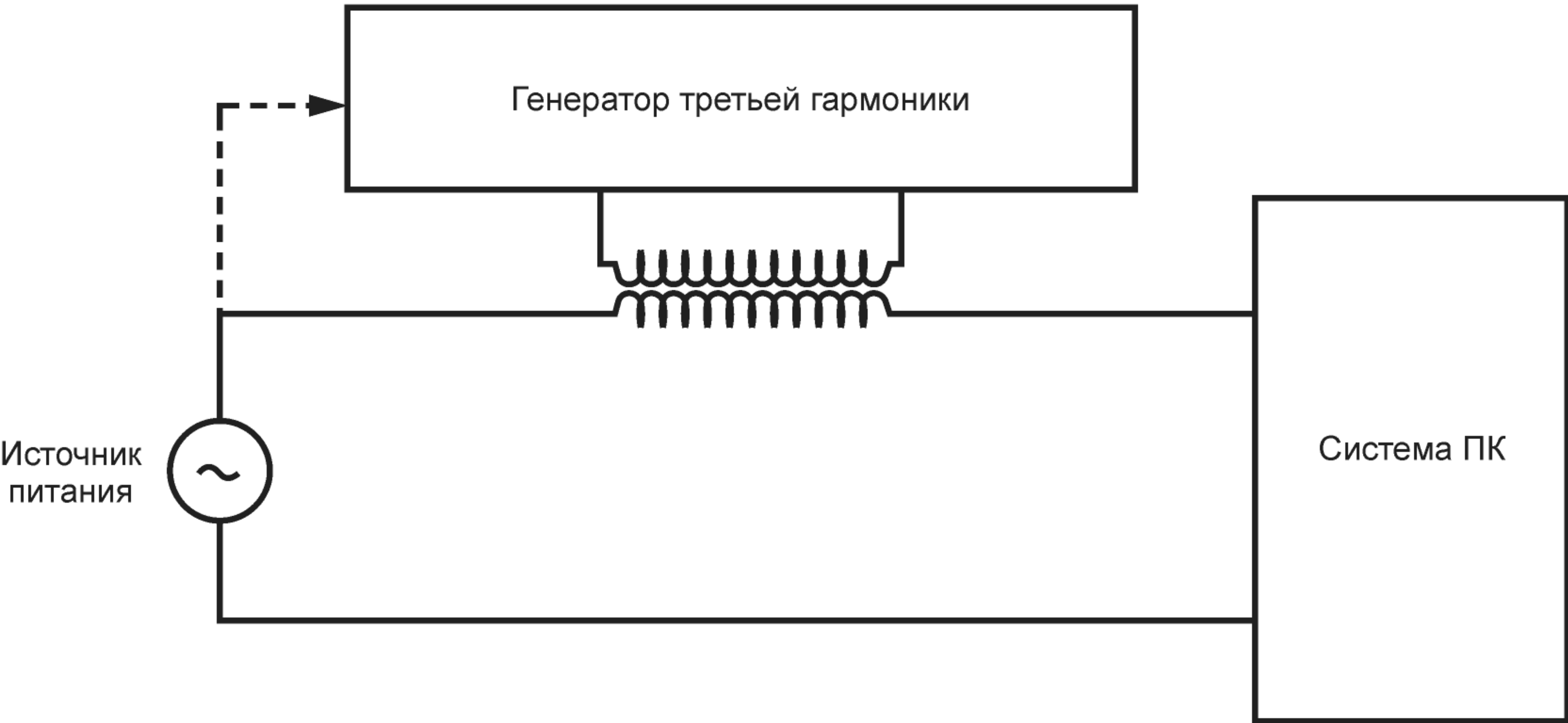
Рисунок 7 — Испытание на устойчивость к напряжению третьей гармоники
