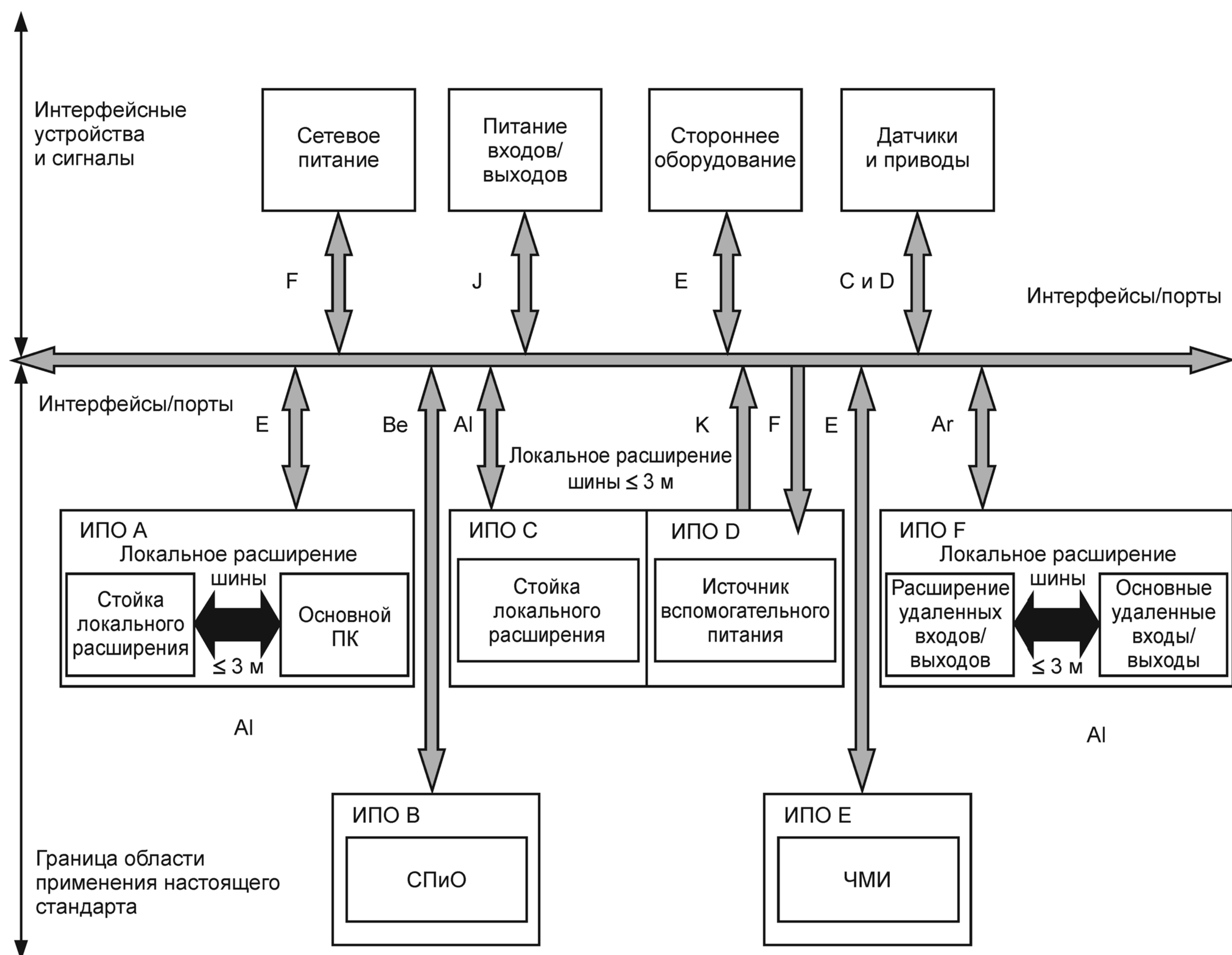
Рисунок 1 — Конфигурации испытываемого оборудования
