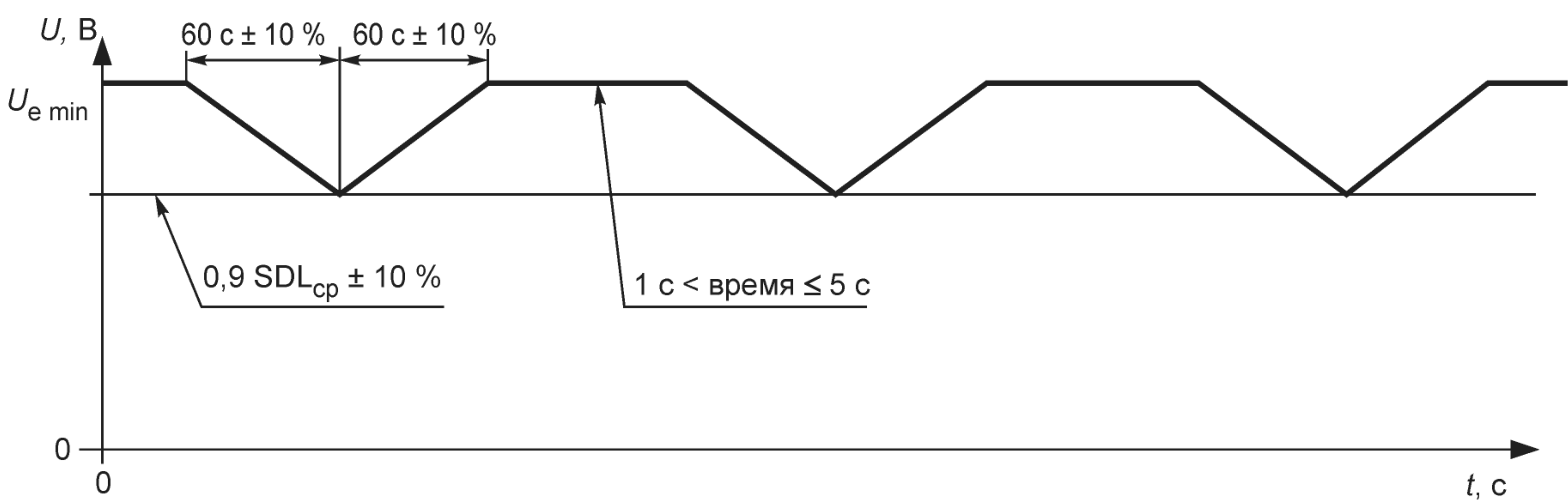
Рисунок 10 — Испытание на медленное изменение напряжения питания
