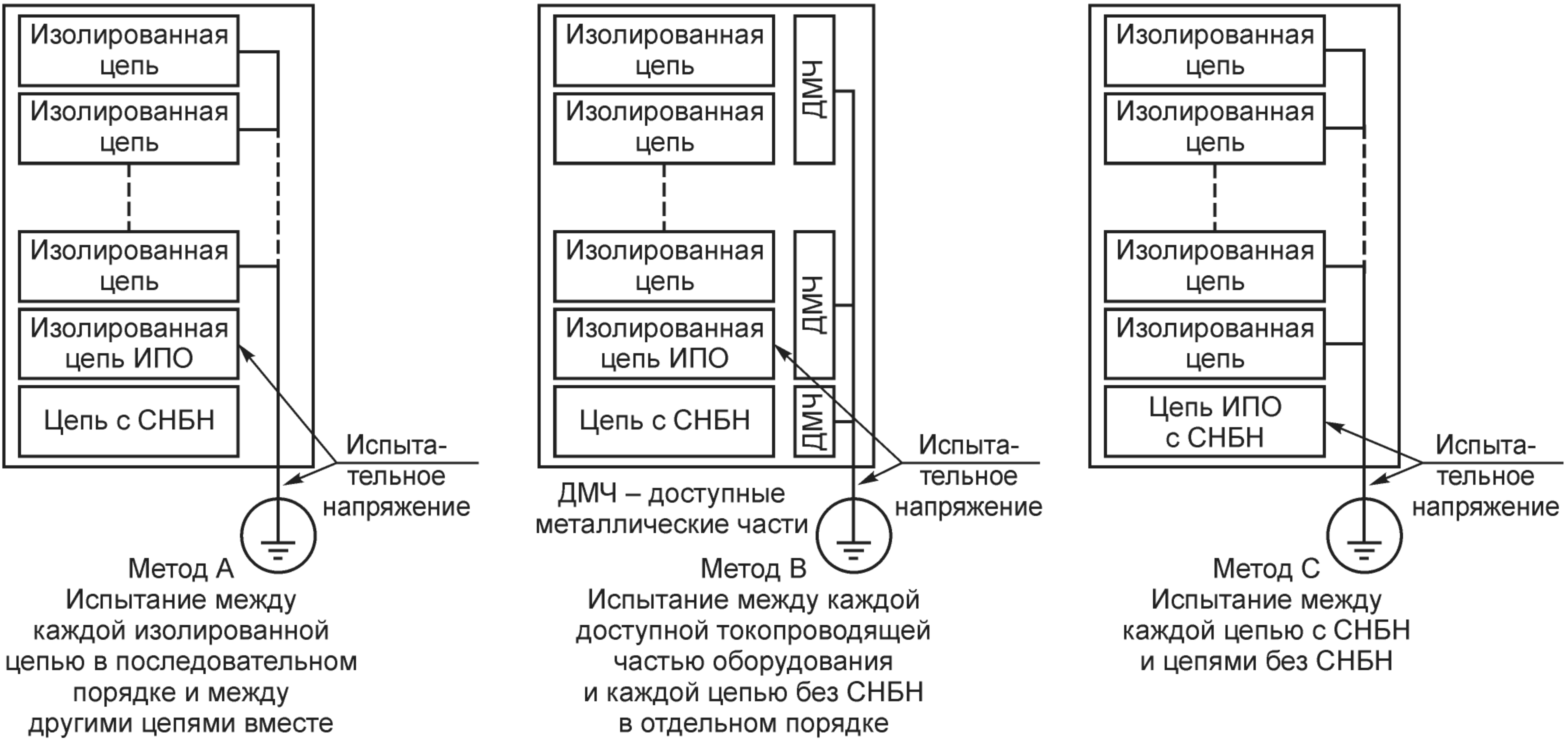
Рисунок 13 — Методы испытания на электрическую прочность диэлектрика
