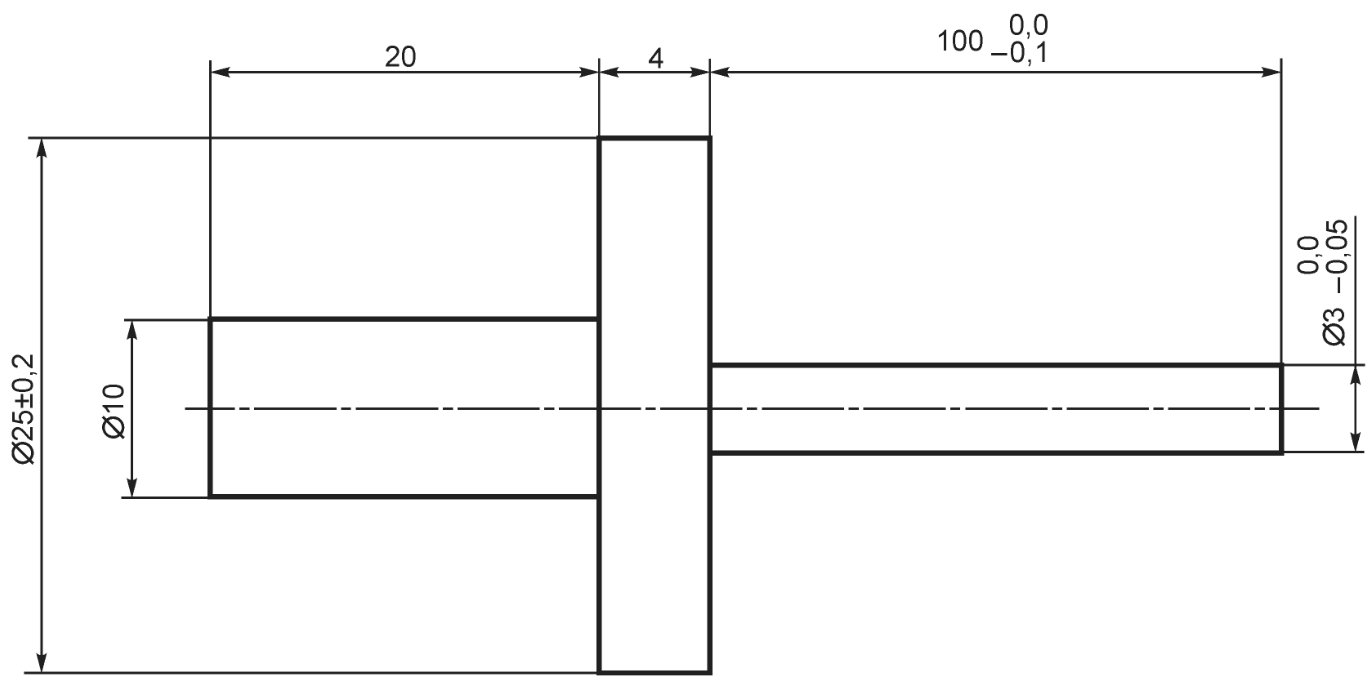
Рисунок С.4 — Испытательный штифт 100 × 3 мм
