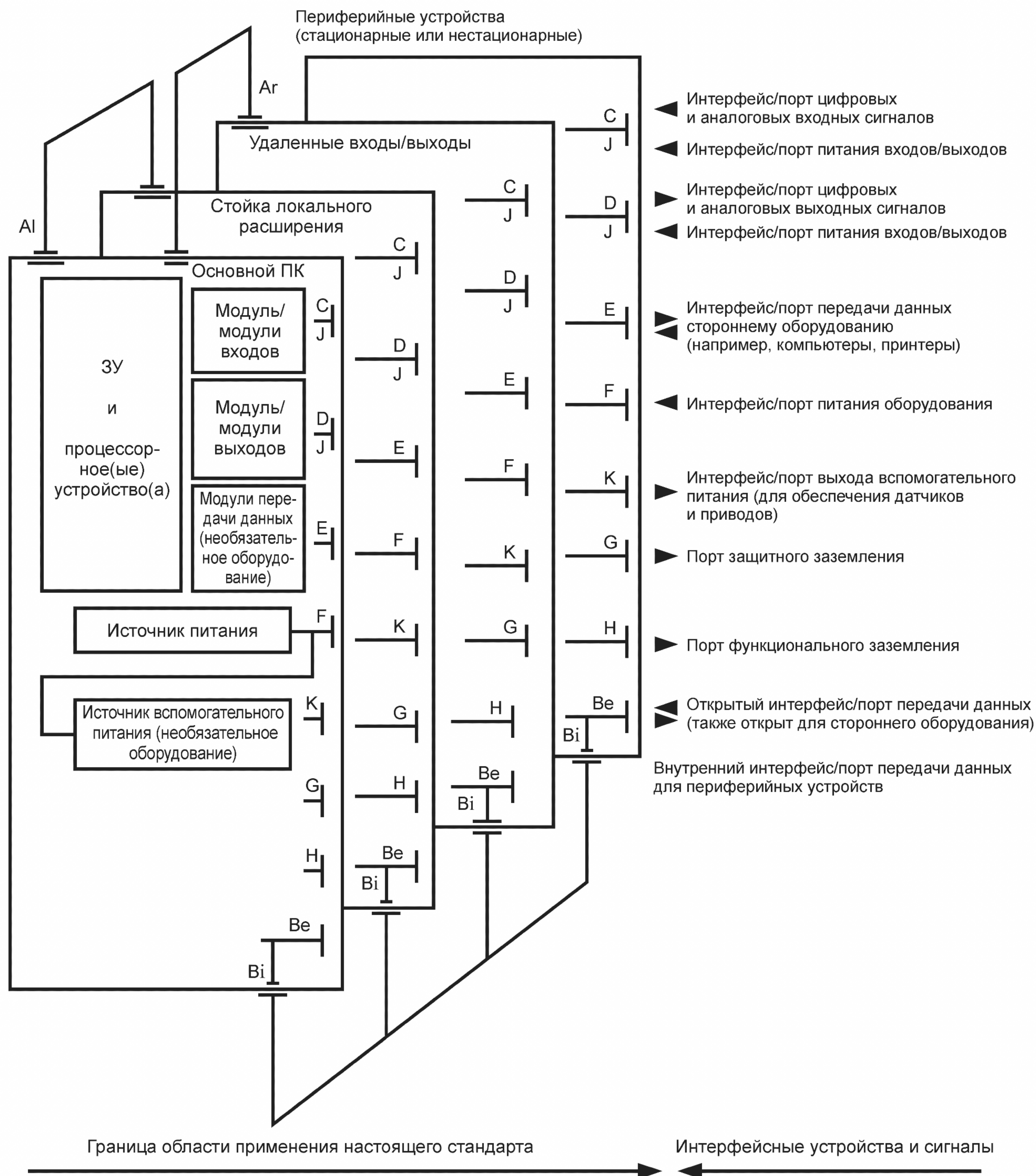
Рисунок 2 — Типовая конфигурация интерфейсов/портов системы ПК
