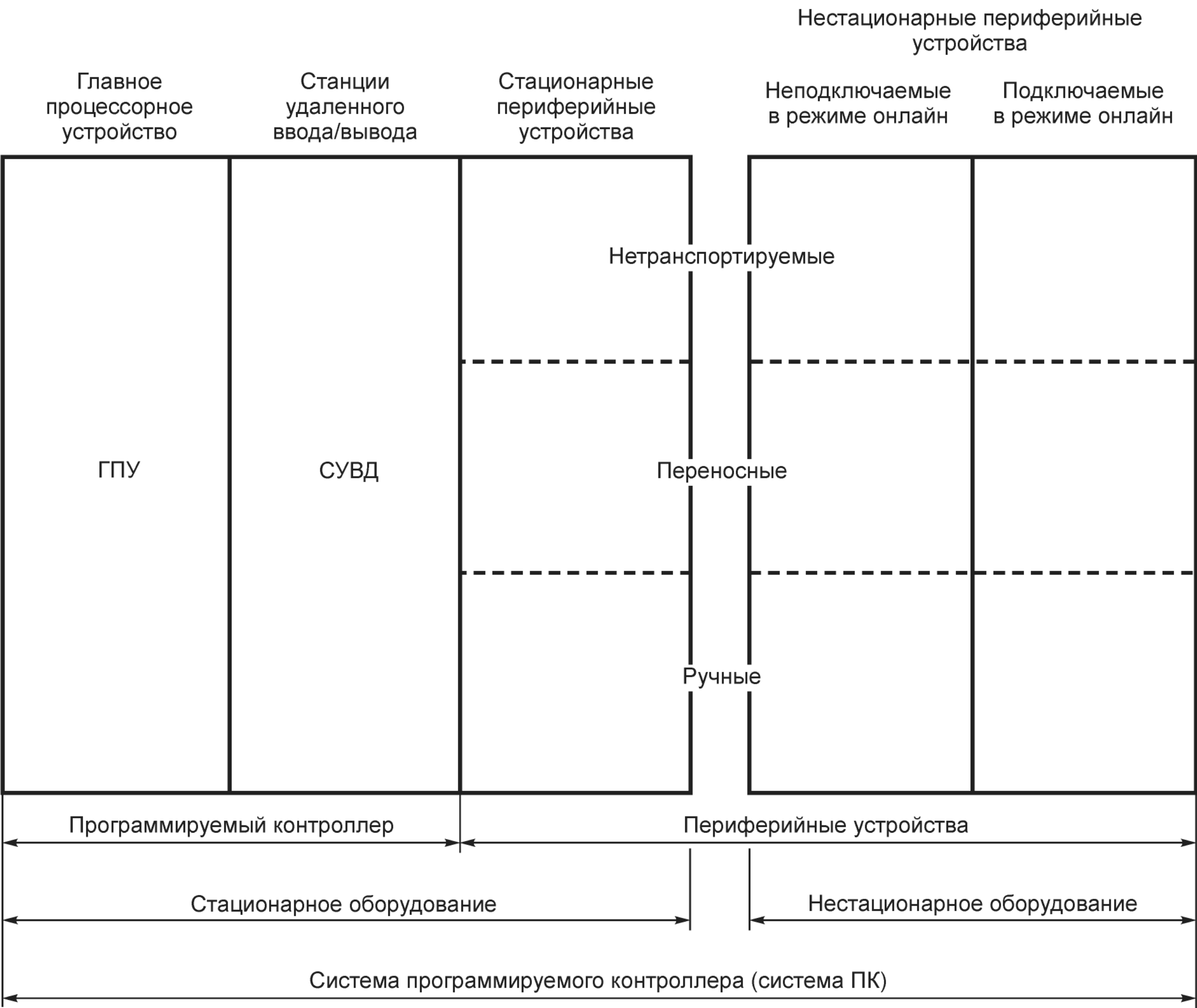
Рисунок А.1 — Система программируемого контроллера (система ПК)
