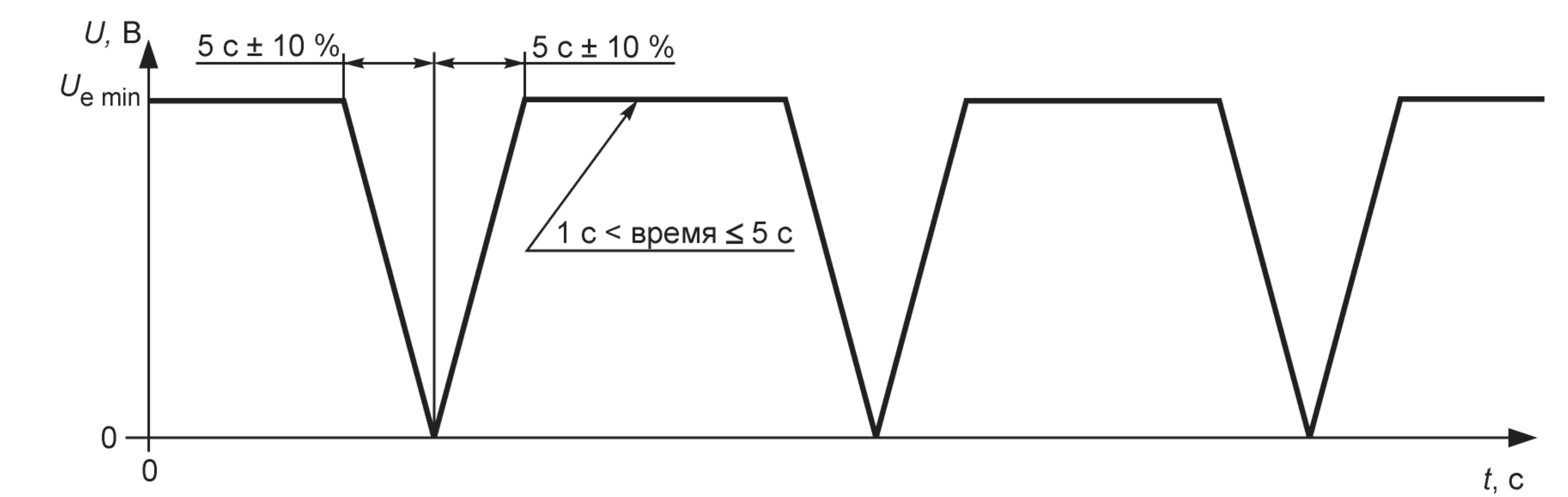
Рисунок 9 — Испытание на быстрое изменение напряжения питания
