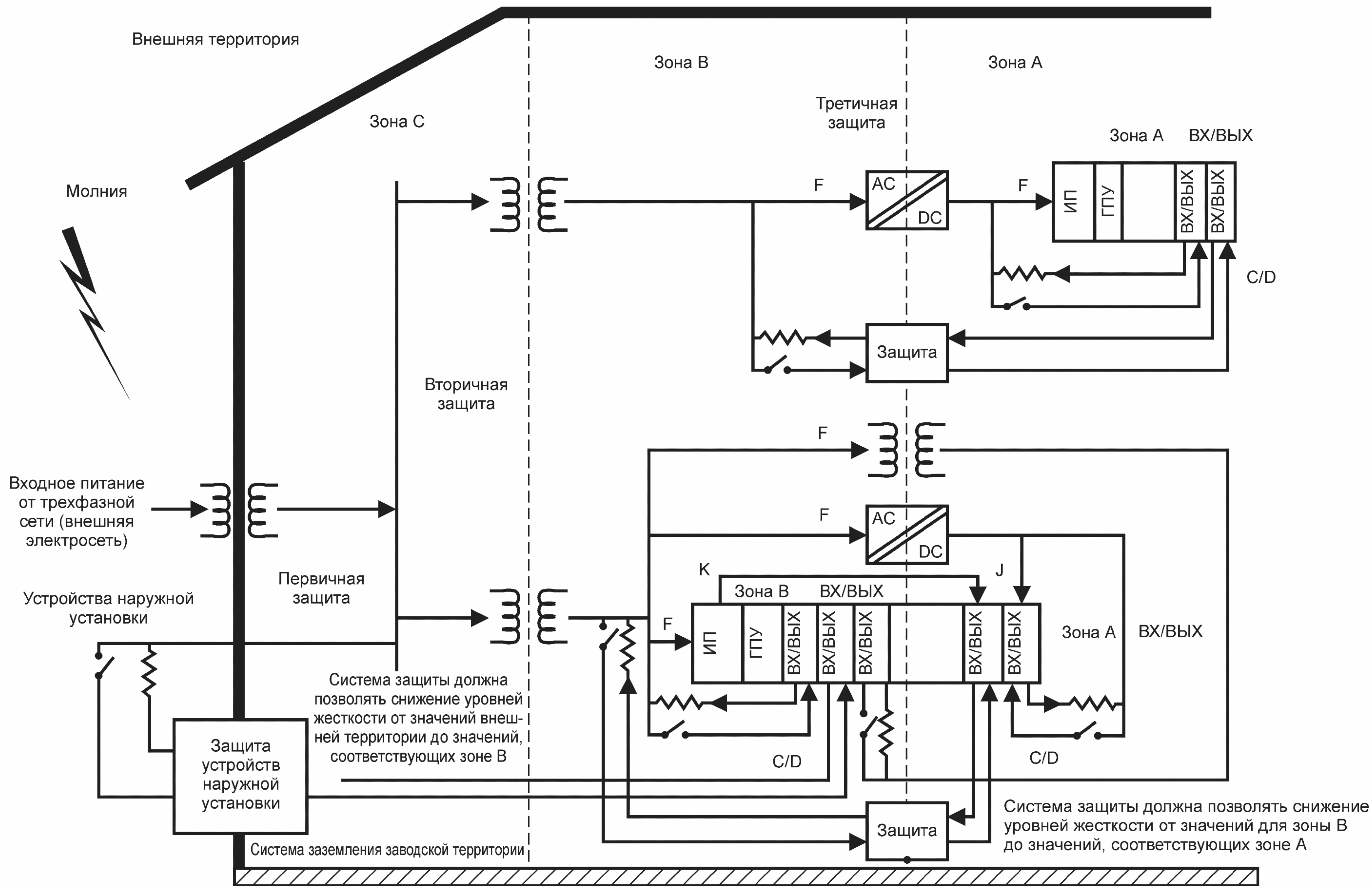
Рисунок 11 — Зоны устойчивости к электромагнитным помехам
