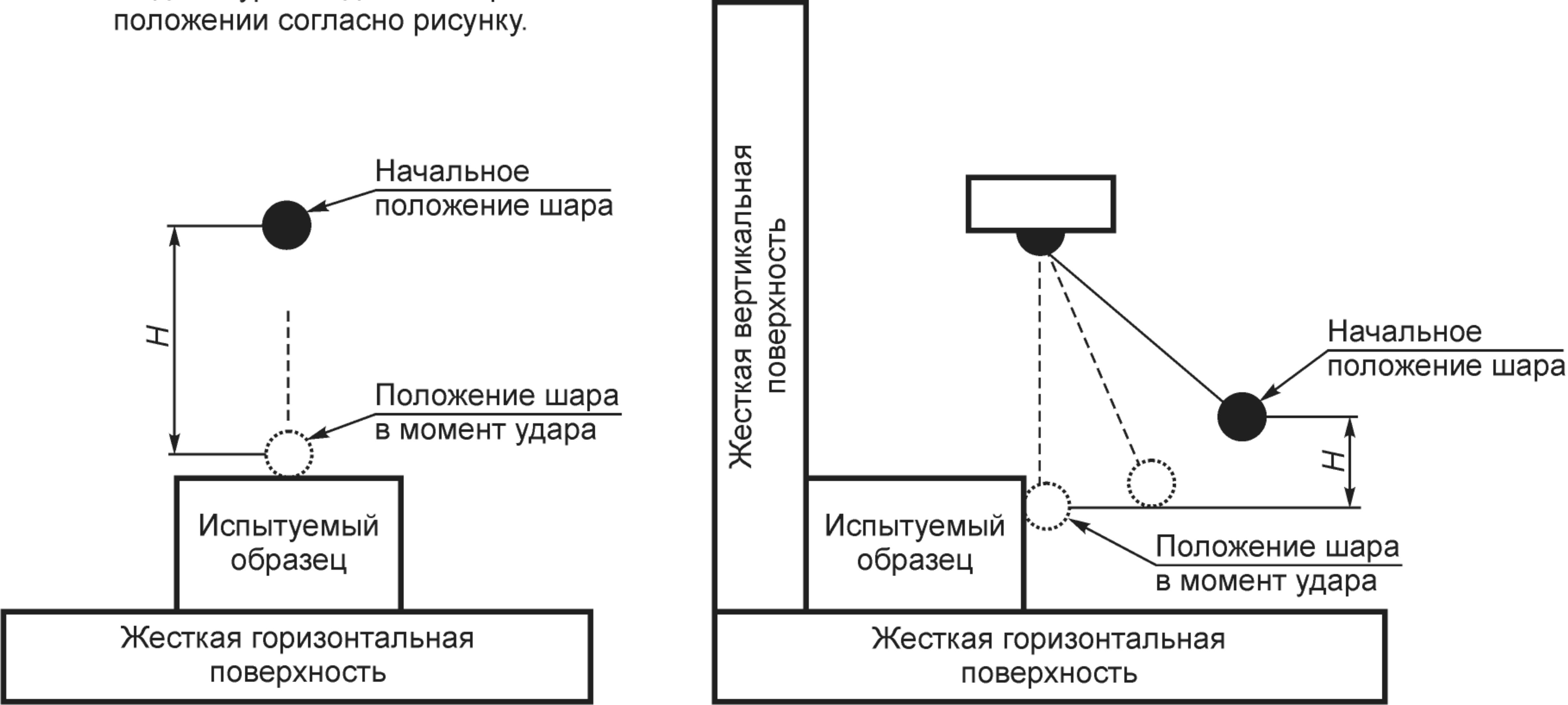
Рисунок 12 — Метод испытаний на ударостойкость
