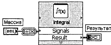
Рис. 2.6. Блок-диаграмма подключения Экспресс-ВП
