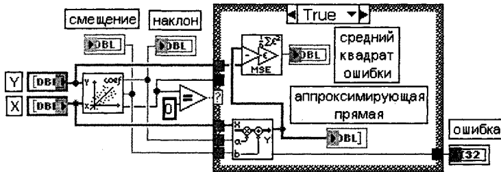
Рис. 3.41. Блок-диаграмма ВП Линейная аппроксимация (Linear Fit)
