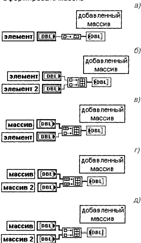
Рис. 2.24. Варианты подключения функции Сформировать массив
