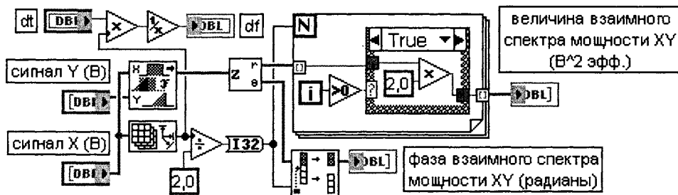
Рис 3.15. Блок-диаграмма ВП Взаимный спектр мощности (Cross Power Spectrum)
