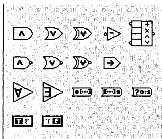
Рис. 2.8 Вид палитры логических функций
