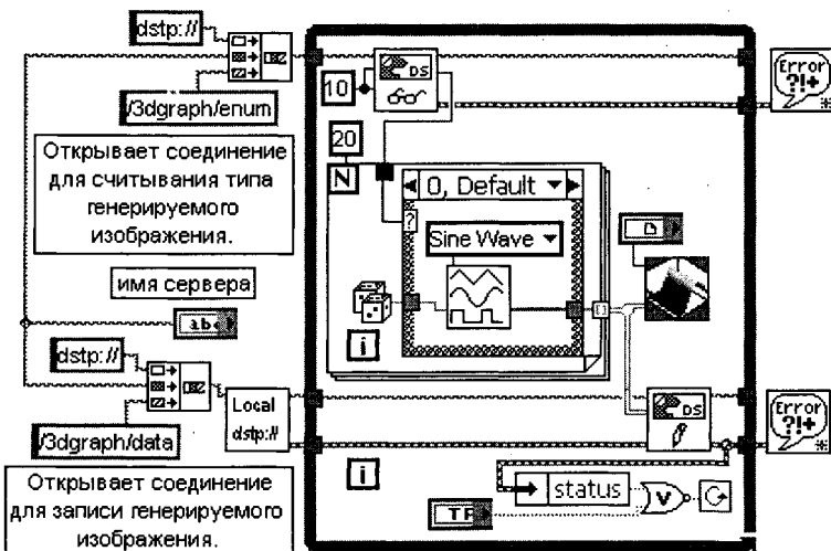
Рис. 4.22. Блок-диаграмма ВП Устройство записи данных трехмерного графика в соединение DataSocket (DS 3D Graph Writer)
