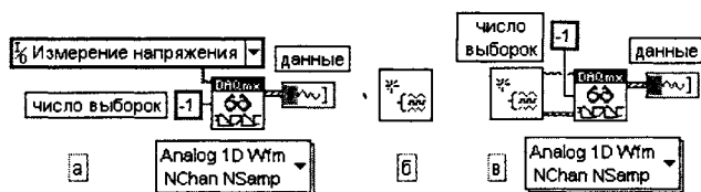
Рис. 5.29. Варианты кода ВП измерения напряжения
