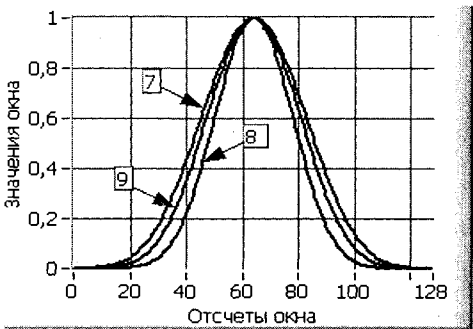
Рис. 3 29 Весовые окна Четырехзвенное Блэкмана-Хэрриса (7), Семизвенное Блэкмана-Хэрриса (8), Low Sidelobe (9)
