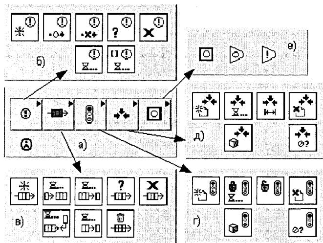
Рис. 3.58. Вид палитры (а) и подпалитр (б–е) функций и ВП синхронизации
