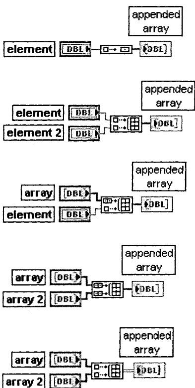
Рис. 2.24. Варианты подключения функции Сформировать массив
