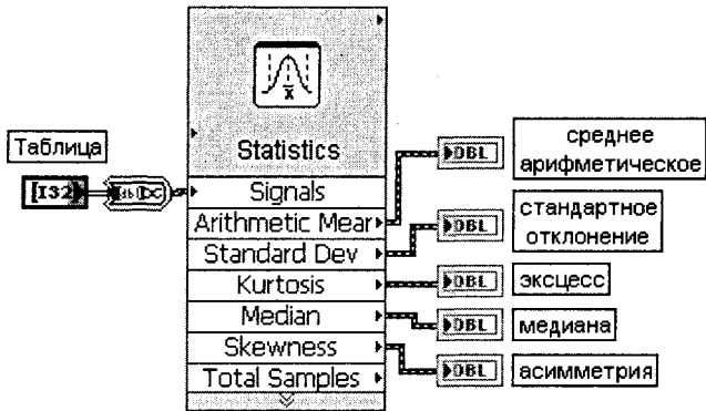
Рис. 3.36. Блок-диаграмма возможного подключения Экспресс-ВП
