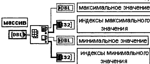
Рис 2.25. Варианты подключения функции Максимум и минимум массива
