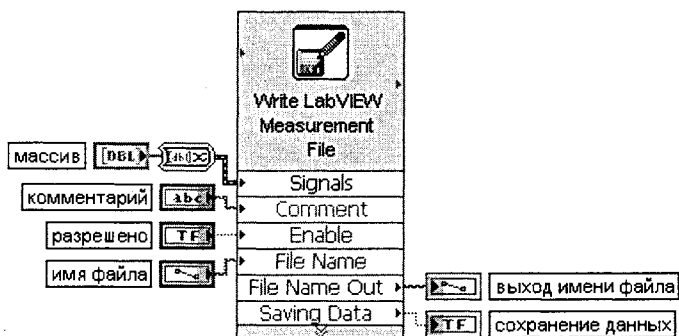
Рис. 2.40 Блок-диаграмма возможного подключения Экспресс-ВП
