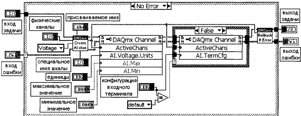
Рис. 5.32 Блок-диаграмма ВП Создать виртуальный канал DAQmx
