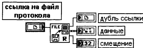
Рис. 2 37. Варианты подключения функции Считать файл (Read File)
