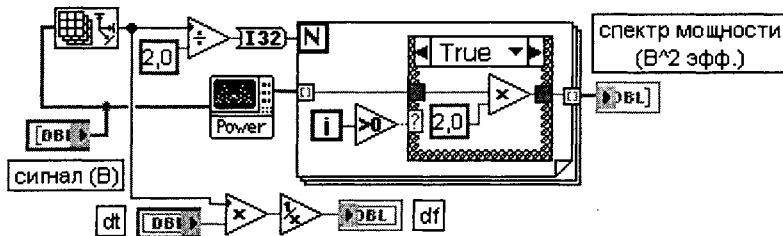
Рис. 3.14. Блок-диаграмма ВП Спектр мощности (Auto Power Spectrum)
