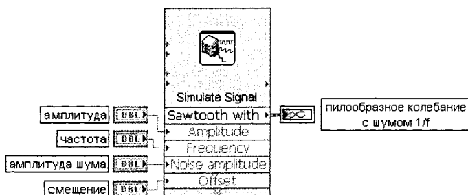
Рис. 5.19. Блок-диаграмма возможного подключения Экспресс-ВП
