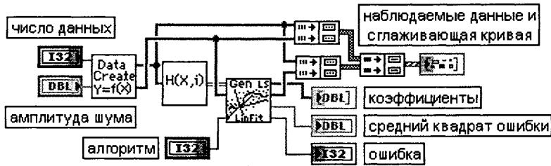
Рис. 3.44 Блок-диаграмма ВП
