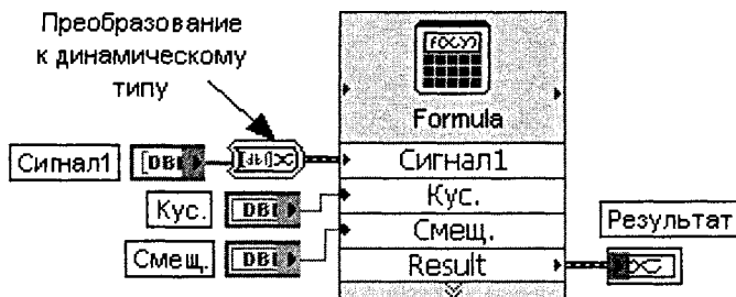
Рис. 2.3 Блок-диаграмма варианта подключения Экспресс-ВП
