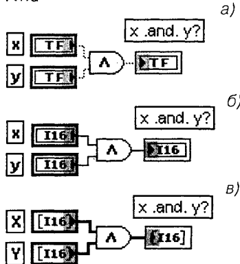
Рис. 2.9 Варианты подключения функции И
