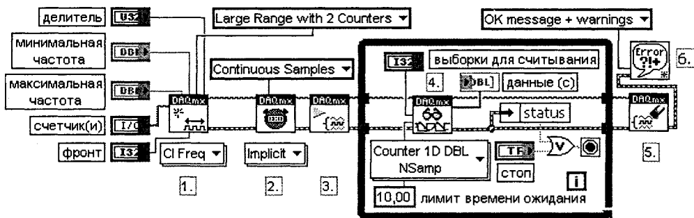
Рис 5.34 Блок-диаграмма ВП Meas Dig Freq-Buffered-Cont-Large Range 2
