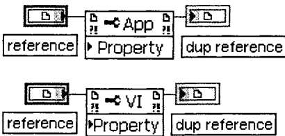
Рис 4 5. Варианты конфигурирования Узла свойства
