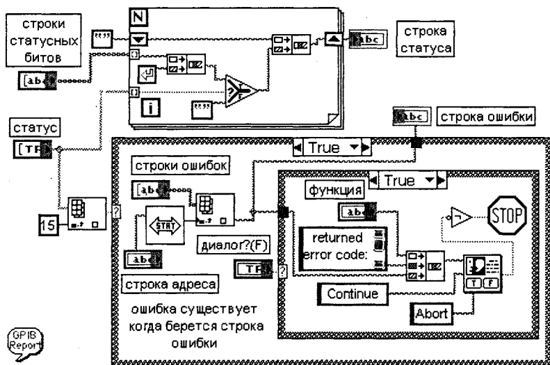
Рис. 5.38. Иконка и блок-диаграмма ВП Сообщение от ошибке GPIB (GPIB Error Report)
