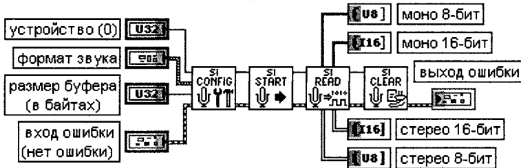
Рис. 3.66 Блок-диаграмма ВП Считать звуковую осциллограмму (Snd Read Waveform)
