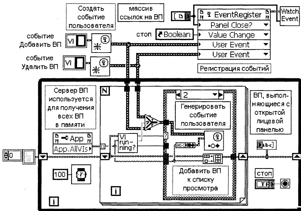
Рис. 4.12 Блок-диаграмма модернизированного ВП Динамическая проверка ВП
