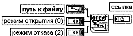
Рис. 2.38. Варианты подключения функции Открыть файл (Open File)
