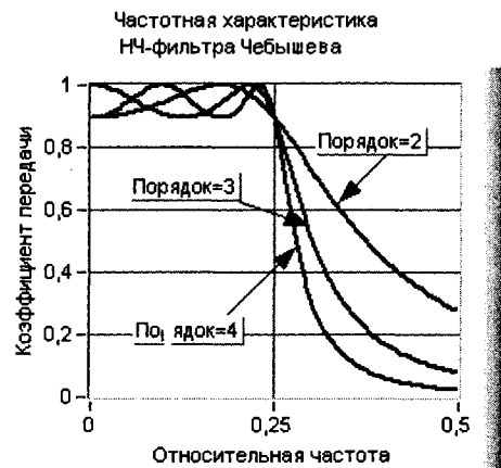
Рис. 3.20 Амплитудно-частотная характеристика фильтра Чебышева
