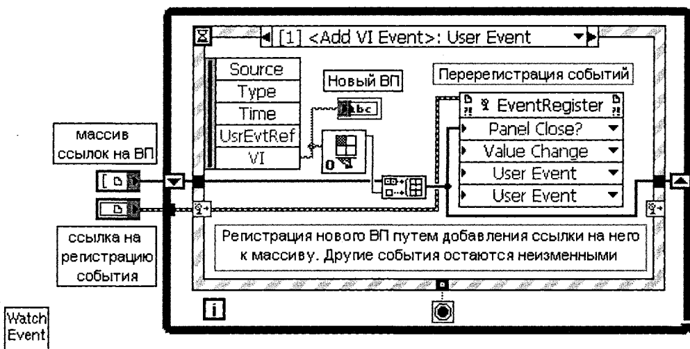
Рис. 4.14 Иконка и блок-диаграмма модернизированного подприбора Ожидать событий
