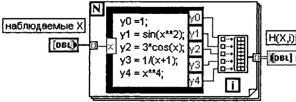
Рис. 3.47. Блок-диаграмма подпрограммы LinBasFns
