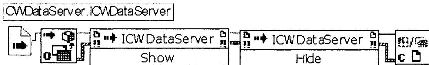
Рис. 4.19. Блок-диаграмма ВП программного вызова сервера DataSocket
