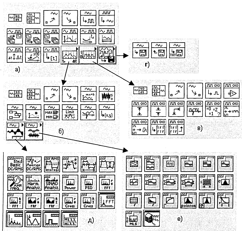
Рис. 5.4 Вид палитры (а) и дополнительных подпалитр (б–е) функций работы с осциллограммами
