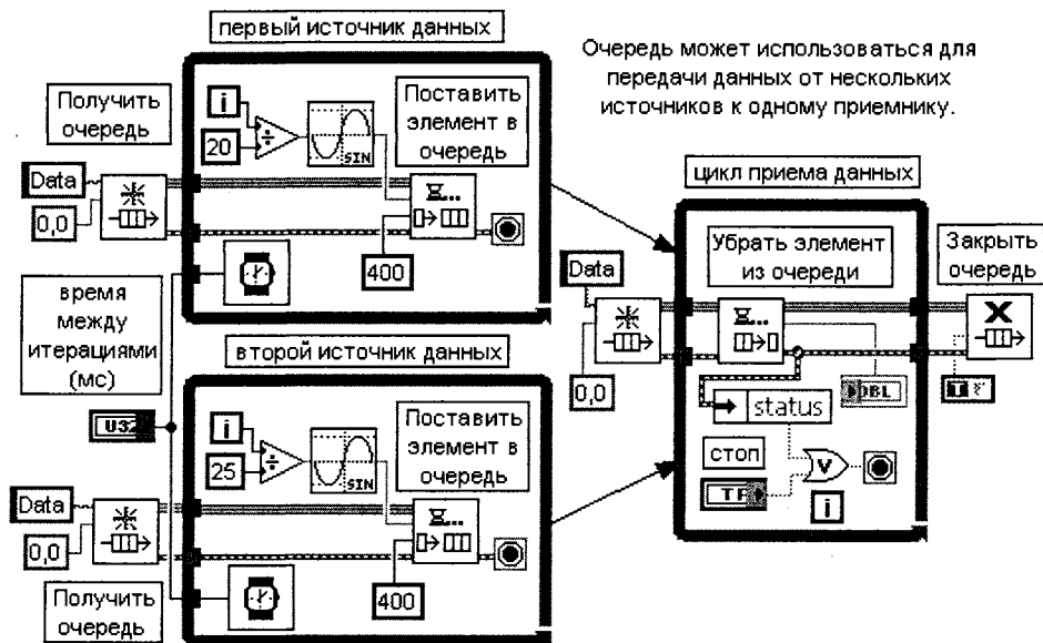
Рис 3 60. Блок-диаграмма ВП Очередь-мультиплексор (Queue Multiplexer)
