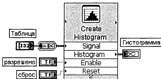
Рис. 3.38. Блок-диаграмма возможного подключения Экспресс-ВП
