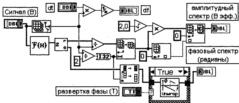
Рис. 3 13 Блок-диаграмма ВП Амплитудный и фазовый спектр (Amplitude and Phase Spectrum)
