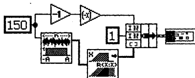
Рис. 3.3. Блок-диаграмма программы расчета автокорреляционной функции с центром в нулевой точке
