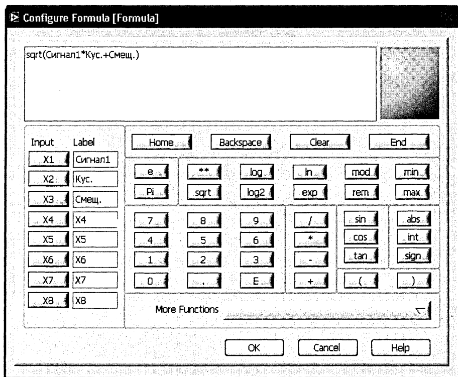
Рис. 2.4 Вид диалогового окна конфигурирования Экспресс-ВП Формула (Formula)
