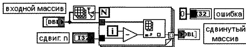
Рис. 3 5 Блок-диаграмма ВП Y[i]=X[i-n]
