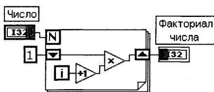
Рис. 1.8 Блок-диаграмма ВП вычисления факториала числа
