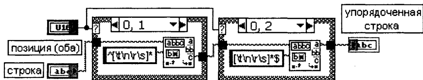
Рис. 2.14. Блок-диаграмма ВП Упорядочить пробелы (Trim Whitespace)
