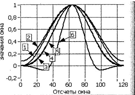
Рис. 3 28 Весовые окна Хана (1), Хэмминга (2), Блэкмана-Хэрриса (3), Точное Блэкмана (4), Блэкмана (5), Плосковершинное (6)
