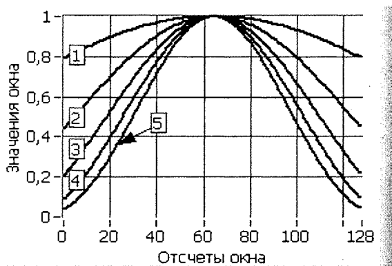
Рис 3 30 Графики окон Кайзера-Бесселя при \beta = 1 \div 5
