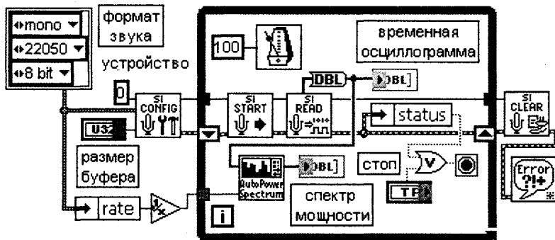
Рис. 3.69. Блок-диаграмма ВП Спектр мощности звуковой карты (Sound Card AutoPower Spectrum)
