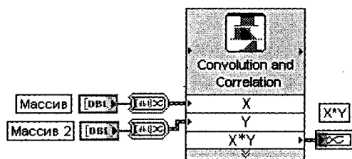
Рис. 3.10. Блок-диаграмма возможного подключения Экспресс-ВП
