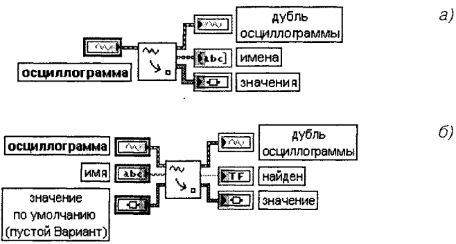
Рис 5.5 Варианты подключения функции Получить атрибуты осциллограммы
