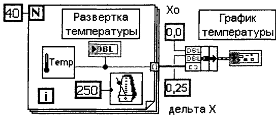
Рис. 1.17. Блок-диаграмма ВП контроля температуры с индикаторами Развертка температуры и График температуры
