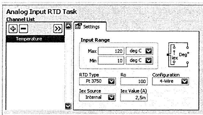
Рис 5.25. Вид раздела Установки диалогового окна настройки параметров физического канала
