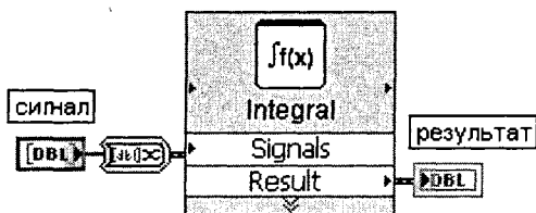
Рис. 3.32. Блок-диаграмма возможного подключения Экспресс-ВП
