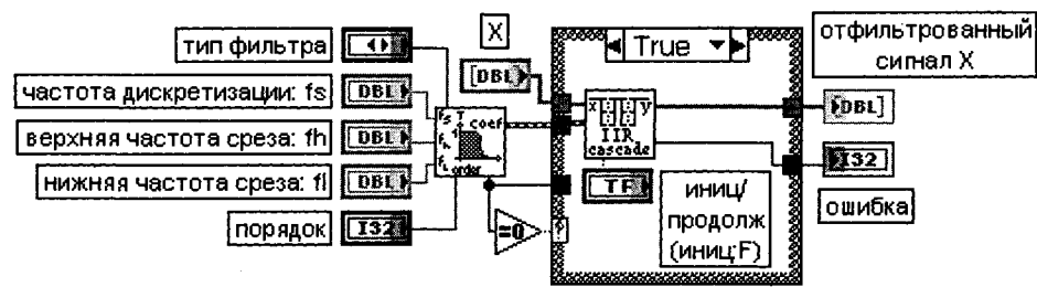
Рис. 3.22. Блок-диаграмма ВП Фильтр Баттерворта (Butterworth Filter)
