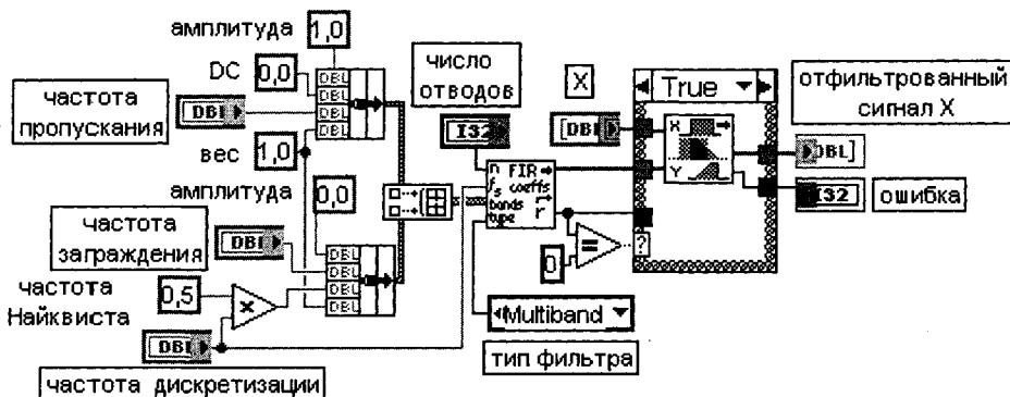
Рис 3 23. Блок-диаграмма ВП Фильтр нижних частот с равномерными пульсациями (Equi-Ripple LowPass)
