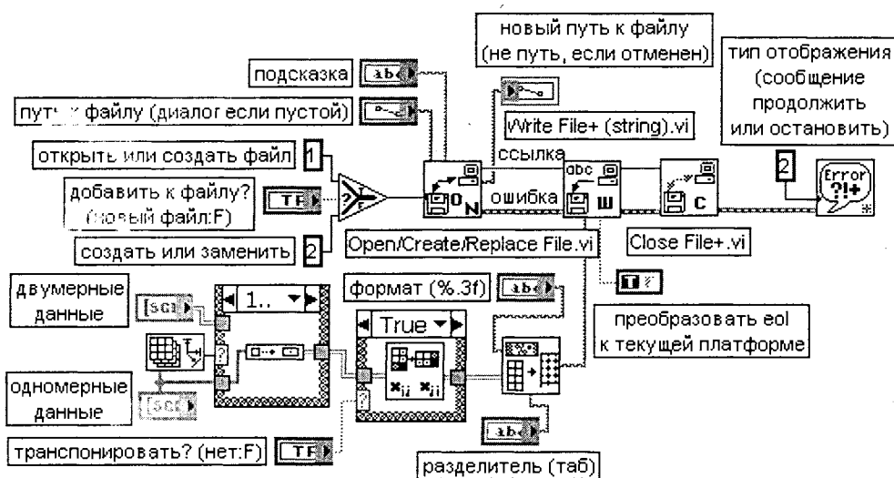
Рис 2.35 Блок-диаграмма ВП Записать в файл табличного формата (Write To Spreadsheet File)
