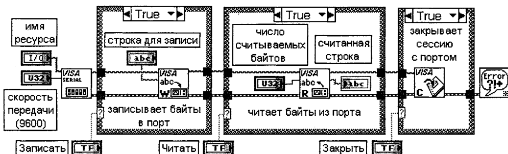
Рис 5 40. Блок-диаграмма модернизированного ВП LabVIEW ↔ Serial
