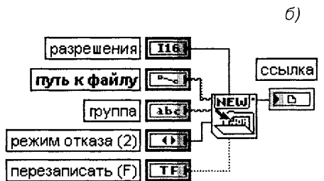
Рис. 2.39. Варианты подключения функции Создать файл (New File)
