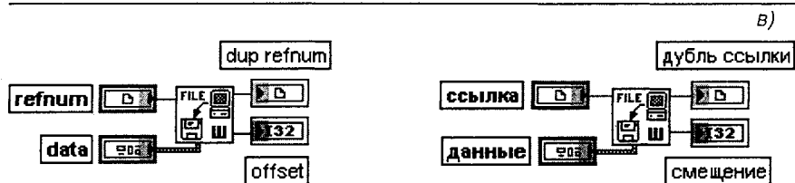
Рис. 2.36 Варианты подключения функции Записать файл (Write File)
