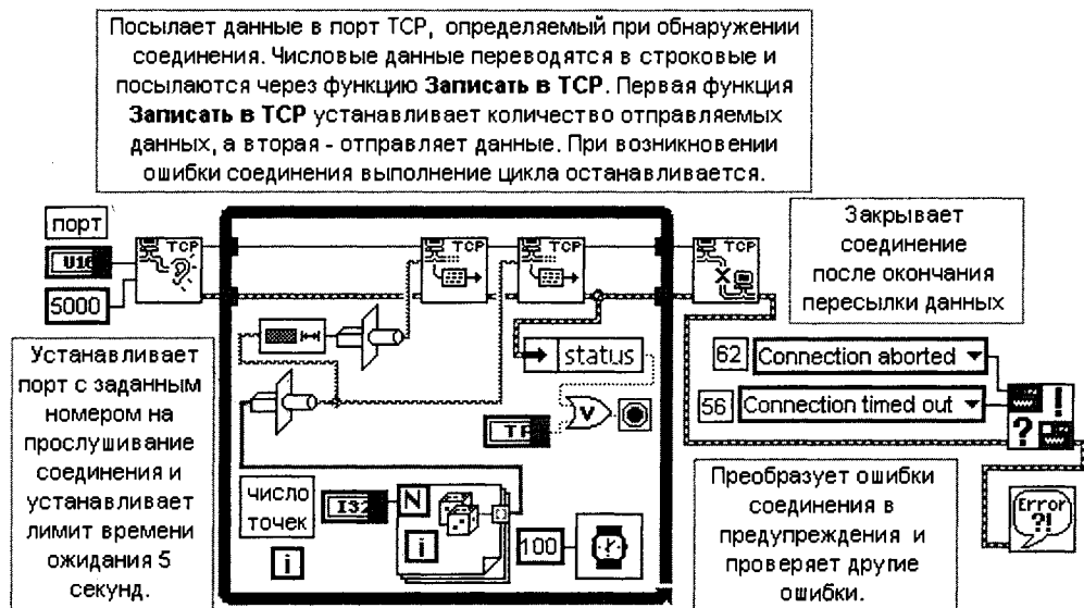
Рис. 4.25. Блок-диаграмма ВП Простой сервер данных (Simple Data Server)
