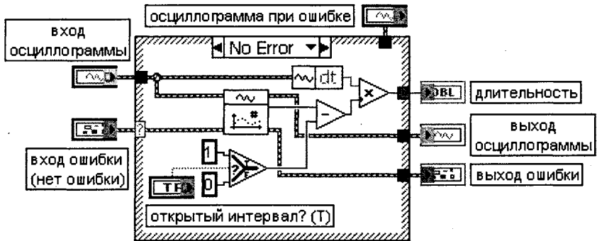
Рис 5.6 Блок-диаграмма ВП Длительность осциллограммы
