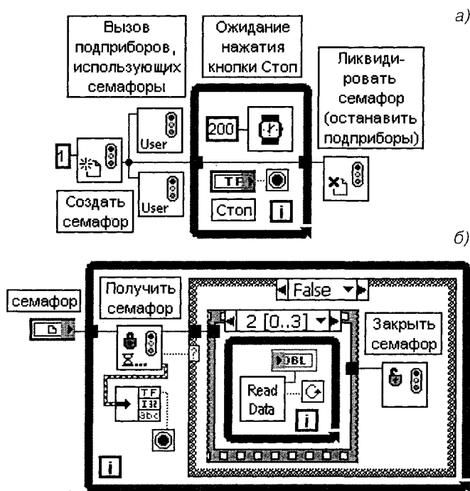
Рис. 3.61 Блок-диаграммы ВП Семафор с подприборами (Semaphore with SubVIs) (a) и подприбора (б)
