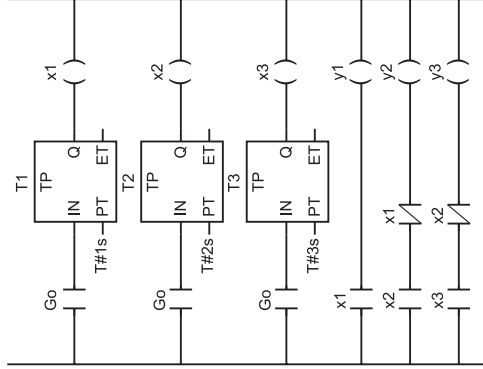
Рис. 9.2. Последовательное управление по времени в LD
