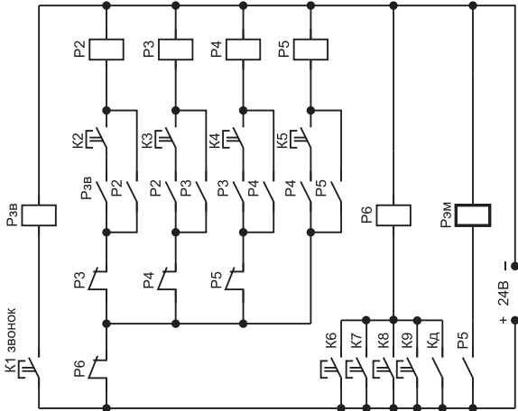
Рис. 9.6. Принципиальная схема кодового замка
