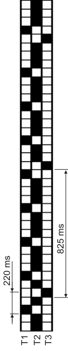
Рис. 6.2. Временная диаграмма исполнения задач T1, T2, T3
