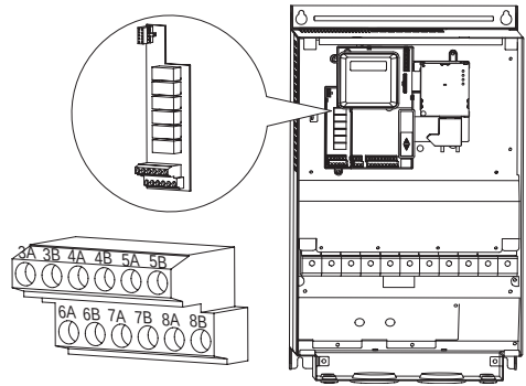
Рис. 1.1 Устанавливаемая пользователем дополнительная релейная плата (только корпуса D, Е и F)
