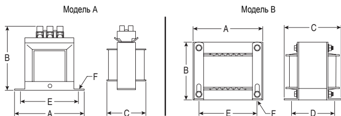
Рис. Б.7 Бюллетень 1321 - индукторы шины постоянного тока. Размеры указаны в миллиметрах (в скобках даны значения в дюймах). Масса указана в килограммах (в скобках дано значение в фунтах).
