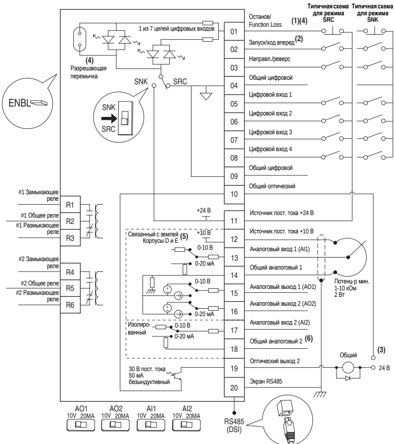
Рис. 1.1 Структурная схема цепей управления
