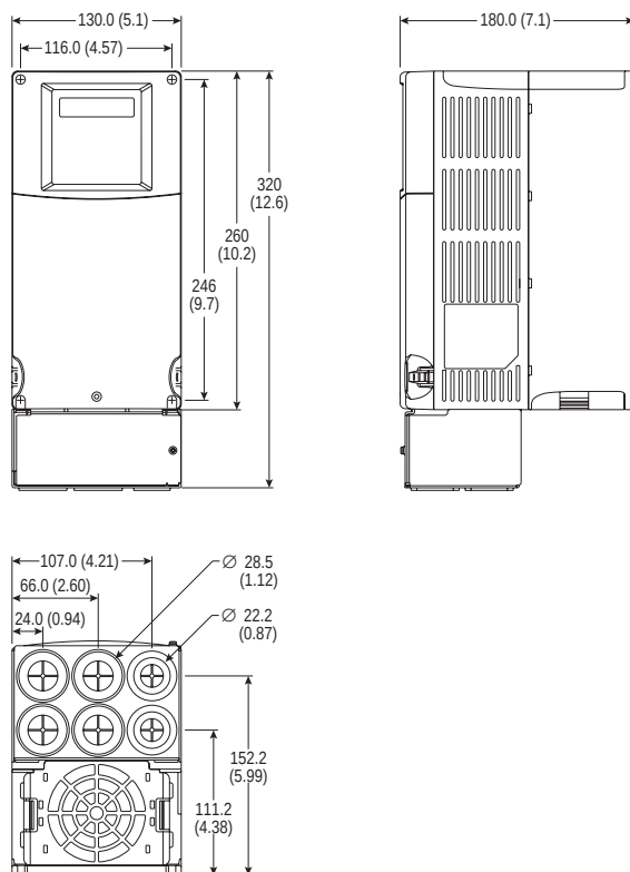
Рис. Б.1 Привод PowerFlex 400 с корпусом С. Размеры указаны в миллиметрах (в скобках даны значения в дюймах)
