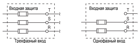
Рис. А.1 Соединения для корпусов С, D и E
