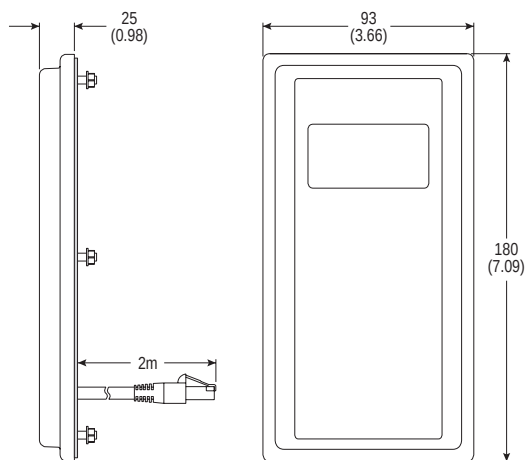
Рис. Б.9 Удаленный сокращенный модуль НІМ (крепление на панели).
