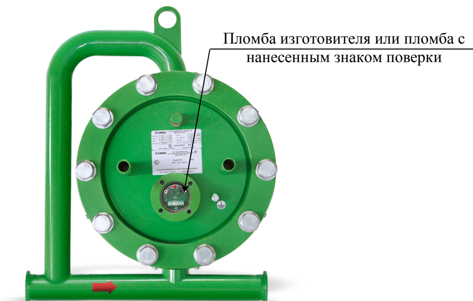
Рисунок 1 – Схема пломбировки счетчиков моноблочного и раздельного исполнения
