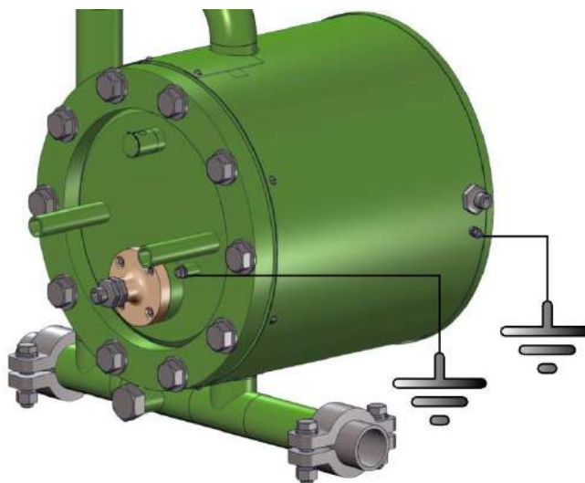
Рисунок 2.9 – Заземление счетчика
