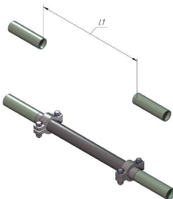
Рисунок 2.3 – Подготовка трубопровода к монтажу счетчика
