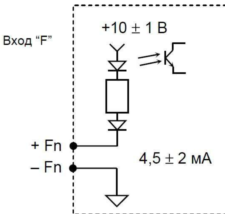
Рисунок 1.6 – Схема входов
