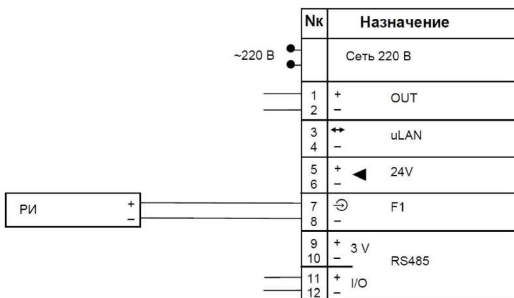
Рисунок 1.7 – Схема питания
