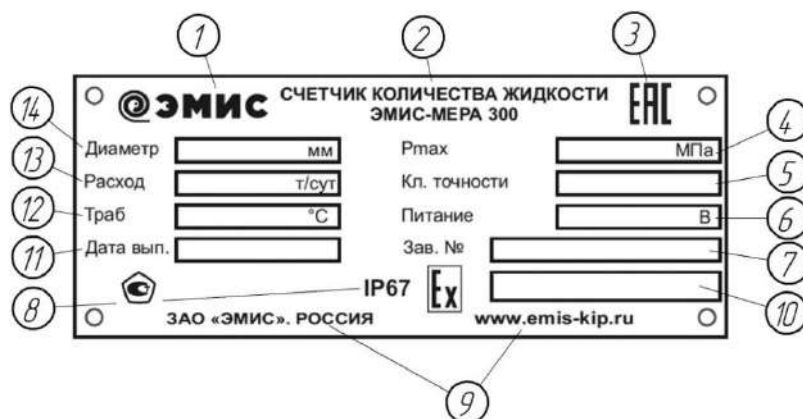
Рисунок 1.8 – Основная табличка счетчика
