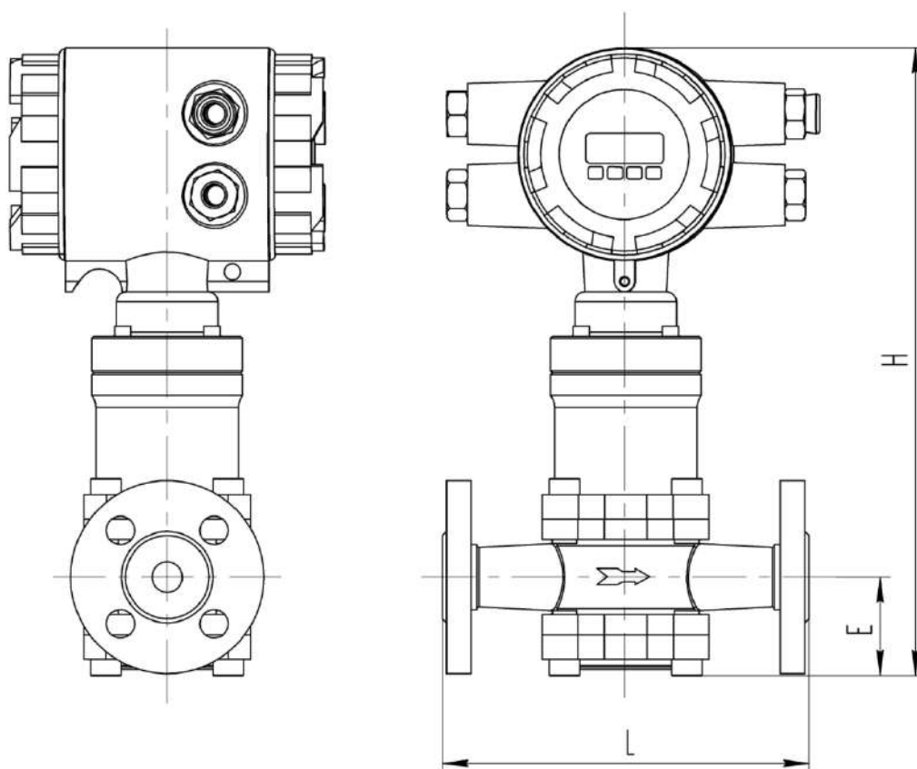
Рисунок А.1 – Внешний вид счетчика с малыми диаметрами Ду (Ду=8,15,25 мм)
