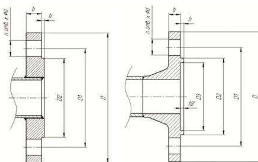
Рисунок А.6 – Размеры фланцев счетчика
