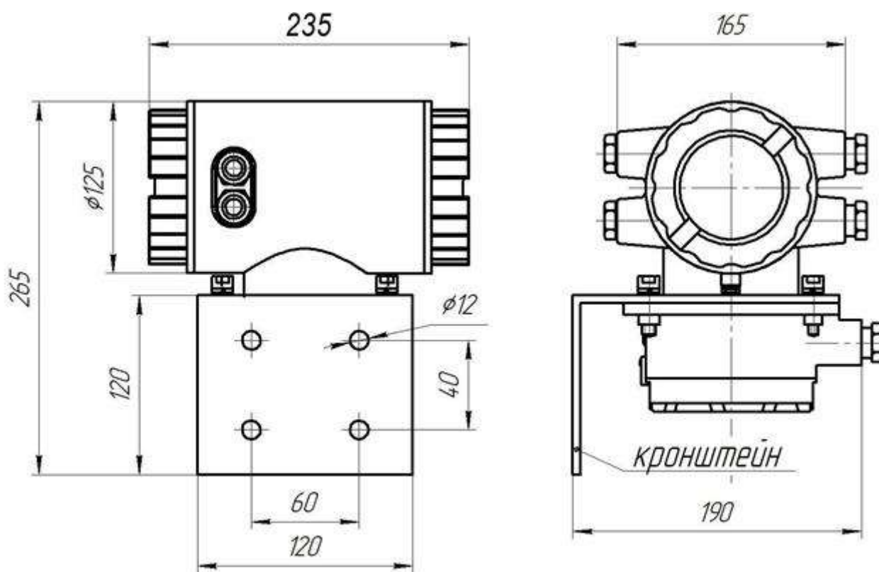
Рисунок Б.1 – Габаритные и присоединительные размеры электронного преобразователя расходомеров дистанционного исполнения
