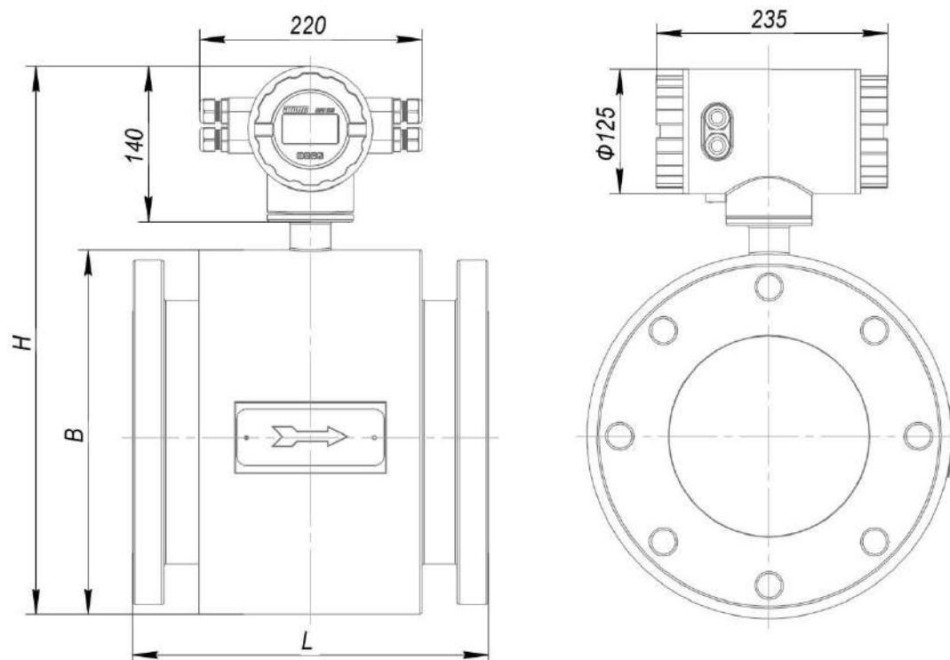
Рисунок А.3 – Габаритные и присоединительные размеры расходомера ( Dу \geq 100 мм)
