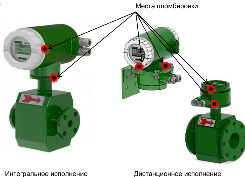
Рисунок 2.17 – Пломбирование расходомера
