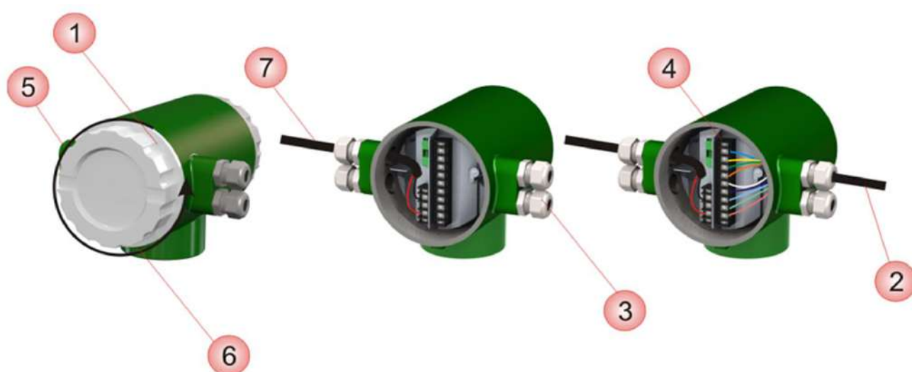
Рисунок 2.7 – Подключение электронного преобразователя
