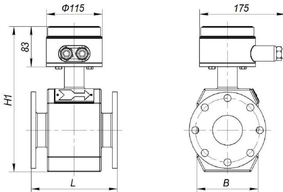
Рисунок А.2 - Габаритные и присоединительные размеры расходомера дистанционного исполнения (Ду 15 - 80мм)
