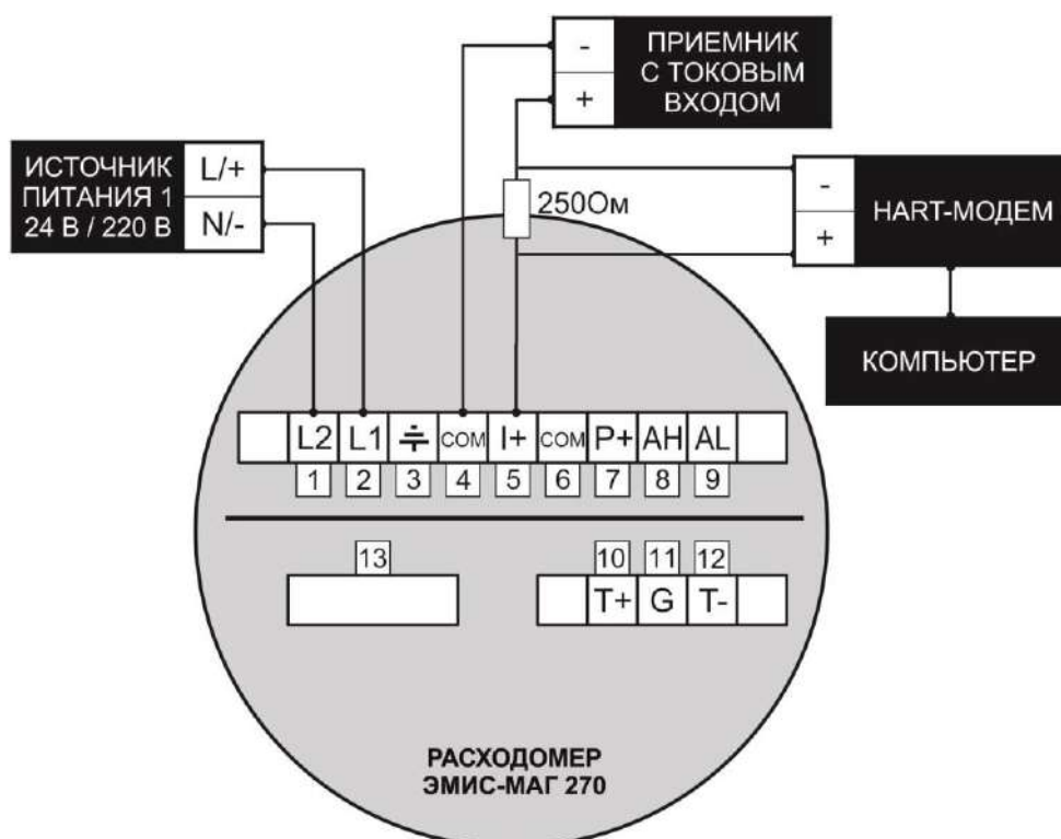
Рисунок В.5 – Схема подключения по аналоговому токовому выходному сигналу и цифровому сигналу стандарта НАРТ*
