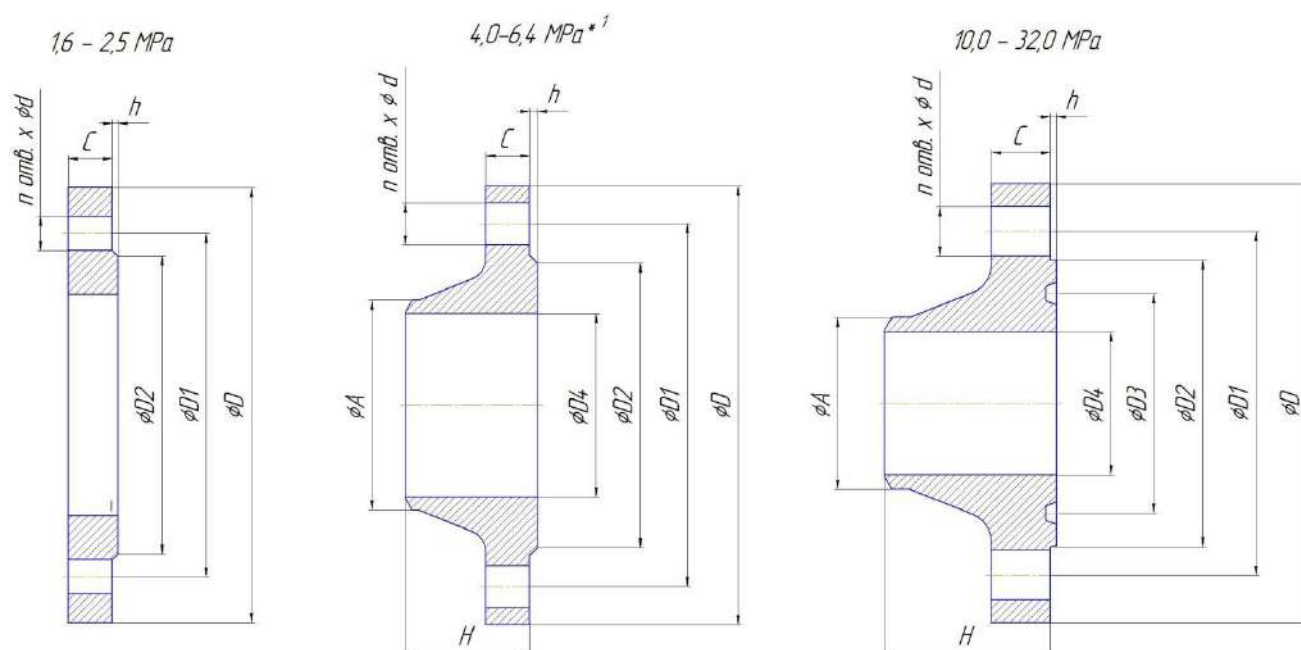
Рисунок А.5 – Присоединительные размеры фланцев расходомера и КМЧ
