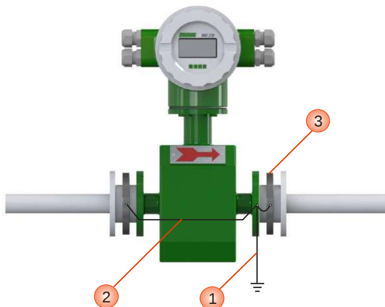
Рисунок 2.10 - Заземление расходомера
