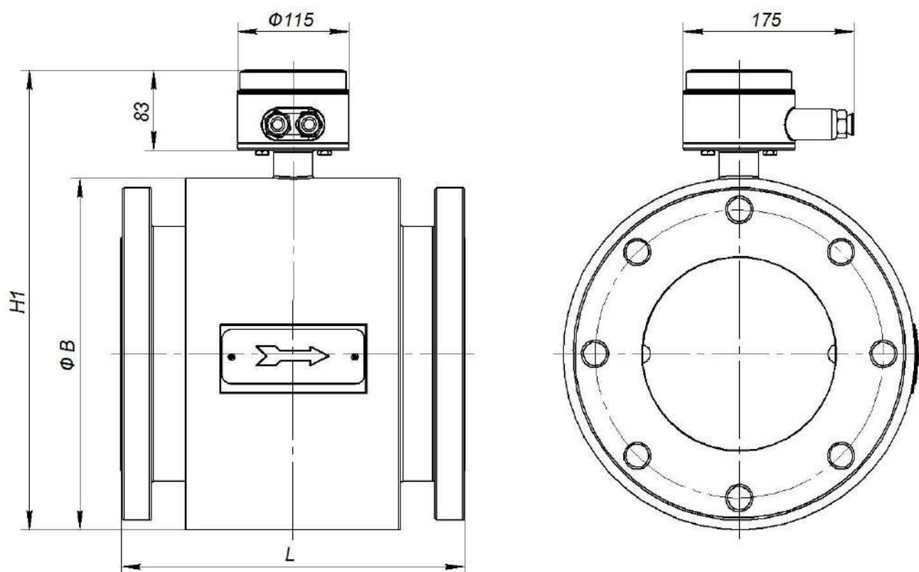
Рисунок А.4 - Габаритные и присоединительные размеры расходомера дистанционного исполнения ( Dу \geq 100 мм)
