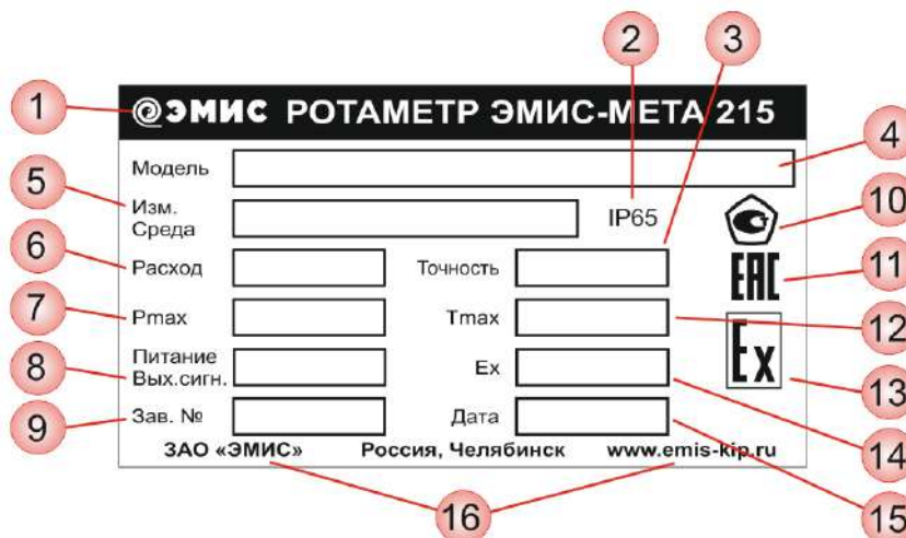
Рисунок 1.7 – Основная табличка ротаметра
