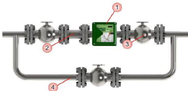
Рисунок 2.2 (а) – Установка ротаметра исполнения «Г» на горизонтальном трубопроводе
