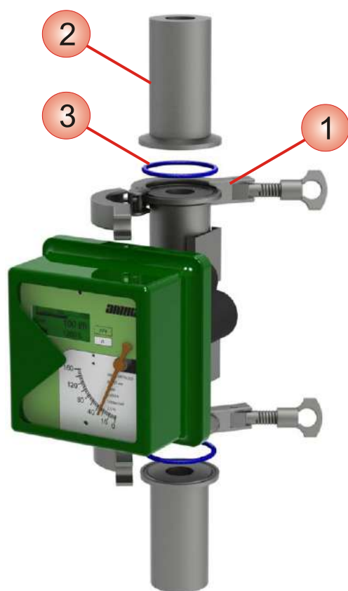
Рисунок 2.9 – Установка ротаметра с зажимным присоединением к трубопроводу
