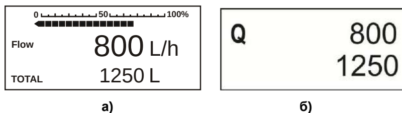
Рисунок 1.5 – ЖК дисплей
