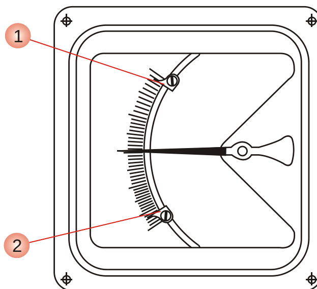
Рисунок 1.6 – Предельные выключатели
