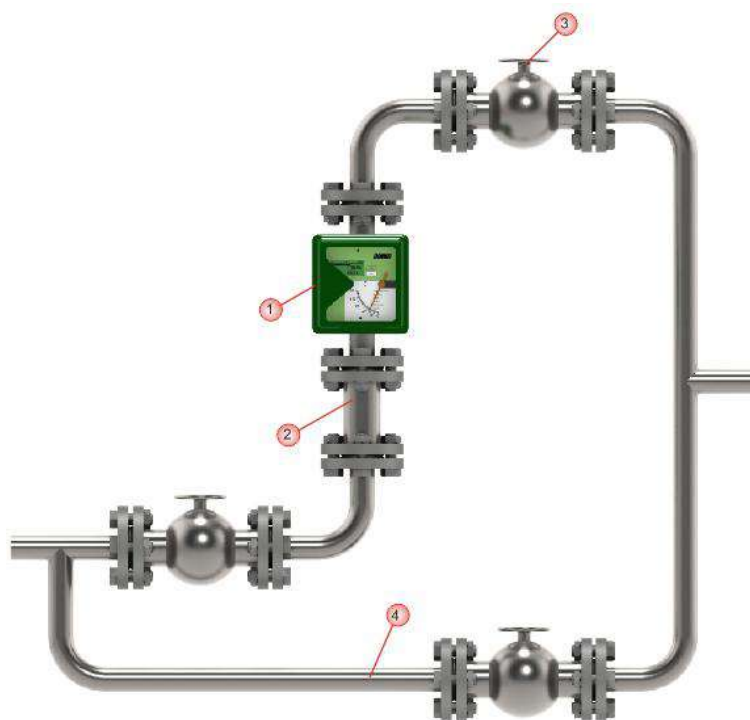
Рисунок 2.2 (в) – Установка ротаметра стандартного исполнения на горизонтальном трубопроводе
