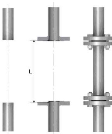
Рисунок 2.3 – Подготовка трубопровода к монтажу ротаметра с фланцевым присоединением
