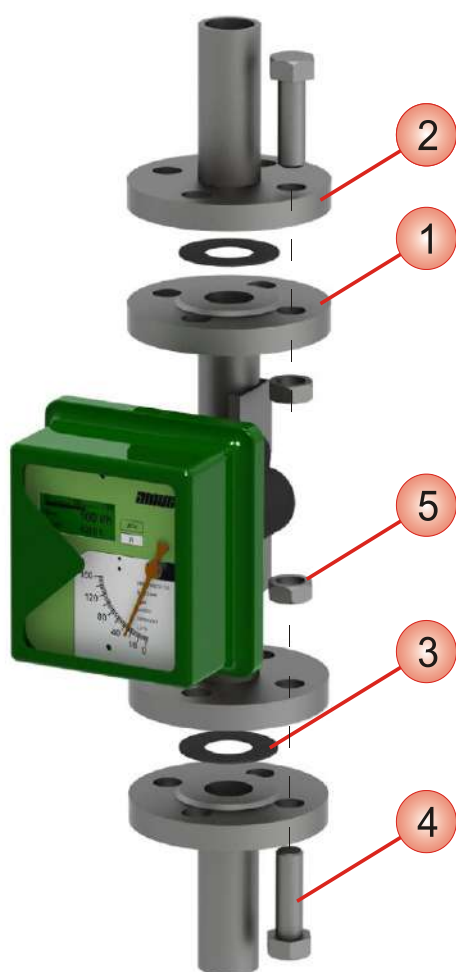
Рисунок 2.6 – Установка ротаметра с фланцевым присоединением к трубопроводу
