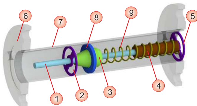
Рисунок 1.3 – Измерительный узел ротаметра исполнения «Г»
