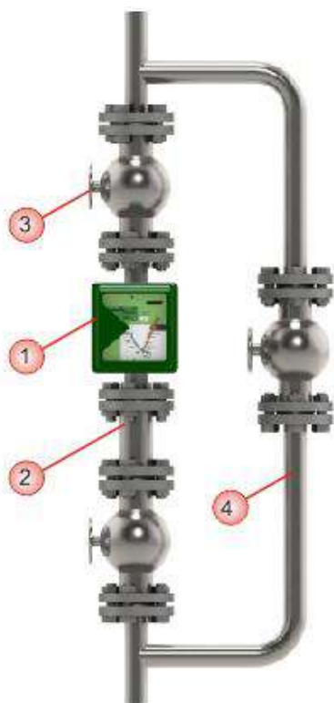
Рисунок 2.2 (б) – Установка ротаметра стандартного исполнения на вертикальном трубопроводе
