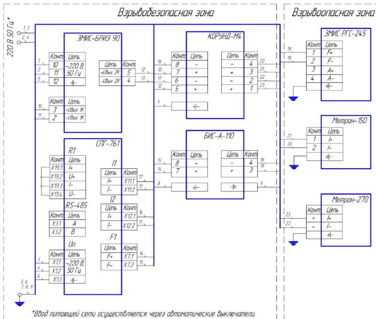
Рисунок Г.7 – Схема подключения комплекса учета газа исполнения ЭМИС-ЭСКО 2230-Р-Exi, с маркировкой взрывозащиты «1ExialIC(T4,T5) X», в составе: Контроллер – СПГ-761 ИП расхода - ЭМИС РГС-245, ИП давления – Метран-150- Exia, ИП температуры – Метран 270-Ex, Блок питания ЭМИС-БРИЗ 90-2-24-100, Барьеры искробезопасности – КОРУНД-М4, БИС-А-110-Ex
