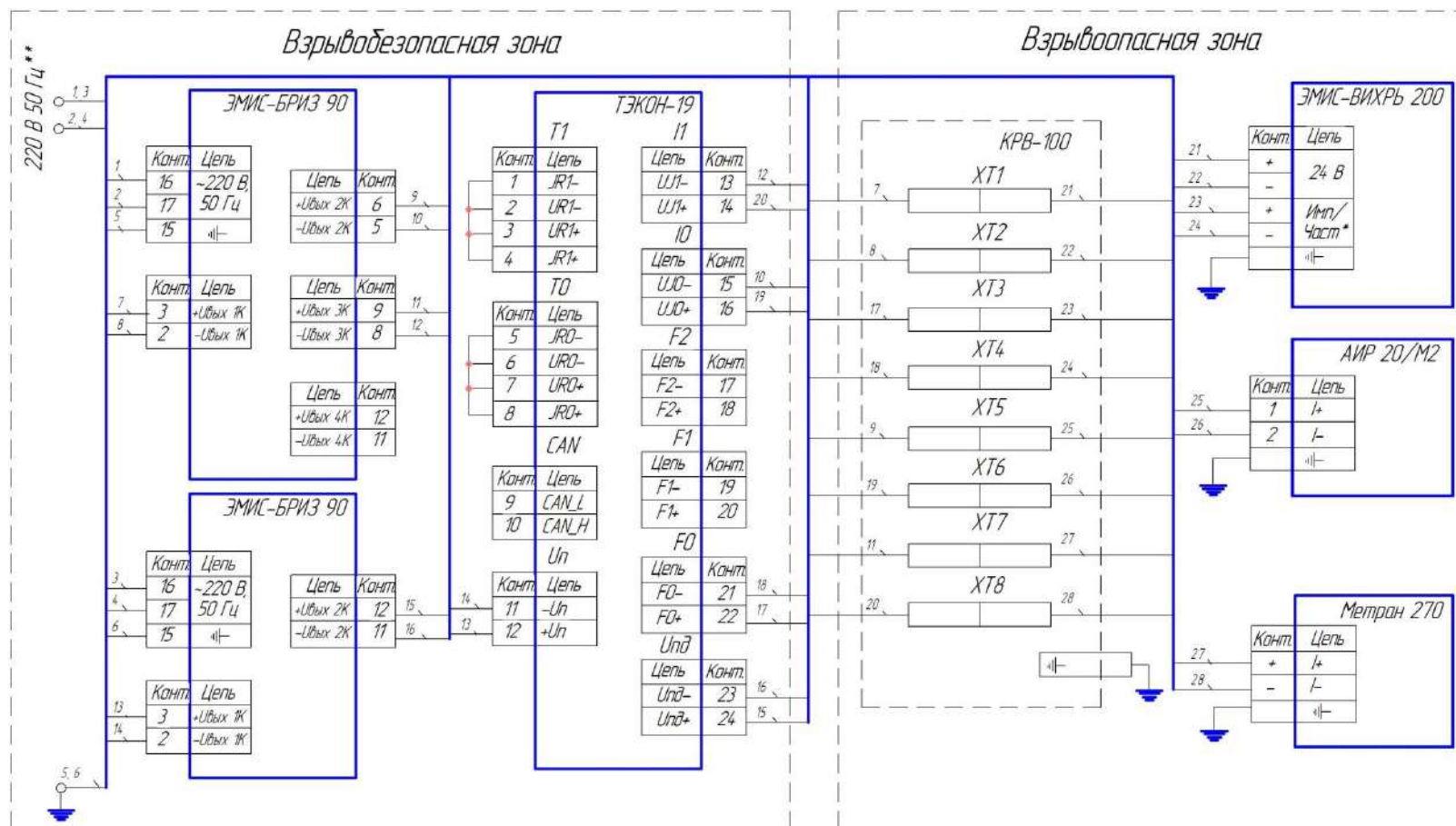
Рисунок В.1 - Схема подключения Комплекса учета газа исполнения ЭМИС-ЭСКО 2230-В-Exd, с маркировкой взрывозащиты «1ExdIICT(T2,T5,T6) X», в составе: ИП расхода – ЭМИС-ВИХРЬ 200-Вн, ИП давления – АИР 20/М2 Exd, ИП температуры – Метран 270-Exd, Контроллер – ТЭКОН-19, Блоки питания ЭМИС-БРИЗ 90-4-24-100, ЭМИС-БРИЗ 90-2-24-250, Коробка распределительная взрывозащищенная – Кр-В-100d.
