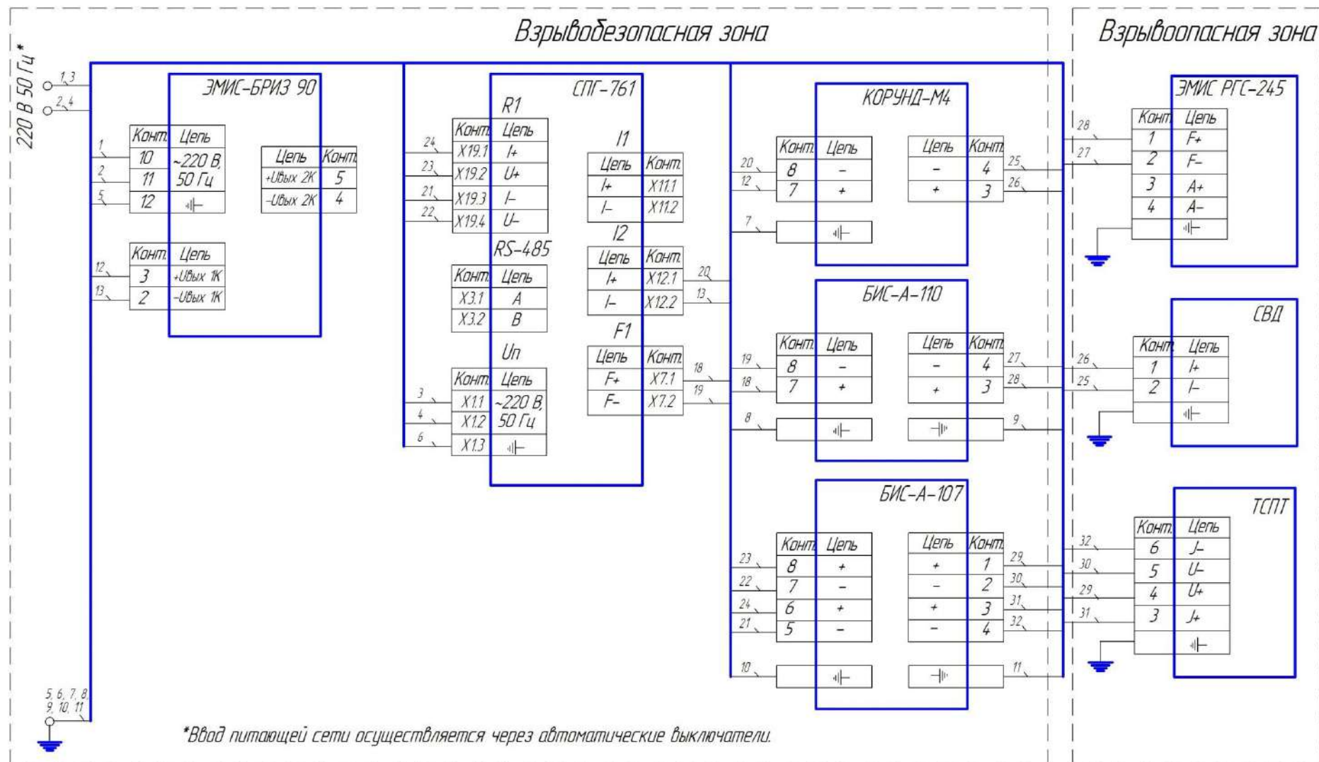
Рисунок Г.6 – Схема подключения комплекса учета газа исполнения ЭМИС-ЭСКО 2230-Р-Exi, с маркировкой взрывозащиты «1ExialICT4 X», в составе: Контроллер – СПГ761, ИП расхода – ЭМИС РГС-245, ИП давления СВД – Ex, ИП температуры – ТСПТ, Блок питания ЭМИС-БРИЗ 90-2-24-100, Барьеры искробезопасности – КОРУНД-М4, БИС-А-107-Ex, БИС-А-110-Ex
