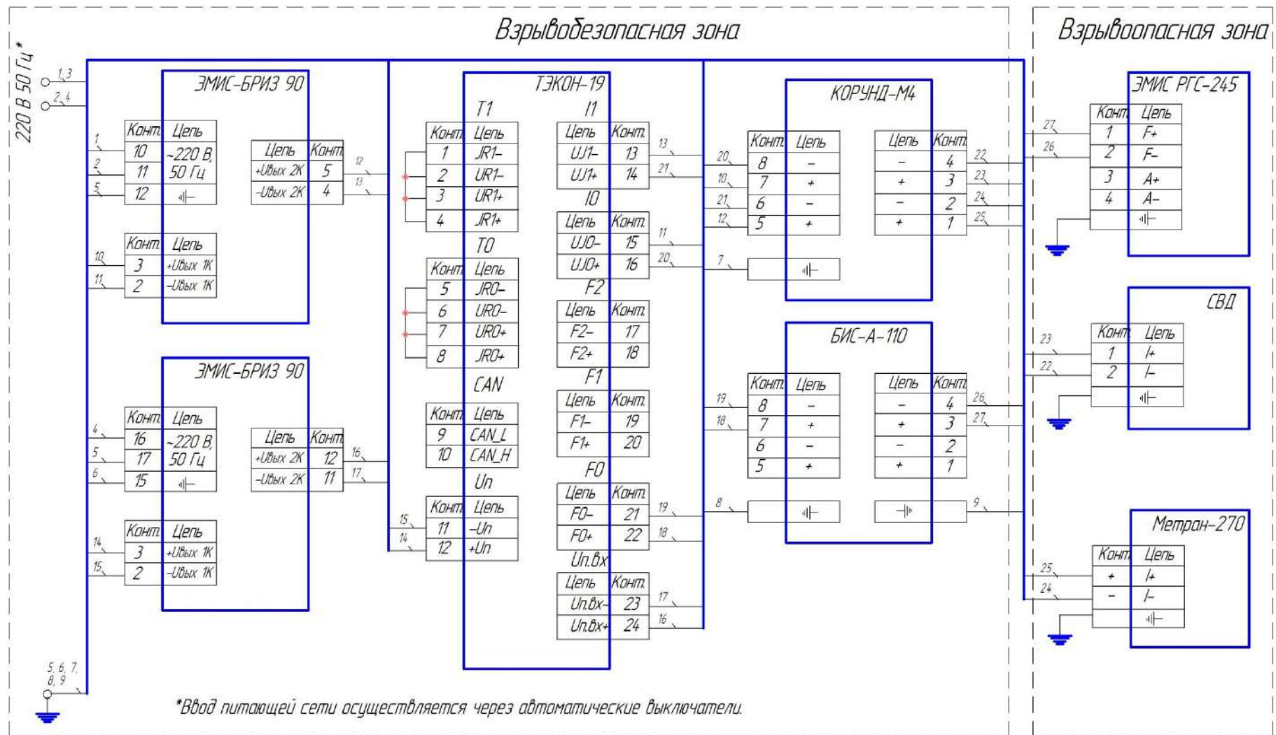
Рисунок Г.3 – Схема подключения комплекса учета газа исполнения ЭМИС-ЭСКО 2230-Р-Exi, с маркировкой взрывозащиты «1ExiaIICT4 X» в составе: Контроллер – ТЭКОН-19, ИП расхода - ЭМИС РГС-245, ИП давления - СДВ-Ех, ИП температуры – Метран 270-Ех, Блоки питания ЭМИС-БРИЗ 90-4-24-100, ЭМИС-БРИЗ 90-2-24-250, Барьеры искробезопасности – КОРУНД-М4, БИС-А-110
