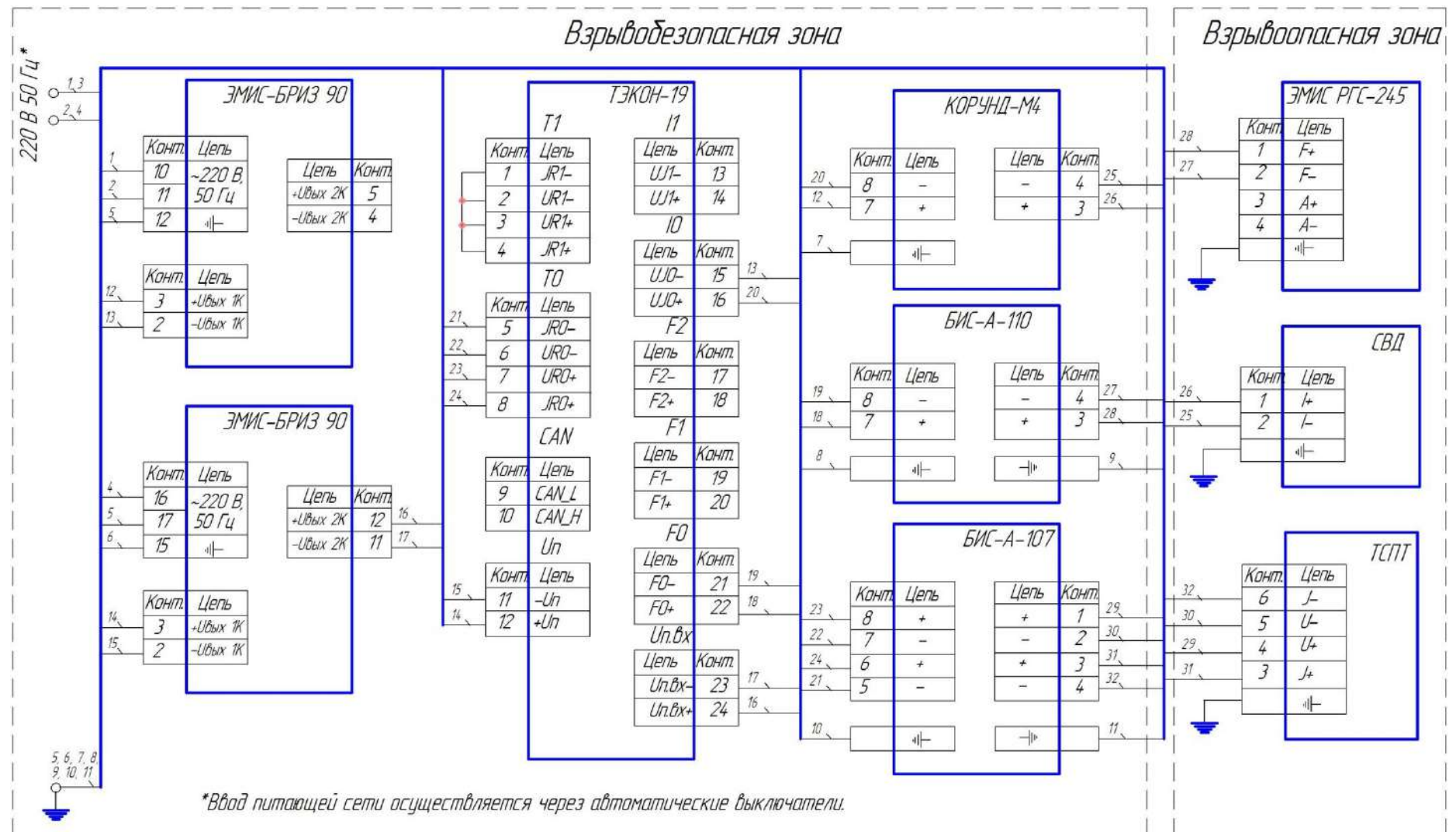
Рисунок Г.5 – Схема подключения комплекса учета газа исполнения ЭМИС-ЭСКО 2230-Р-Exi, с маркировкой взрывозащиты «1ExialICT4 X», в составе: Контроллер – ТЭКОМ-19, ИП расхода – ЭМИС РГС-245, ИП давления СДВ-Ex, ИП температуры – ТСПТ-Ex, Блоки питания ЭМИС-БРИЗ 90-4-24-100, ЭМИС-БРИЗ 90-2-24-250, Барьеры искробезопасности – КОРУНД-М4, БИС-А-107-Ex, БИС-А-110-Ex
