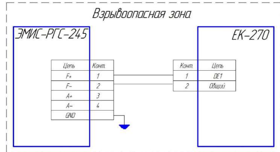
Рисунок Г.2 – Схема подключения комплекса учета газа исполнения ЭМИС-ЭСКО 2230-Р-БК-Ехi, с маркировкой взрывозащиты «1ExibIIBT4 X», в составе: Блок коррекции – ЕК-270, ИП расхода- ЭМИС РГС-245.
