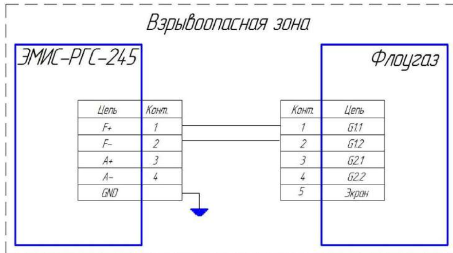
Рисунок Г.1 – Схема подключения комплекса учета газа исполнения ЭМИС-ЭСКО 2230-Р-БК-Ехi, с маркировкой взрывозащиты «1ExibIIBT4 X», в составе: Блок коррекции – ФЛОУГАЗ, ИП расхода- ЭМИС РГС-245.
