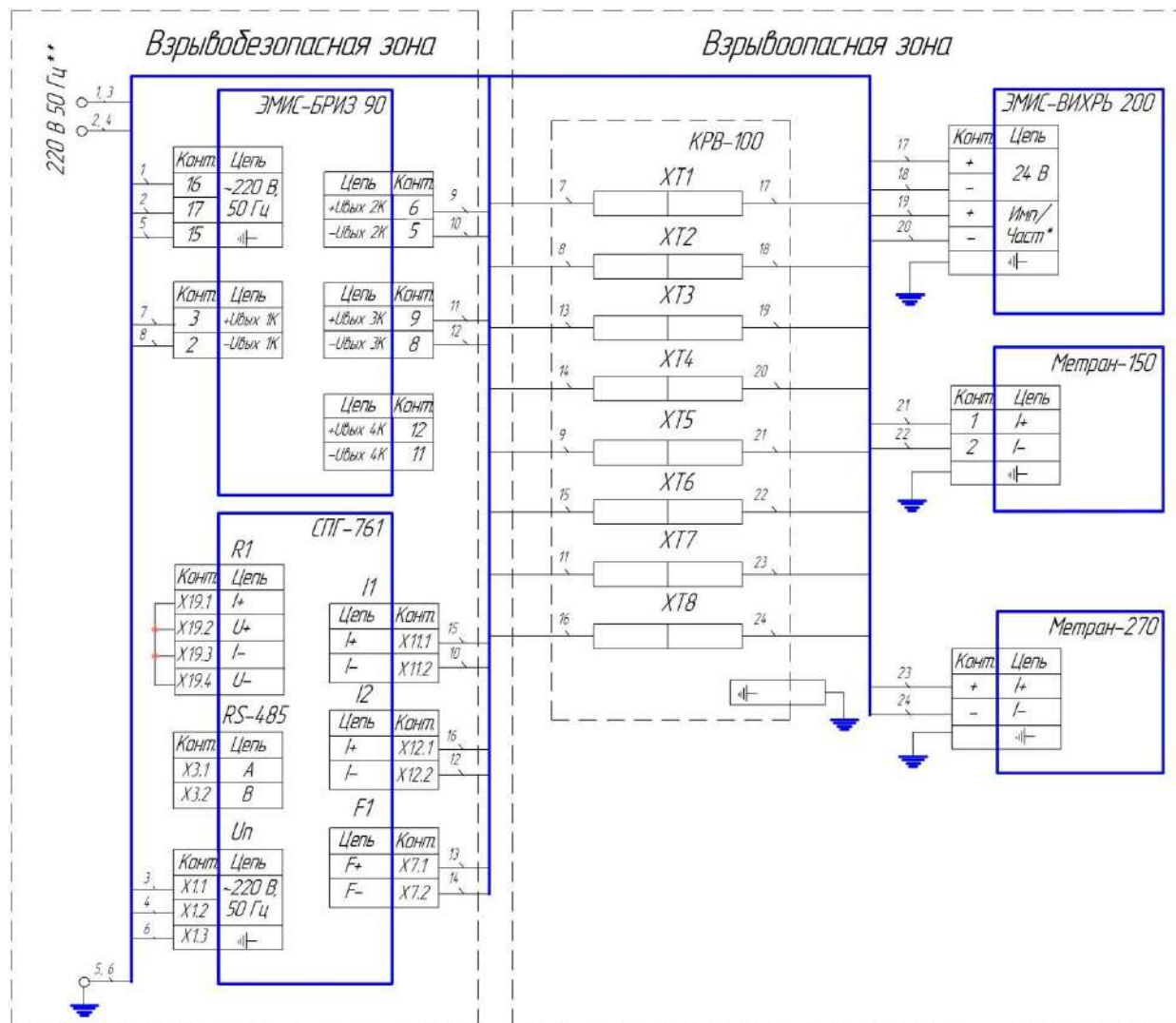
Рисунок В.5 - Схема подключения Комплекса учета газа исполнения ЭМИС-ЭСКО 2230-В-Exd, с маркировкой взрывозащиты «1ExdIICT2,T5,T6) X» в составе: ИП расхода – ЭМИС-ВИХРЬ 200-Вн, ИП давления – Метран-150- Exd, ИП температуры – Метран 270-Exd, Контроллер – СПГ 761, Блок питания ЭМИС-БРИЗ 90-4-24-100, Коробка распределительная взрывозащищенная – Кр-В-100d.
