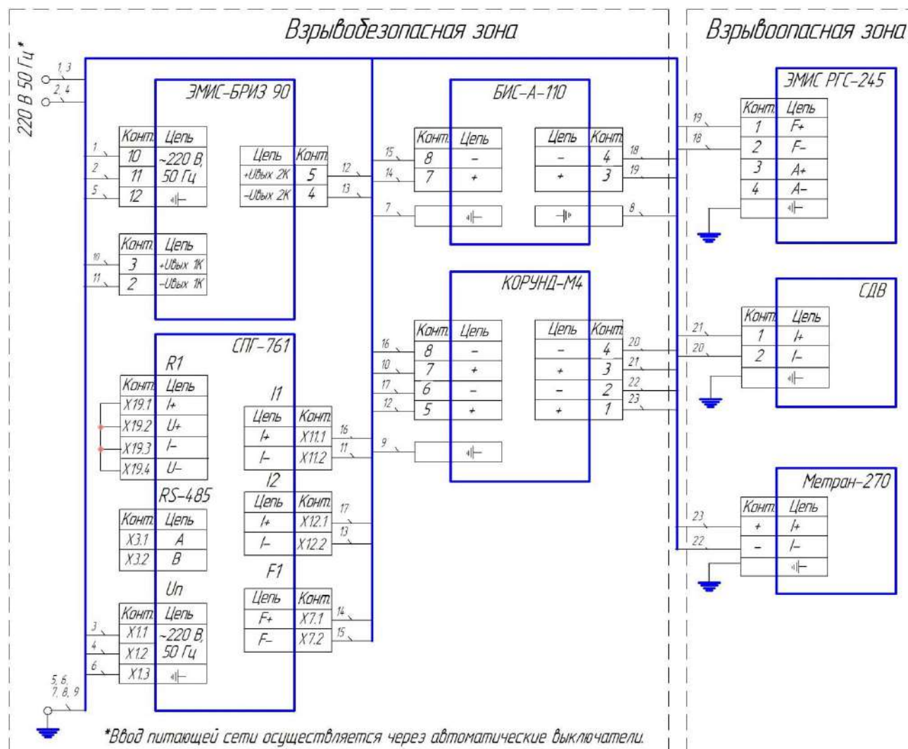
Рисунок Г.8 – Схема подключения комплекса учета газа исполнения ЭМИС-ЭСКО 2230-Р-Exi, с маркировкой взрывозащиты «1ExiaIICT4,T5) X», в составе: Контроллер – СПГ761, ИП расхода - ЭМИС РГС-245, ИП давления СДВ, ИП температуры – Метран-270-Ex, Блок питания ЭМИС-БРИЗ 90-4-24-100, Барьеры искробезопасности – КОРУНД-М4, БИС-А-110-Ex
