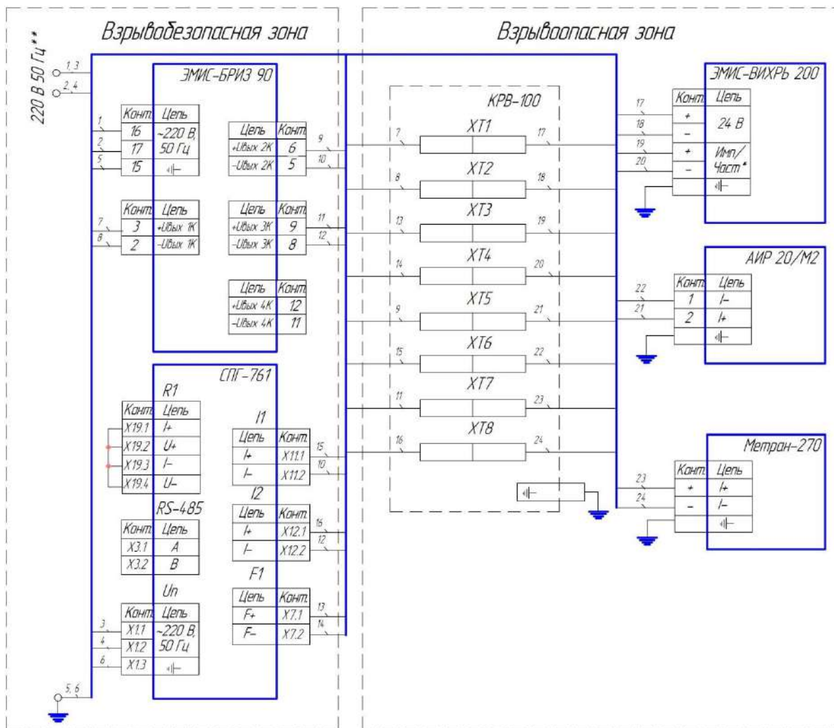
Рисунок В.4 - Схема подключения Комплекса учета газа исполнения ЭМИС-ЭСКО 2230-В-Exd, с маркировкой взрывозащиты «1ExdIIC(T2,T5,T6) X», в составе: ИП расхода – ЭМИС-ВИХРЬ 200-Вн, ИП давления – АИР 20/М2 Exd, ИП температуры – Метран 270-Exd, Контроллер – СПГ 761, Блок питания ЭМИС-БРИЗ 90-4-24-100, Коробка распределительная взрывозащищенная - Кр-В-100d
