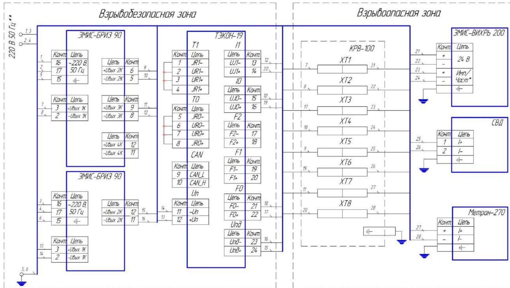
Рисунок В.3 - Схема подключения Комплекса учета газа исполнения ЭМИС-ЭСКО 2230-B-Exd, с маркировкой взрывозащиты «1ExdIICT2 X», в составе: ИП расхода – ЭМИС-ВИХРЬ 200-Вн, ИП давления – СВД-Smart-Exd, ИП температуры – Метран 270-Exd, Контроллер – ТЭКОН-19, Блоки питания ЭМИС-БРИЗ 90-4-24-100, ЭМИС-БРИЗ 90-2-24-250, Коробка распределительная взрывозащищенная – Кр-В-100d.
