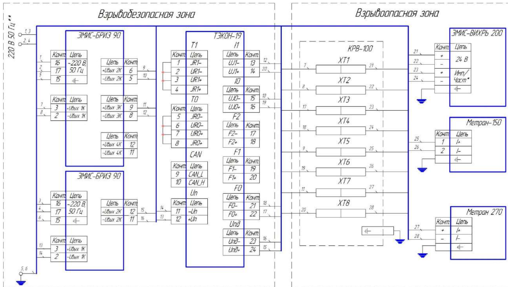
Рисунок В.2 – Схема подключения Комплекса учета газа исполнения ЭМИС-ЭСКО 2230-В-Exd, с маркировкой взрывозащиты «1ExdIIС(T2,T5,T6) X», в составе: ИП расхода – ЭМИС-ВИХРЬ 200-Вн, ИП давления – Метран-150-Exd, ИП температуры – Метран 270-Exd, Контроллер – ТЭКОН-19, Блоки питания ЭМИС-БРИЗ 90-4-24-100, ЭМИС-БРИЗ 90-2-24-250, Коробка распределительная взрывозащищенная – Кр-В-100d.
