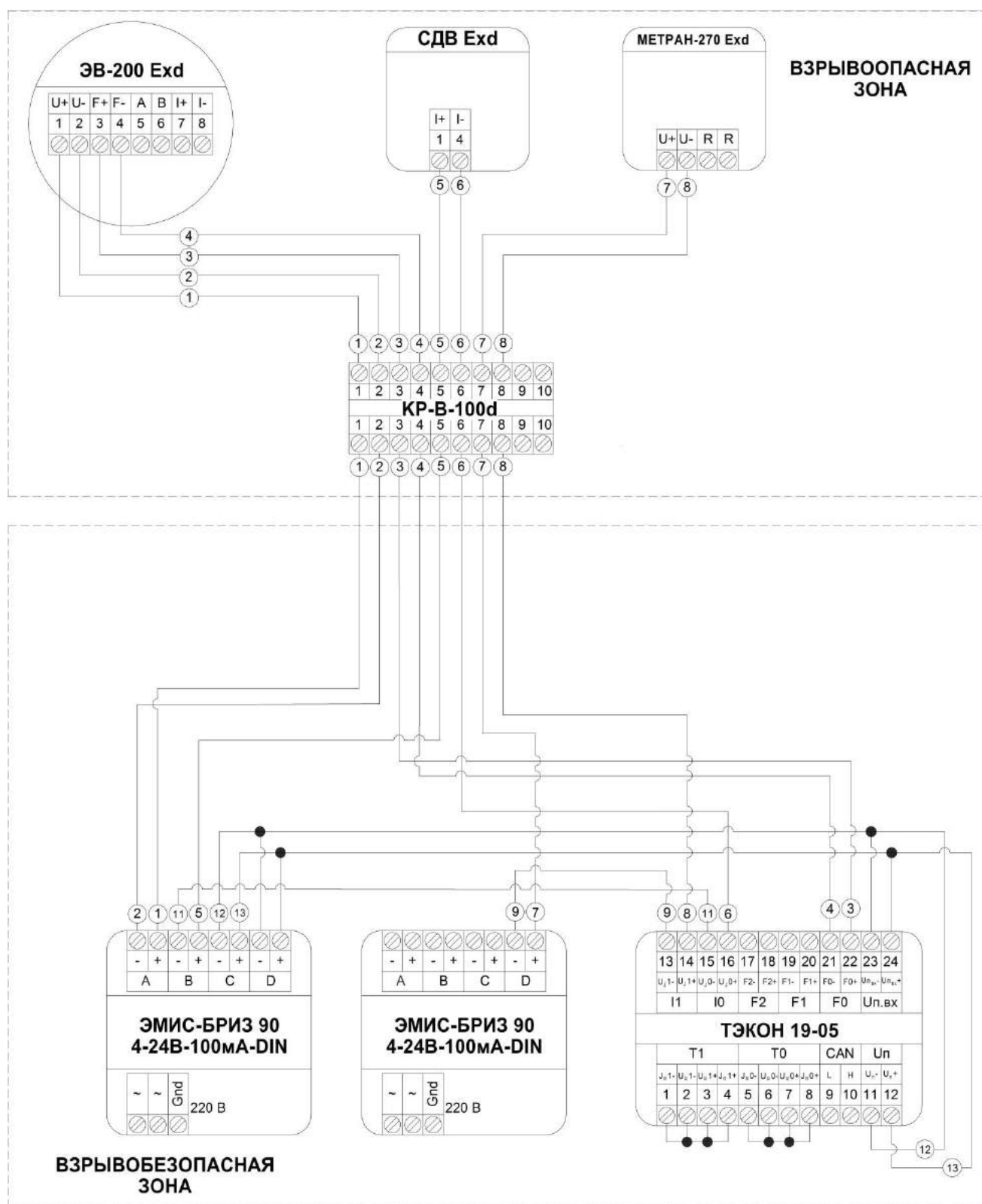
Схема 3. – Подключение узла типа Exd во взрывоопасной зоне с датчиком температуры с выходным сигналом 4-20
