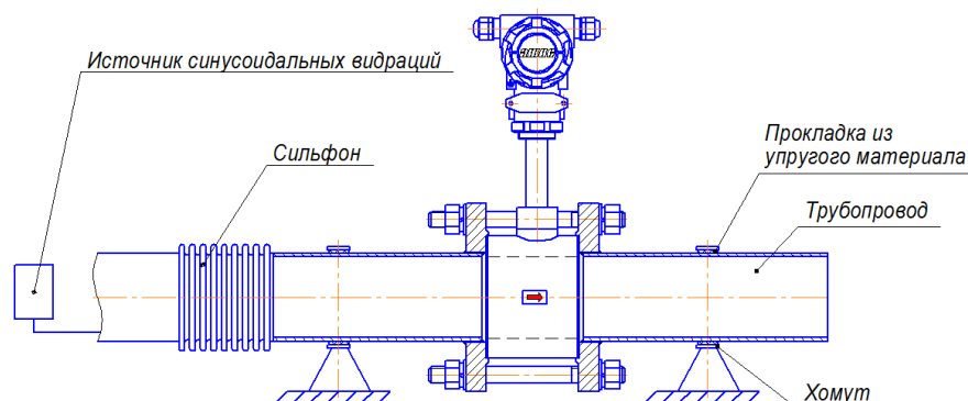
Рисунок 2.7 – Закрепление трубопровода После закрепления трубопровода проверить отсутствие «самохода».
