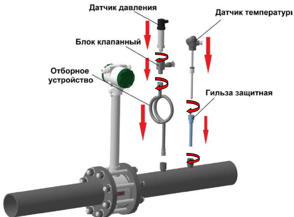
Рисунок 2.4 – Схема монтажа преобразователя давления и преобразователя температуры
