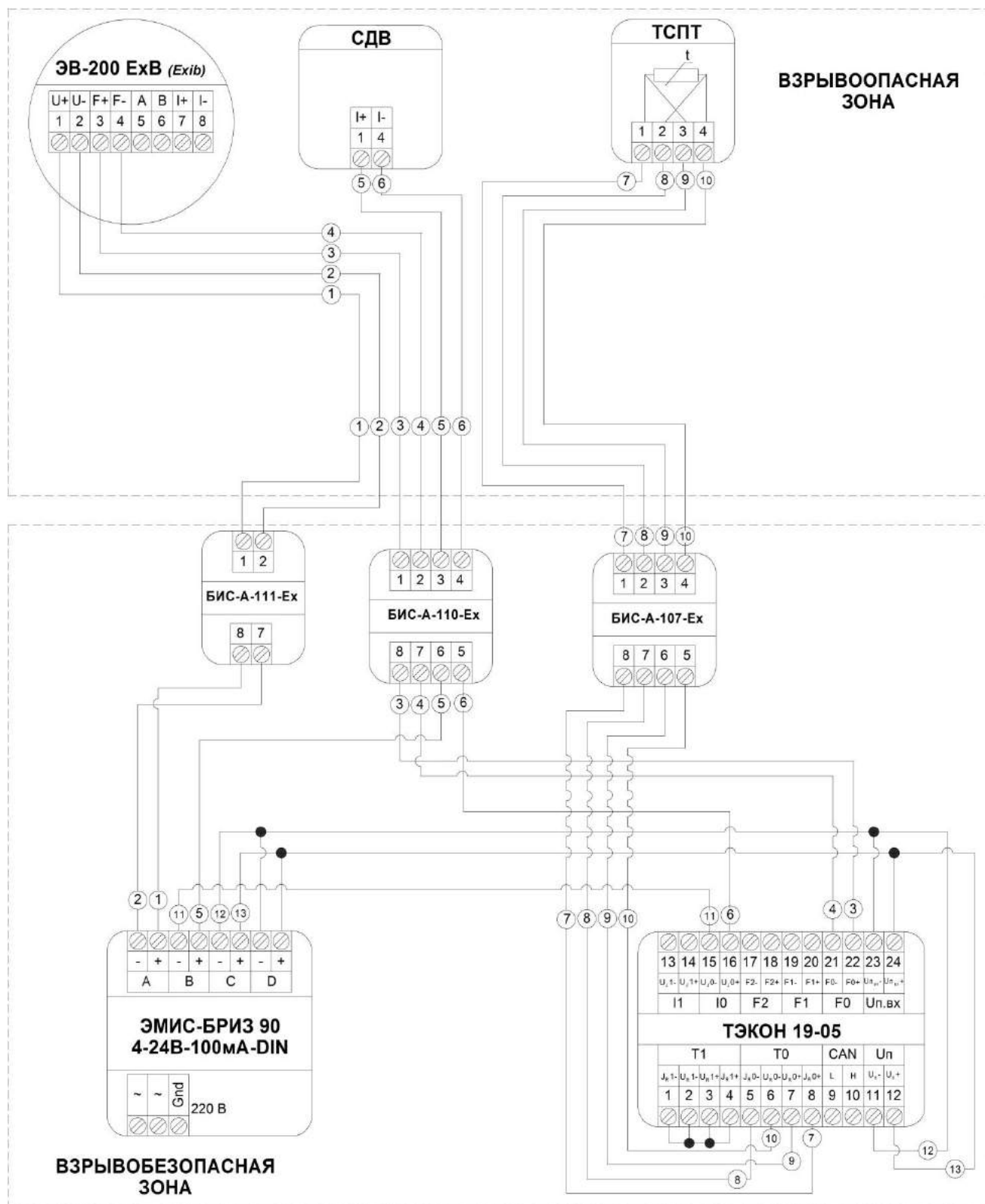
Схема 5. – Подключение узла типа Exi во взрывоопасной зоне с датчиком температуры с выходным сигналом по сопротивлению
