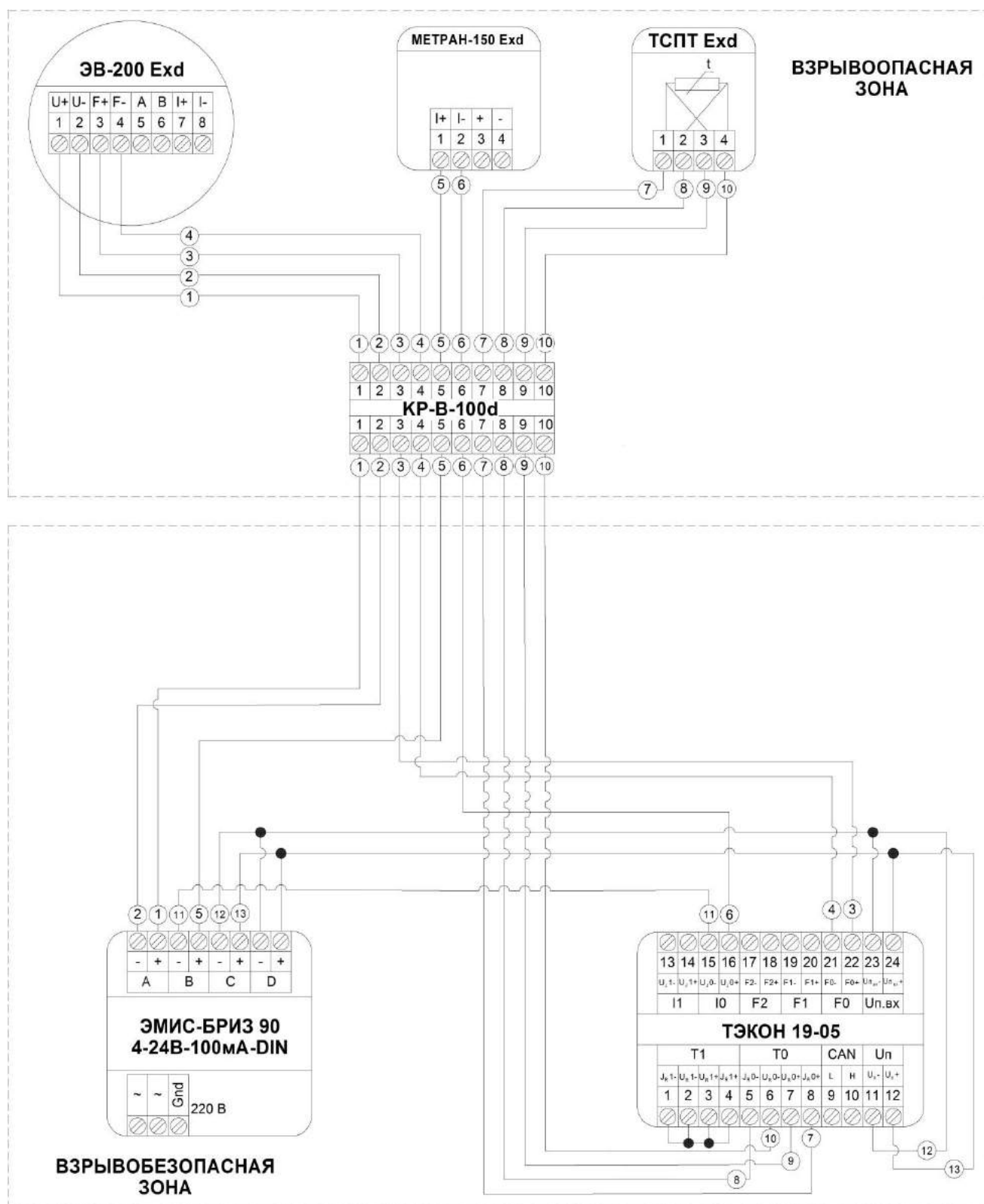
Схема 6. – Подключение узла типа Exd во взрывоопасной зоне с датчиком температуры с выходным сигналом по сопротивлению
