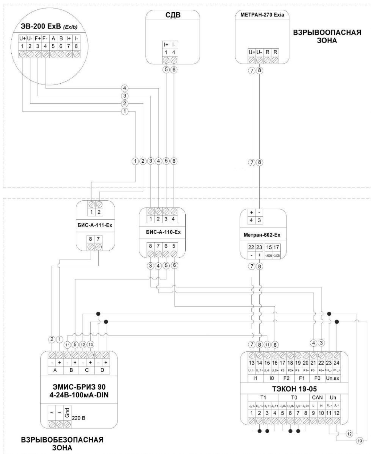
Схема 4. – Подключение узла типа Exi во взрывоопасной зоне с датчиком температуры с выходным сигналом 4-20
