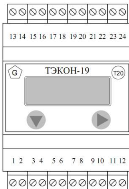
Рисунок 2.6 —Внешний вид передней панели и нумерация клемм ТЭКОН-19-05
