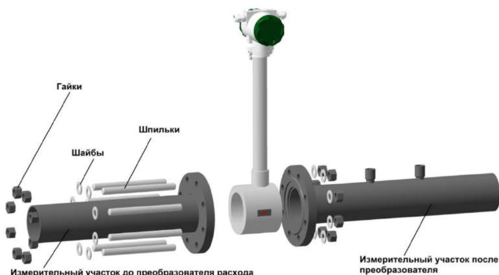
Рисунок 2.1 – Сборка преобразователя расхода
