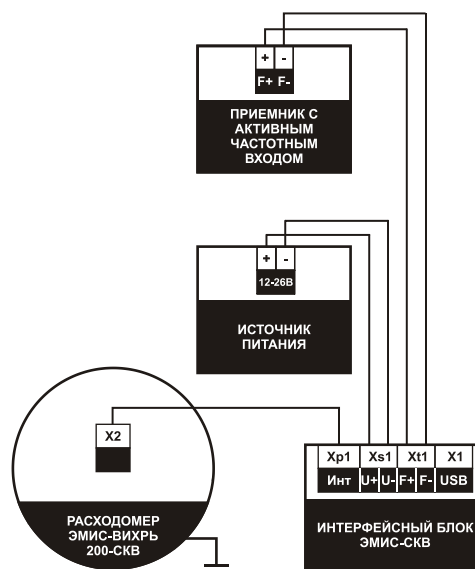
Рисунок Б.5 - Схема подключения преобразователя ЭВ-200-СКВ к прибору с активным частотным входом
