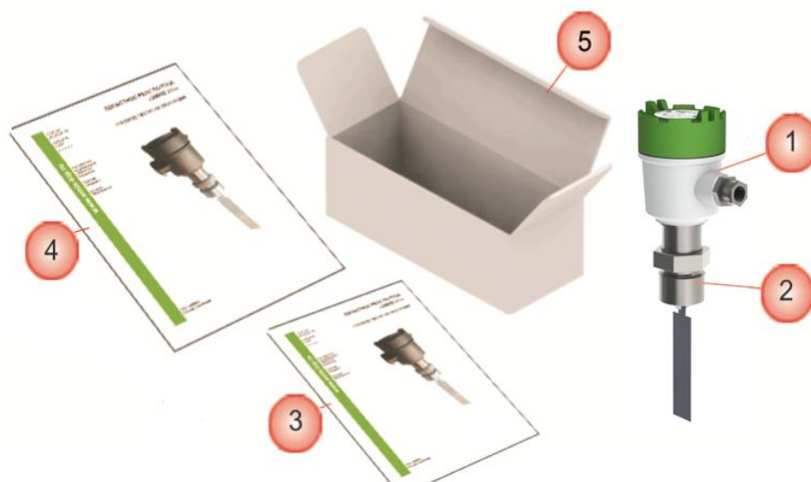
Рисунок 1.5 – Комплект поставки
