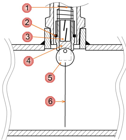
Рисунок 1.2 А) – Герконовое реле разомкнуто
