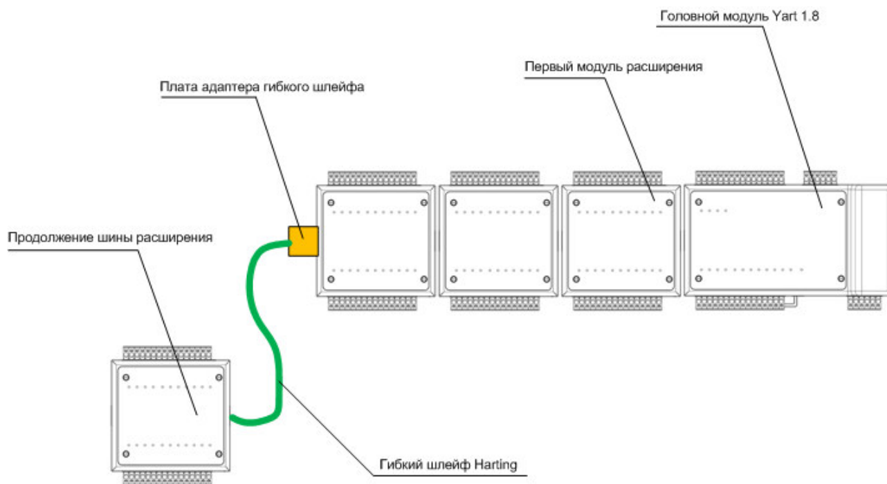
Рисунок 2 – Подключение модулей расширения к Контроллеру
