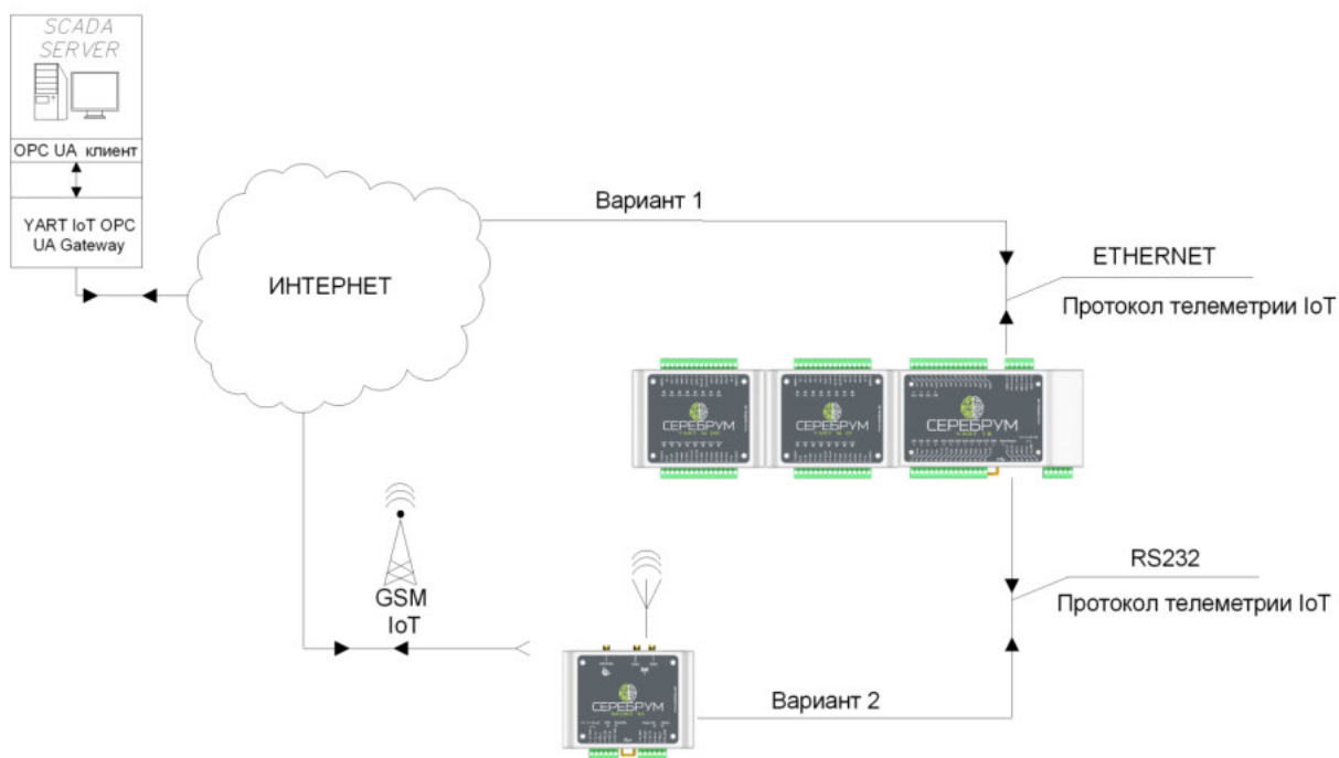
Рисунок 5а - Пример построения систем диспетчеризации: интернет
