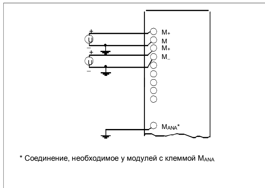
Рис. 5–9. Подключение датчиков напряжения к аналоговому входу
