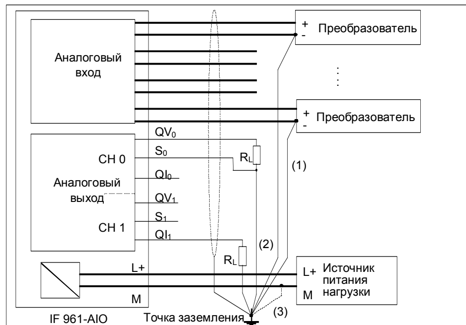
Рис. 13–12. Заземление аналоговых входов и выходов интерфейсного субмодуля IF 961-AIO
