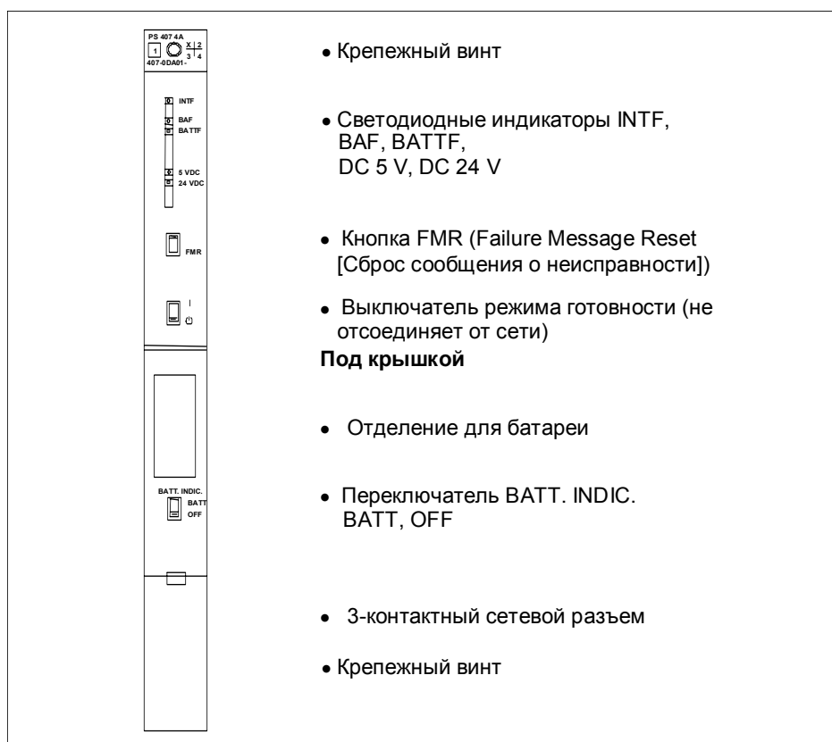
Рис. 3–3. Органы управления и индикаторы PS 407 4 A
