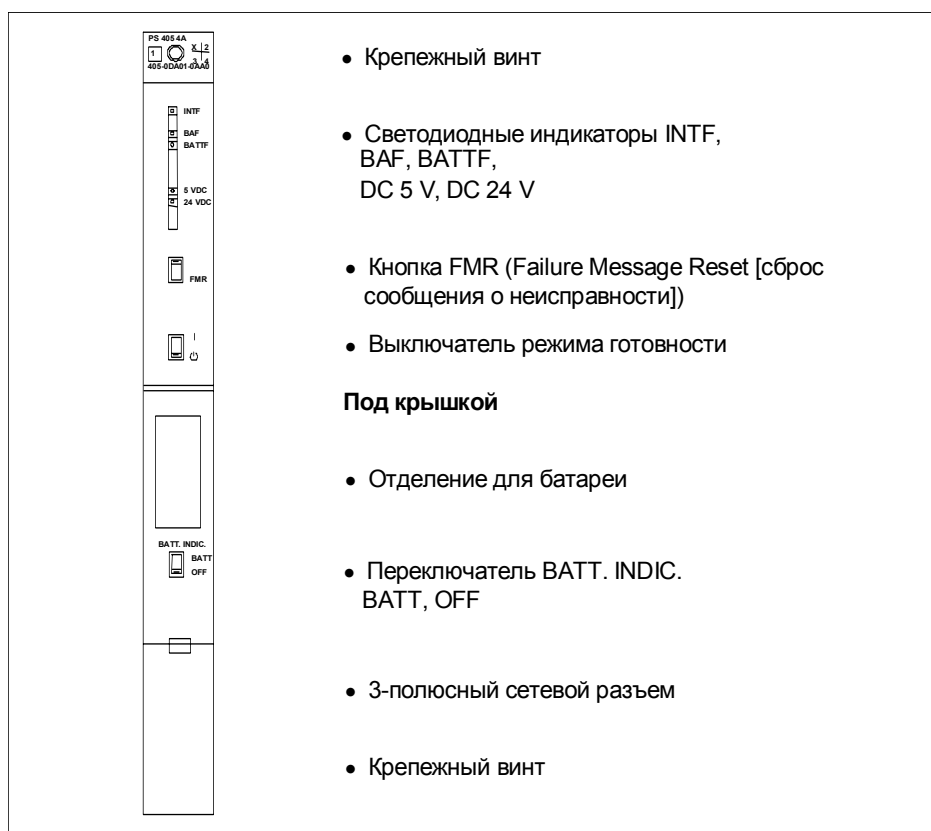
Рис. 3–8. Органы управления и индикаторы PS 405 4 A
