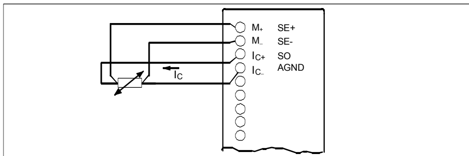
Рис. 5–14. Четырехпроводное присоединение термометров сопротивления к аналоговому входу
