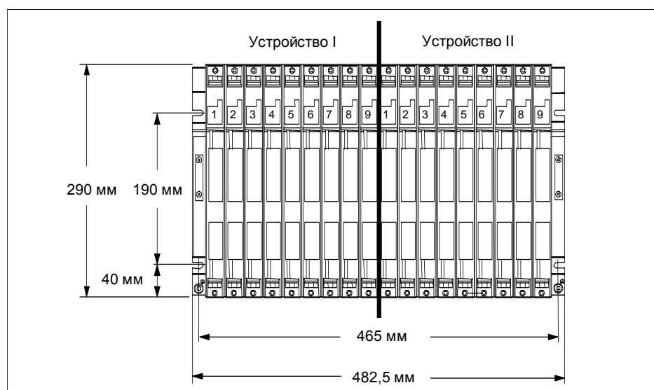
Рис. 2-3. Размеры стойки
