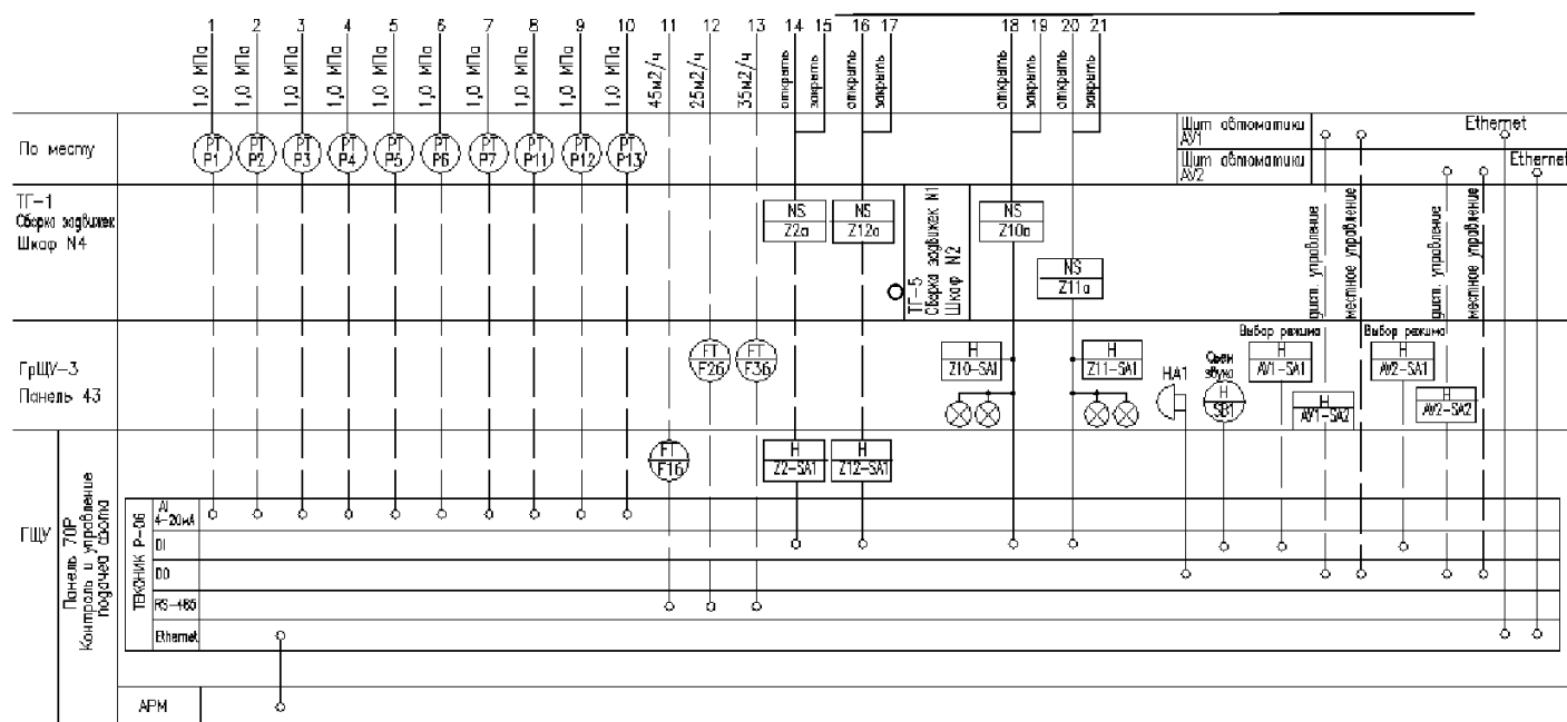
Рисунок В.36. Пример выполнения схемы АСУ ТП развернутым способом (начало схемы на рисунке В.3а)
