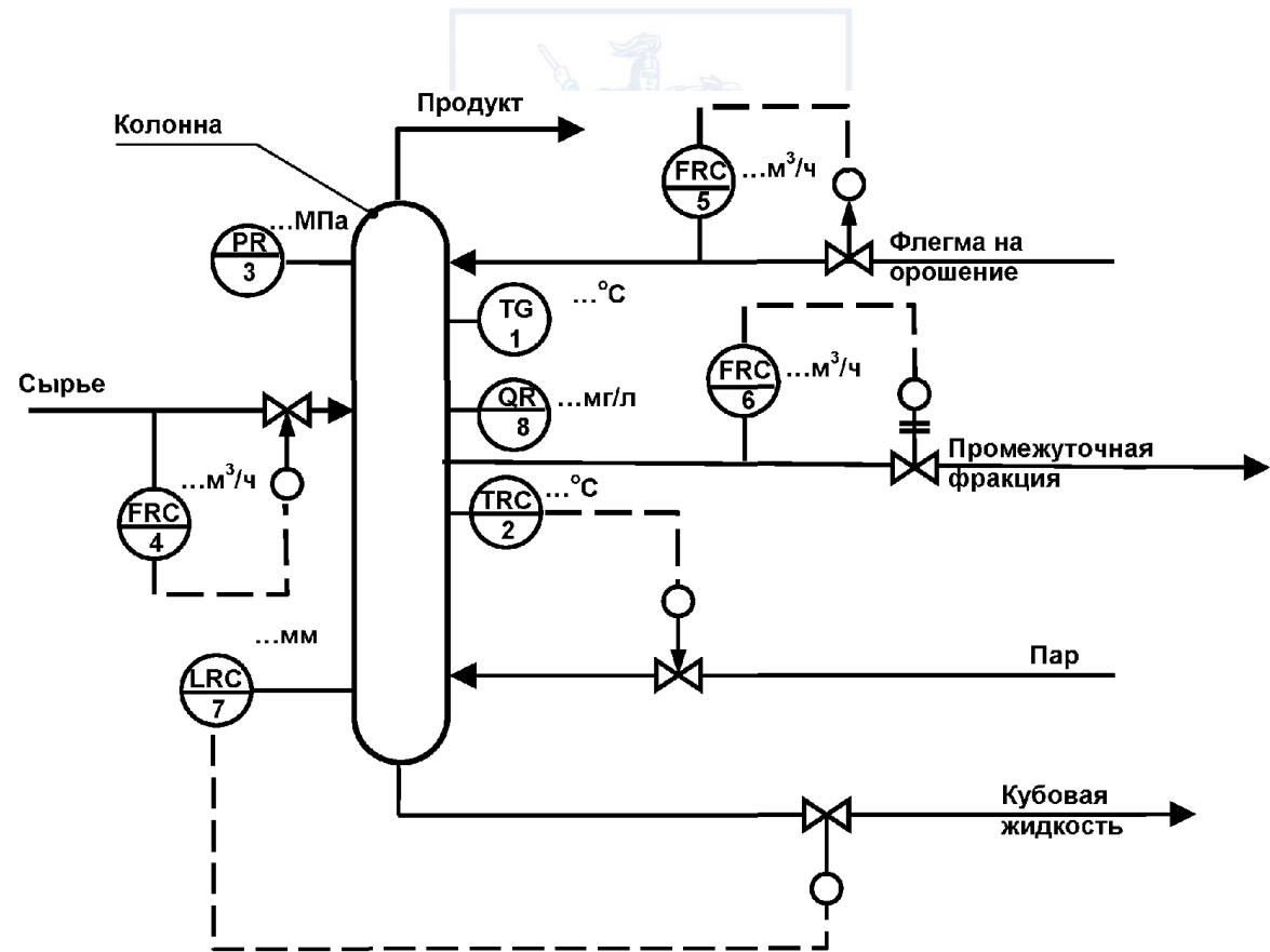
Рисунок В.1. Пример выполнения схемы автоматизации развернутым способом
