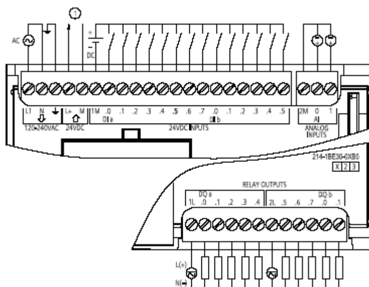
Рис. A-7. CPU 1214C AC/DC/Relay (6ES7 214-1BE30-0XB0)
