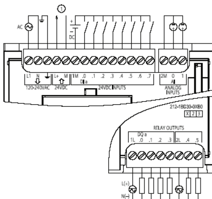
Рис. A-4. CPU 1212C AC/DC Relay (6ES7 212-1BD30-0XB0)
