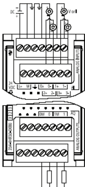
SM 1234 AI 4 x 13 Бит / AQ 2 x 14 бит
