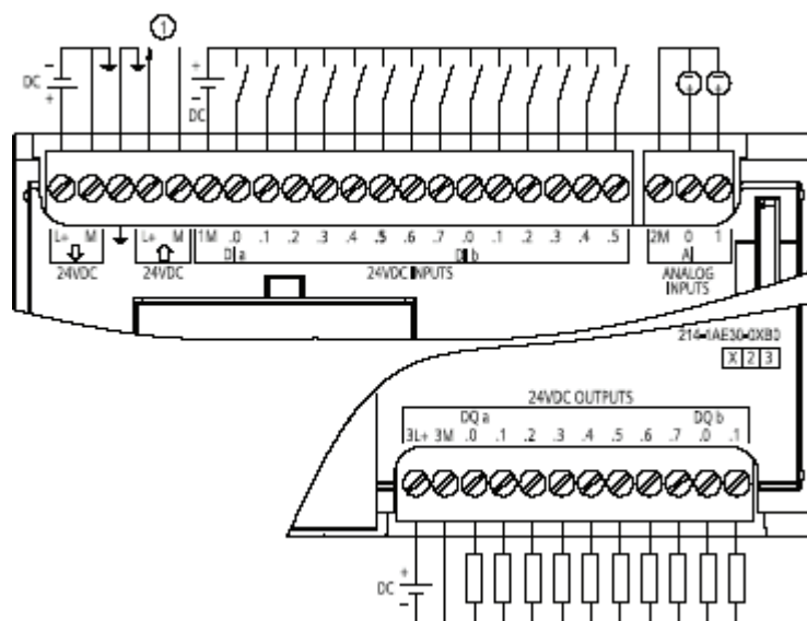
Рис. A-9. CPU 1214C DC/DC/DC (6ES7 214-1AE30-0XB0)
