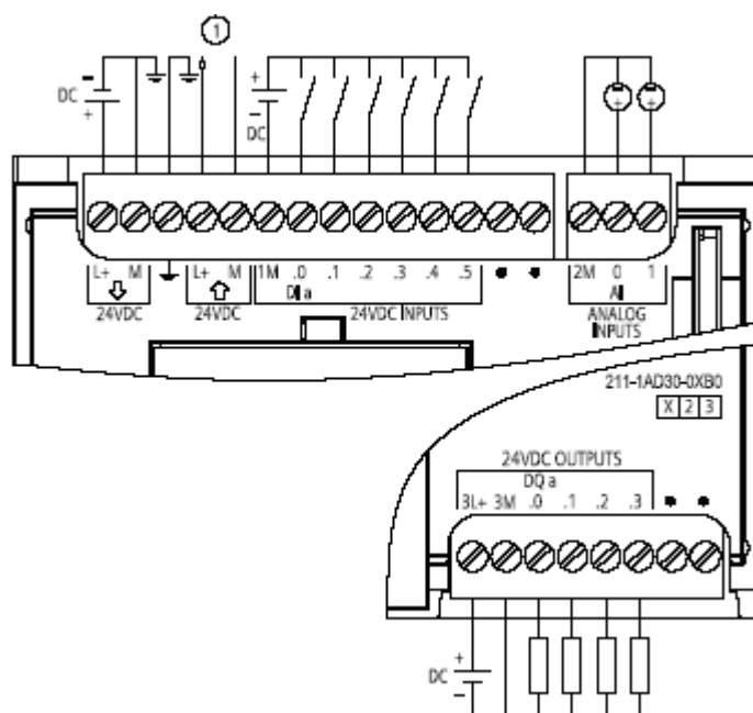
Рис. A-3. CPU 1211C DC/DC/DC (6ES7 211-1AD30-0XB0)
