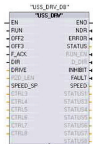
LAD (расширенное представление)
