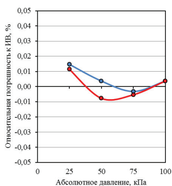
Рис. 2. Эталонный датчик абсолютного давления на 100 кПа и его относительная погрешность
