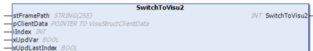
Рисунок 5.3.9.1 – Сигнатура метода SwitchToVisu2
