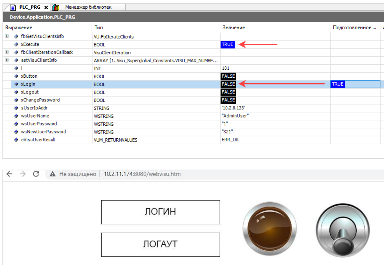
Рисунок 2.5.3 – Web-визуализация примера после авторизации пользователя AdminUser
