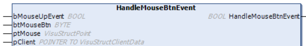
Рисунок 7.3.2.1 – Сигнатура метода HandleMouseBtnEvent
