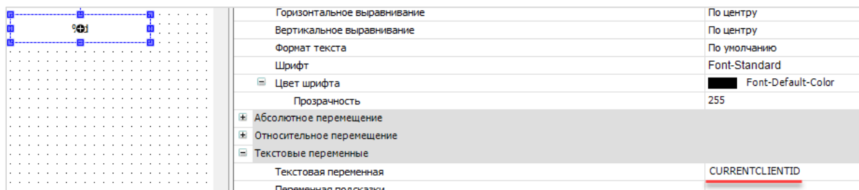
Рисунок 1.2.7.2 – Привязка системной переменной CURRENTCLIENTID к элементу визуализации
