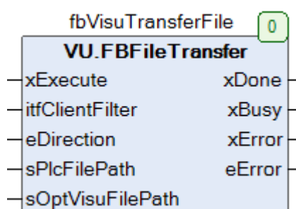
Рисунок 1.6.1 – Внешний вид ФБ FBFileTransfer на языке CFC
