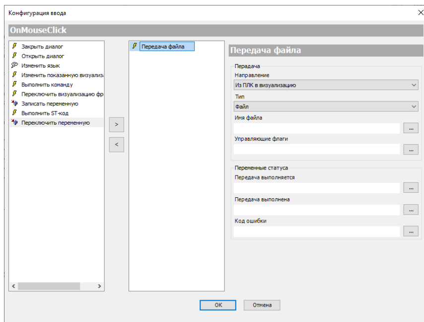
Рисунок 1.6.2 – Настройки действия Передача файла . ФБ FBFileTransfer является «программным» вариантом этого действия
