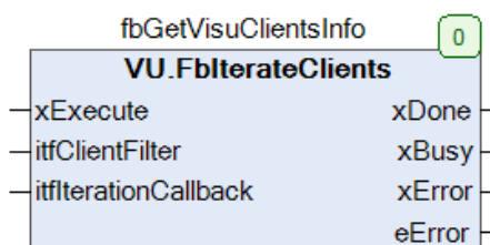
Рисунок 1.2.1 – Внешний вид ФБ FblterateClients на языке CFC
