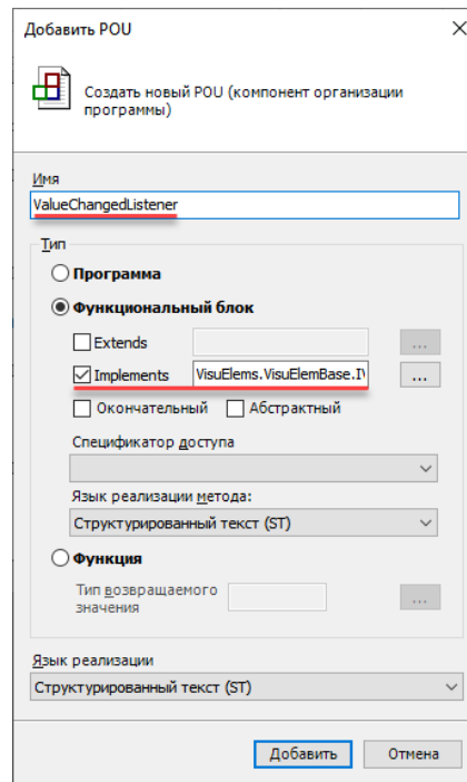
Рисунок 7.6.3.2 – Создание ФБ, реализующего интерфейс VisuElems.VisuElemBase.IValueChangedListener
