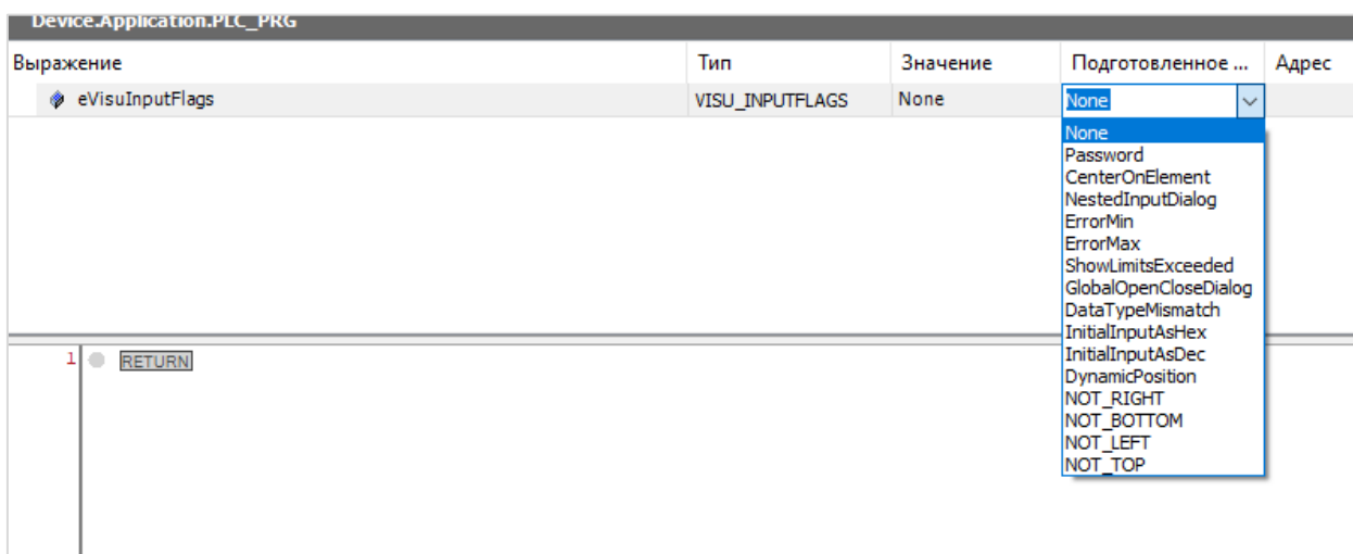
Рисунок 1.4.7.2 – Состав перечисления Visu_InputFlags
