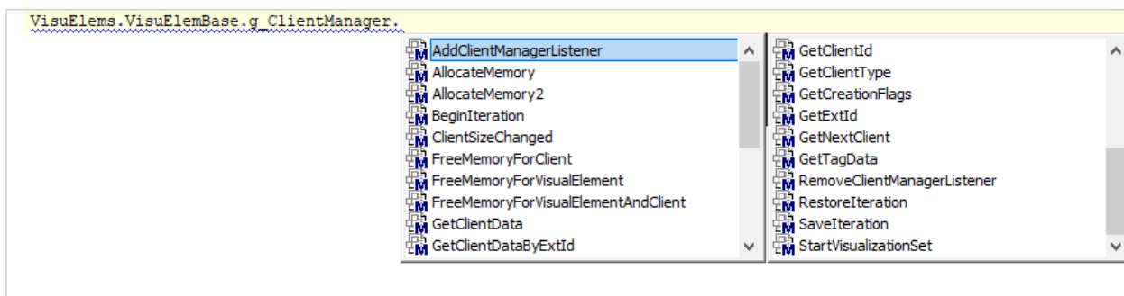
Рисунок 3.5.1 – Методы g_ClientManager
