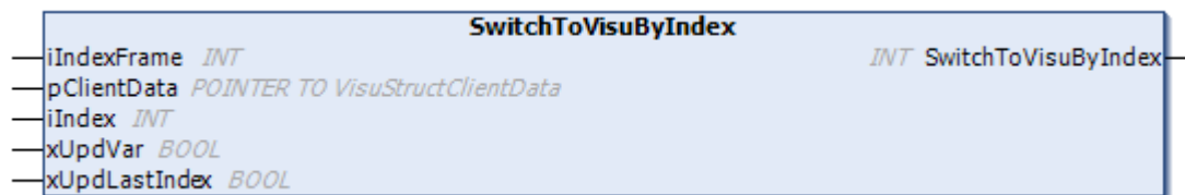
Рисунок 5.3.12.1 – Сигнатура метода SwitchToVisuByIndex
