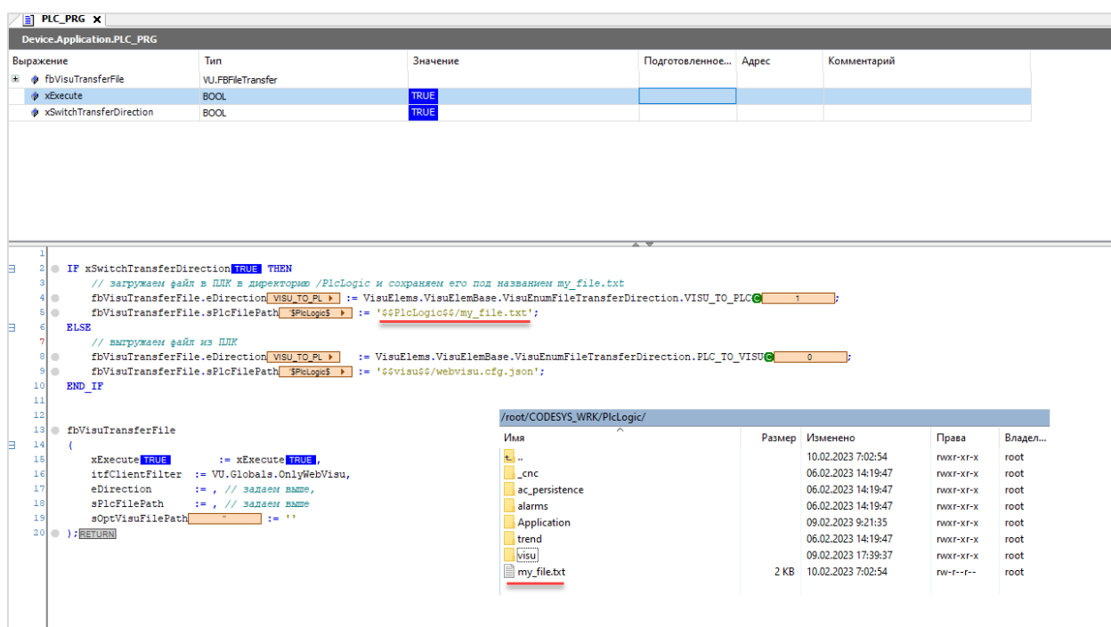
Рисунок 1.6.5 – Работа примера (для подключения к файловой системе контроллера использовалась утилита WinSCP )
