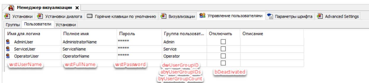
Рисунок 2.2.3 – Пояснения к полям структуры VUM_UserInternal
