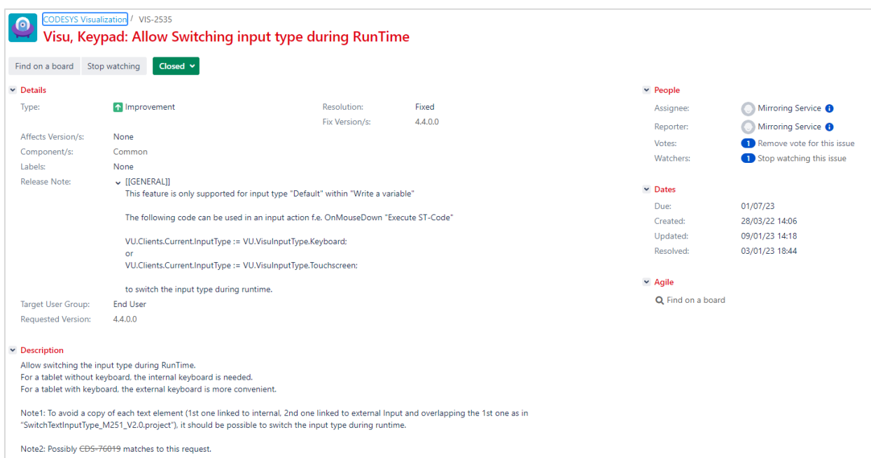
Рисунок 1.7.1 – Пожелание в баг-трекере CODESYS о добавлении в библиотеку Visu Utils возможности переключения типа ввода клиента визуализации
