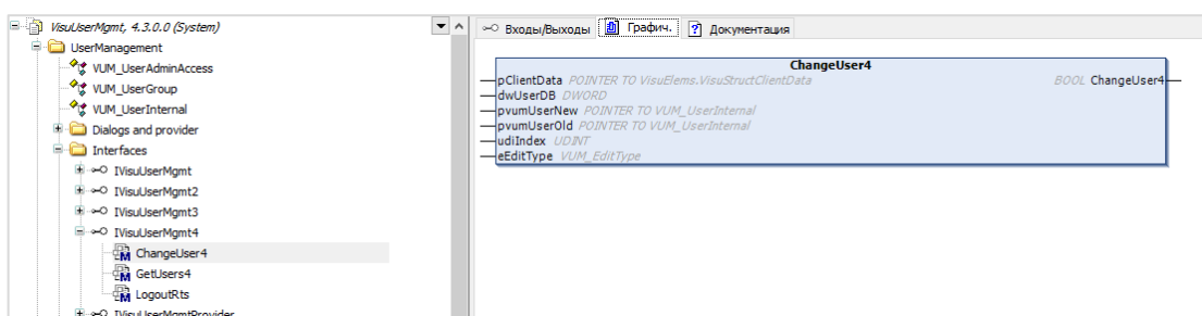
Рисунок 2.7.1 – Сигнатура метода ChangeUser4
