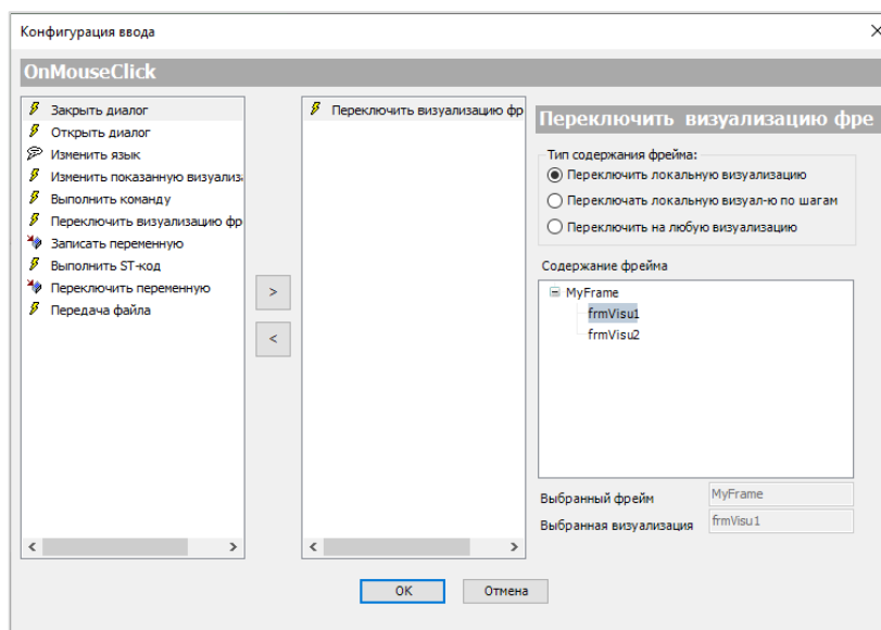
Рисунок 5.2.2 – Настройки для типа содержания «Переключить локальную визуализацию»
