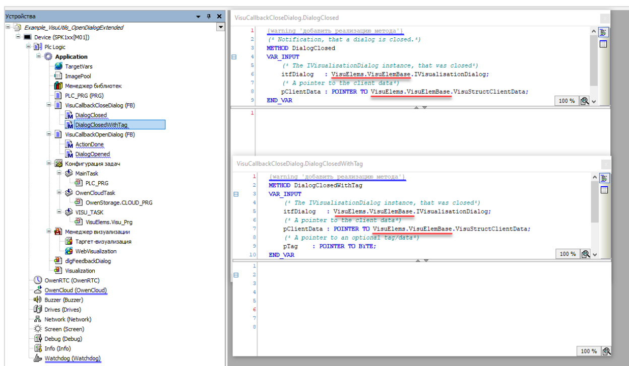
Рисунок 1.4.4.1 – Методы, полученные от интерфейса IDialogCloseListenerWithTag
