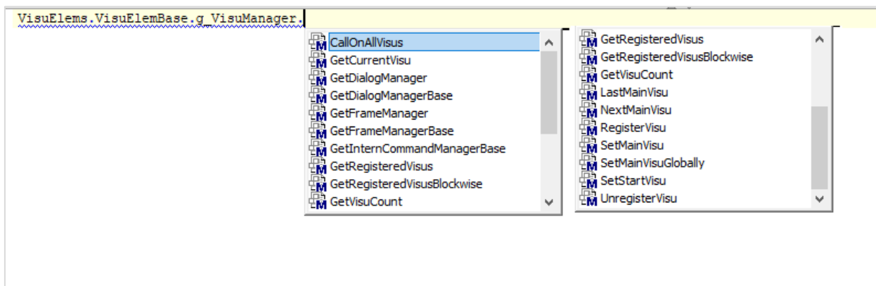
Рисунок 3.4.1 – Методы g_VisuManager
