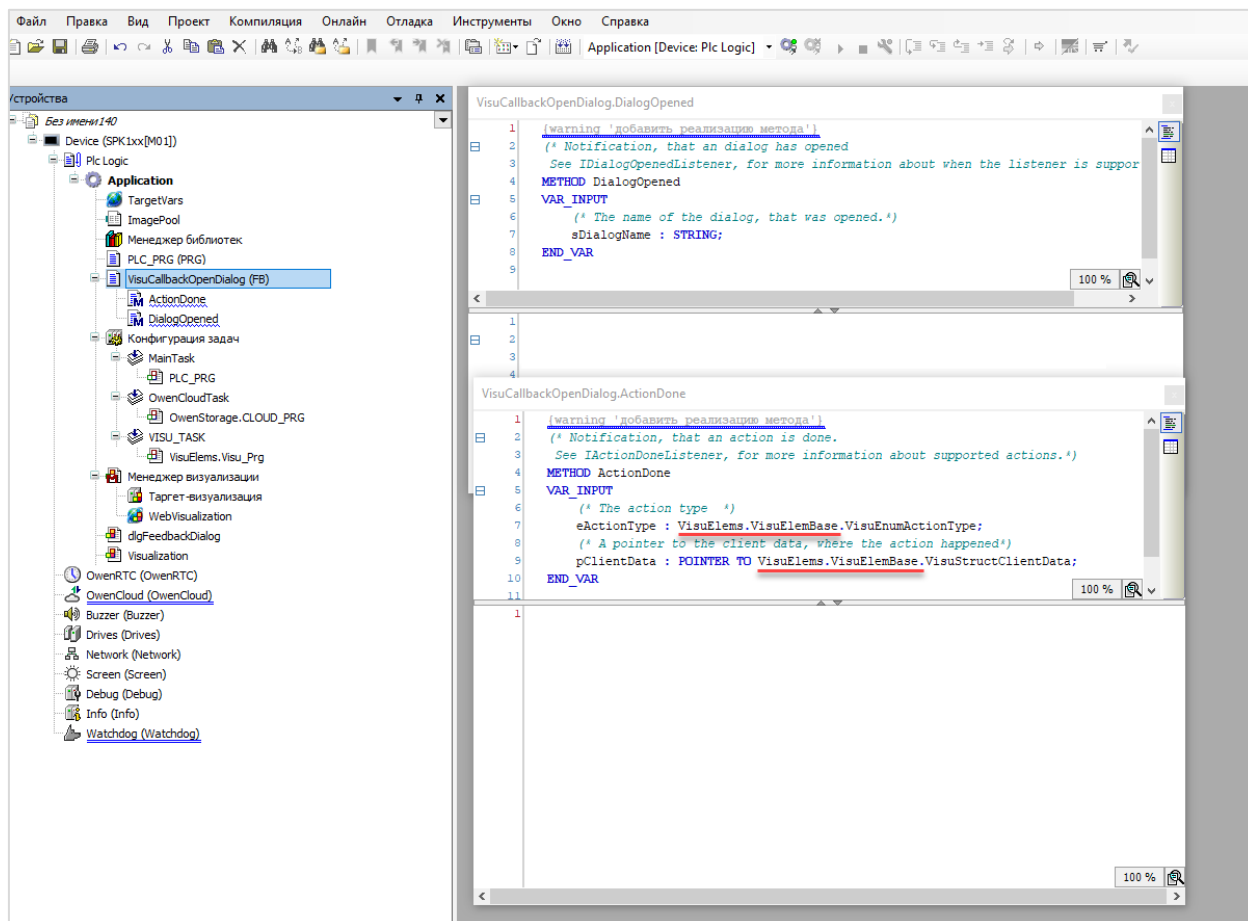
Рисунок 1.4.3.1 – Методы, полученные от интерфейса itfDialogOpenedListener
