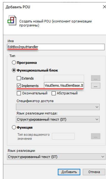
Рисунок 7.5.3.2 – Создание ФБ, реализующего интерфейс VisuElems.VisuElemBase.IEditBoxInputHandler
